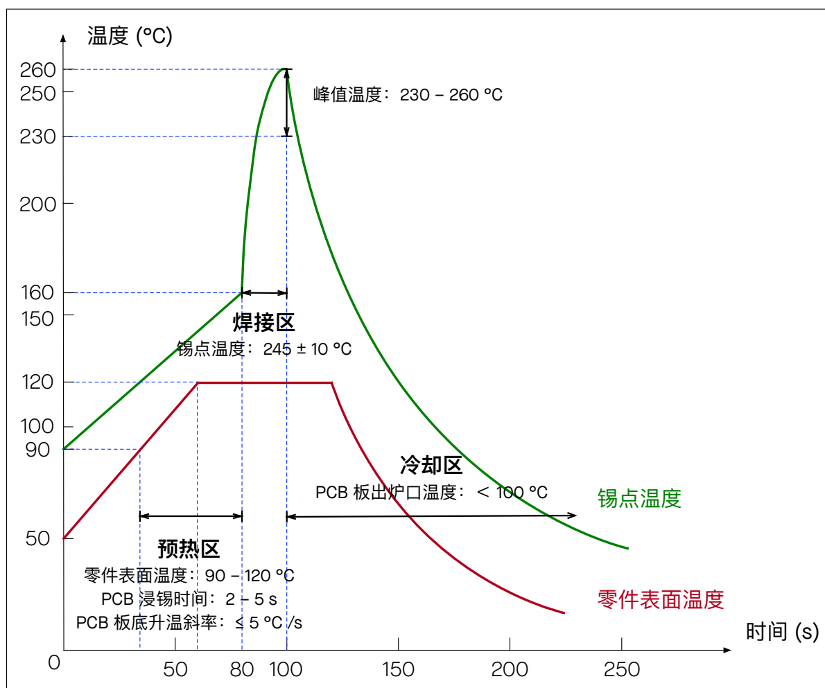
图 12-1. 波峰焊温度曲线
