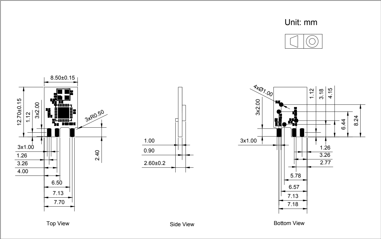
图 10-1. 模组尺寸
