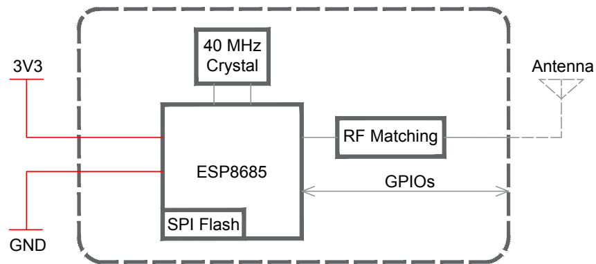
图 2-1. 功能框图
