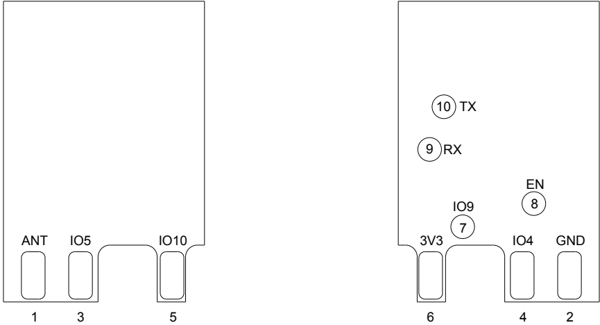
图 3-1. 管脚布局
