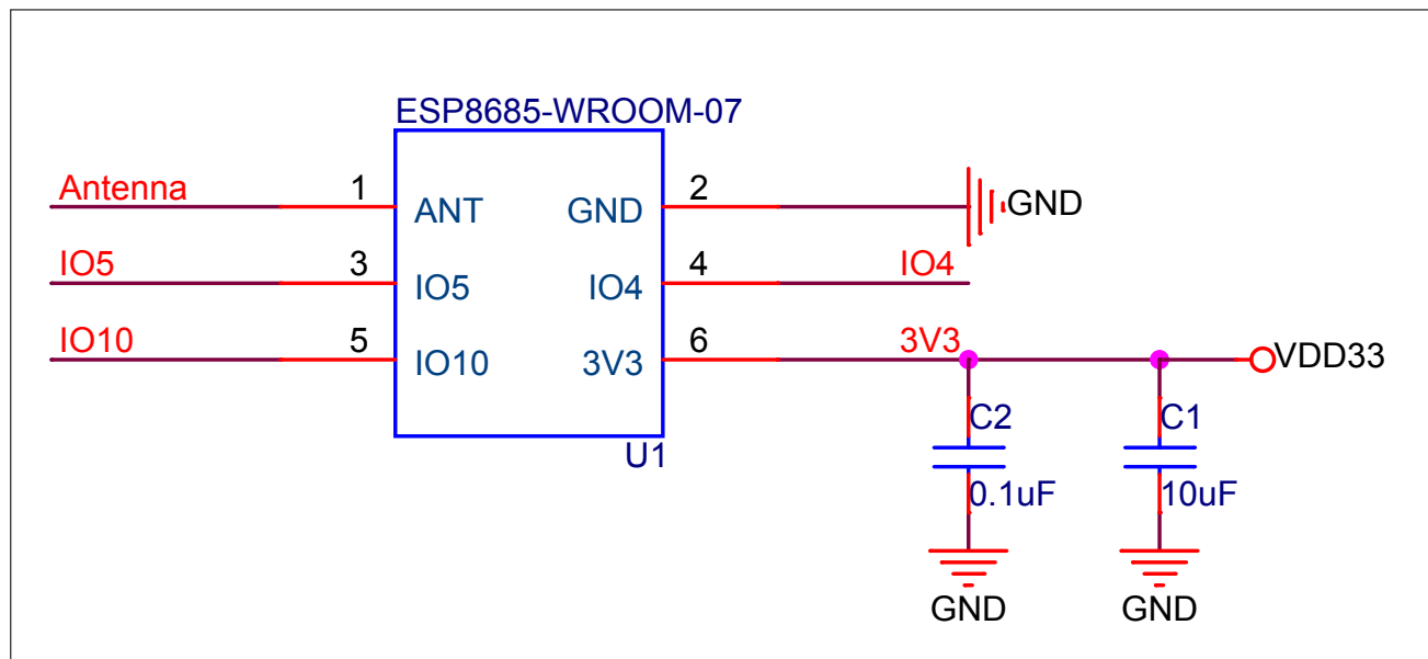
图 9-1. 外围设计原理图
