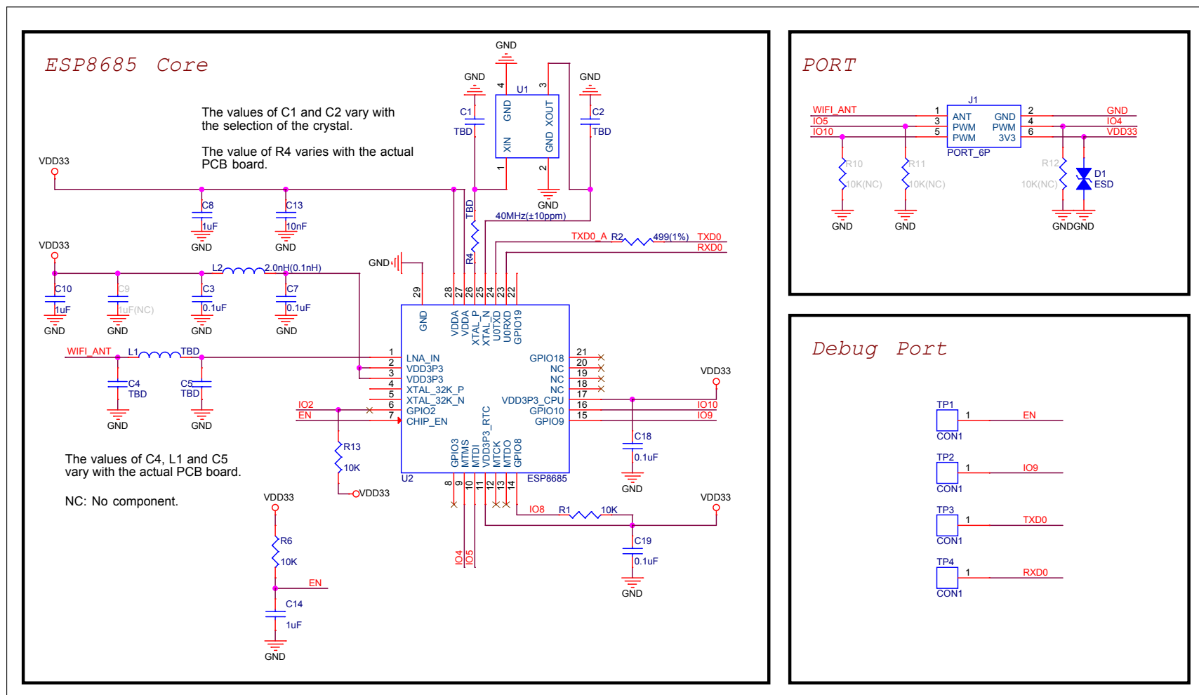
图 8-1. 原理图
