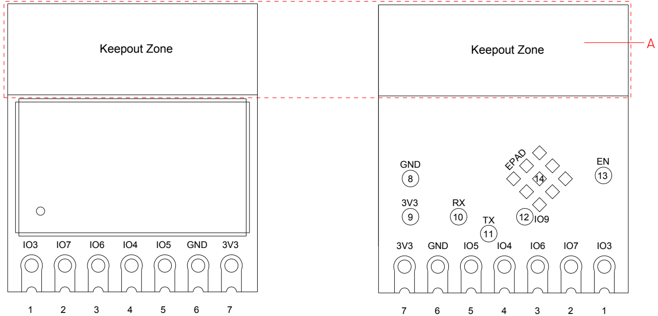
图 3-1. 管脚布局（顶视图和底视图）
