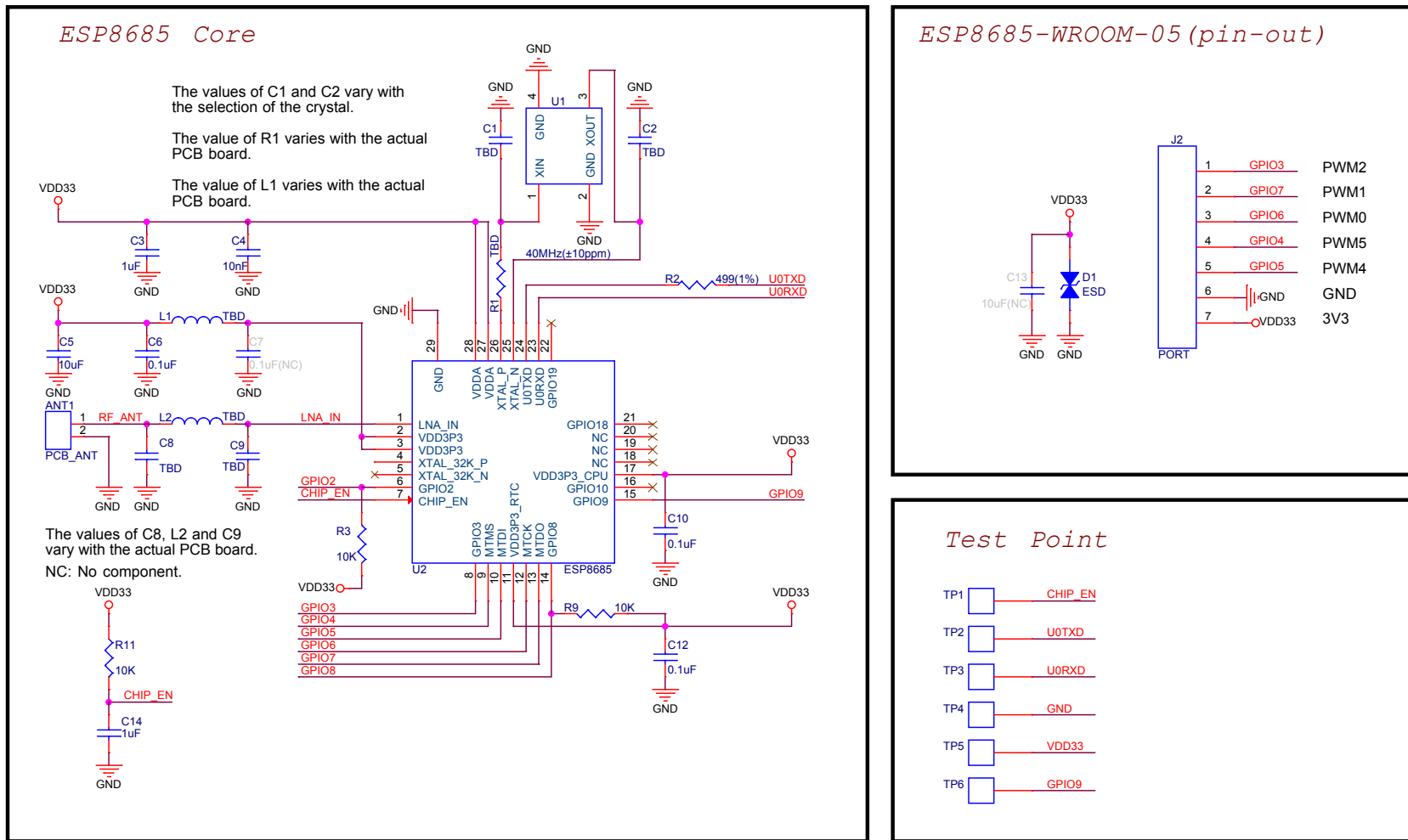
图 8-1. 原理图
