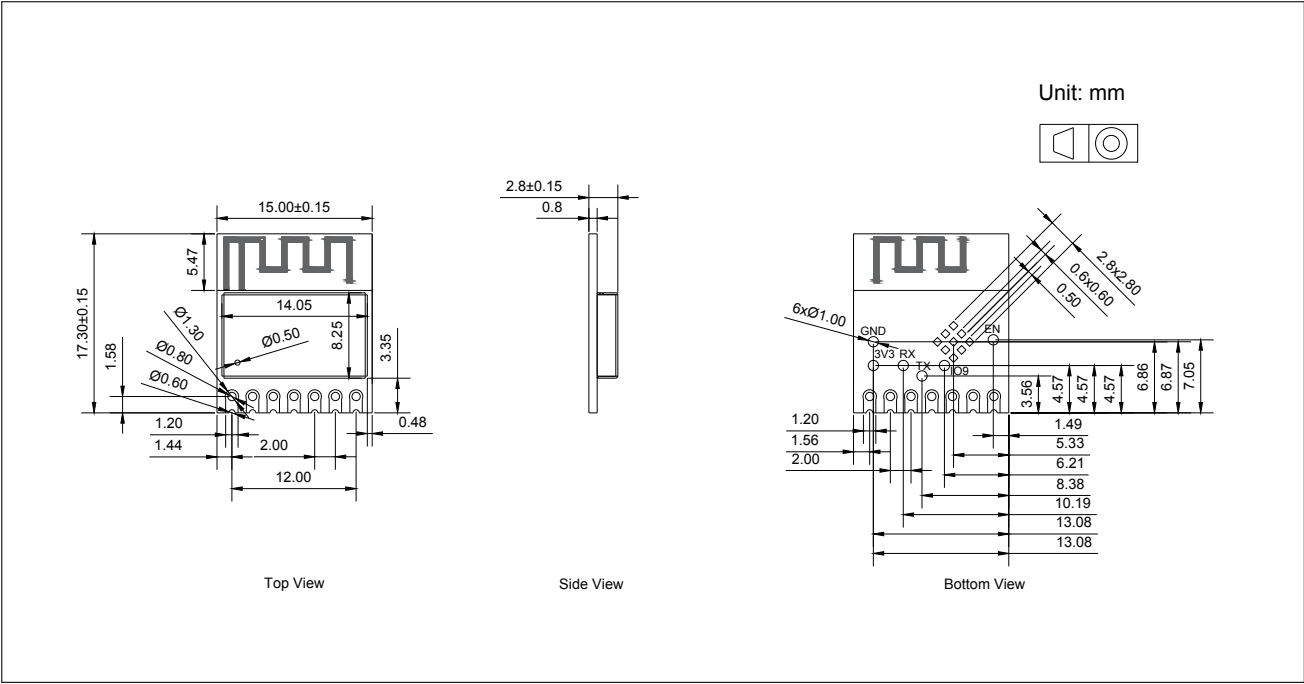
图 10-1. 模组尺寸
