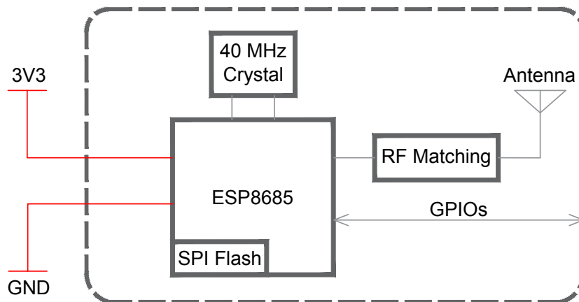
图 2-1. 功能框图
