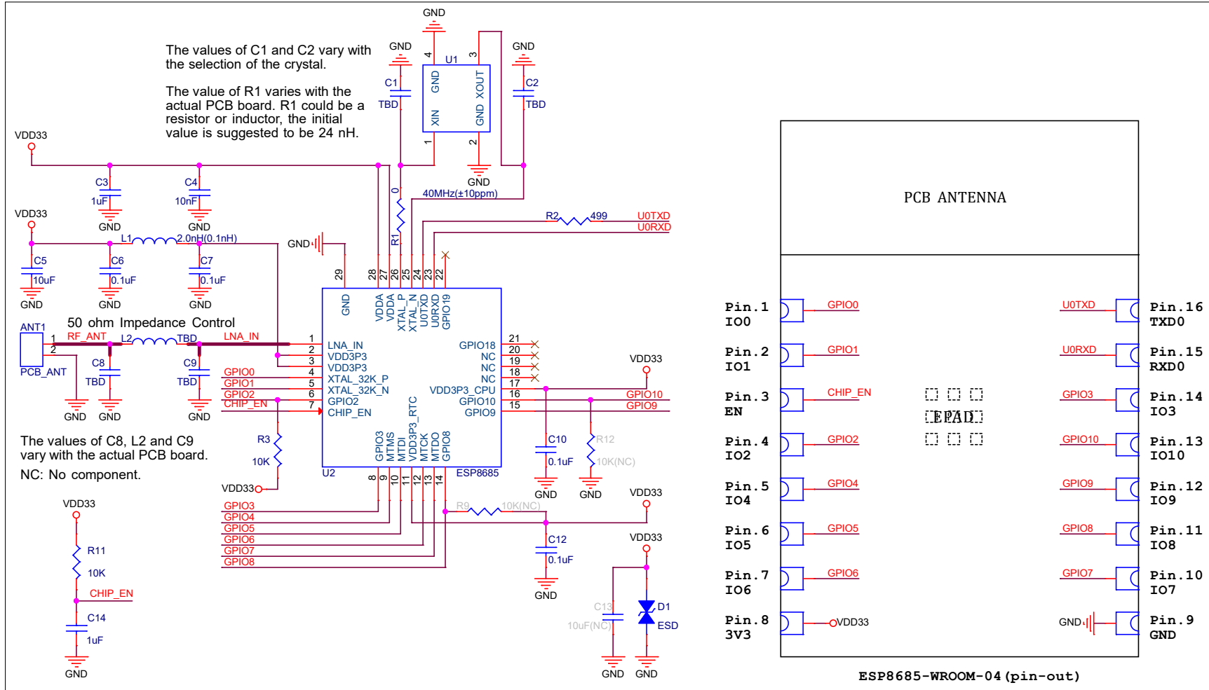
图 8-1. 原理图
