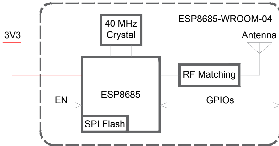
图 2-1. 功能框图
