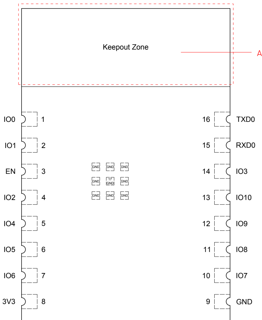
图 3-1. 管脚布局（顶视图）
