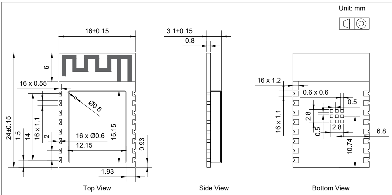
图 10-1. 模组尺寸
