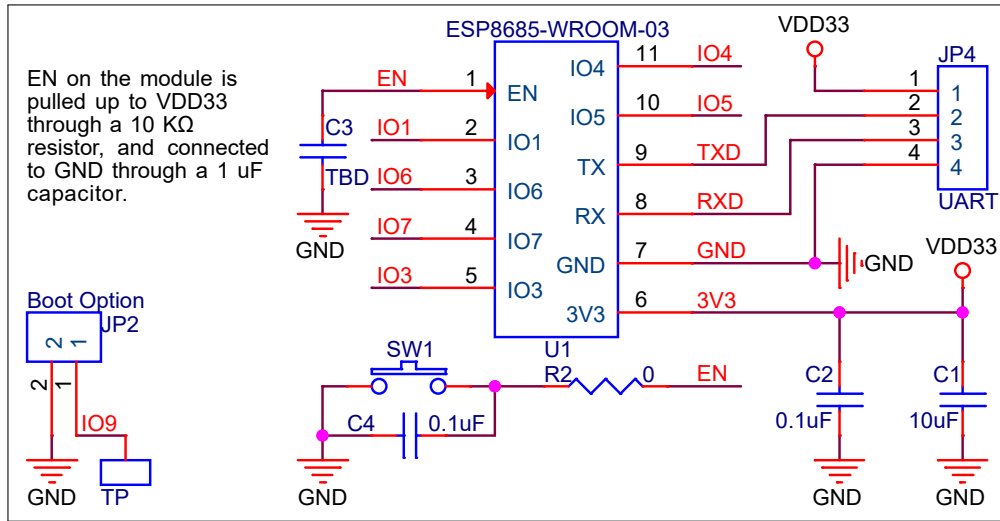
图 9-1. 外围设计原理图
