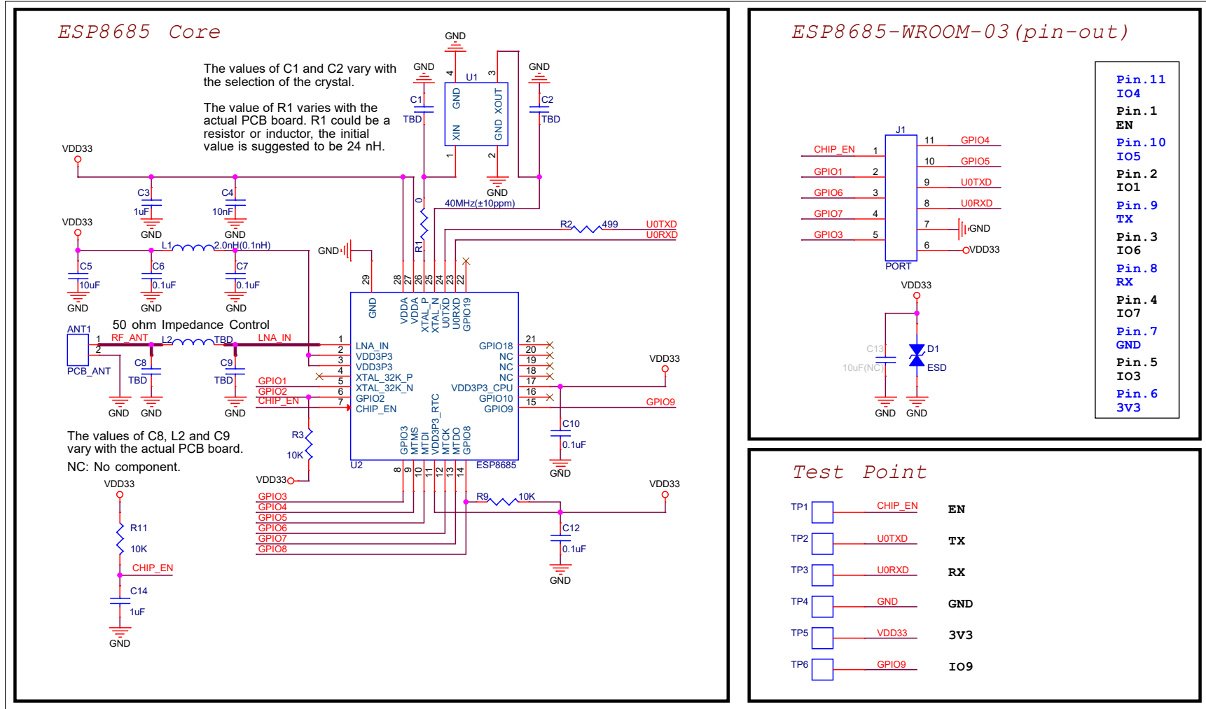
图 8-1. 原理图
