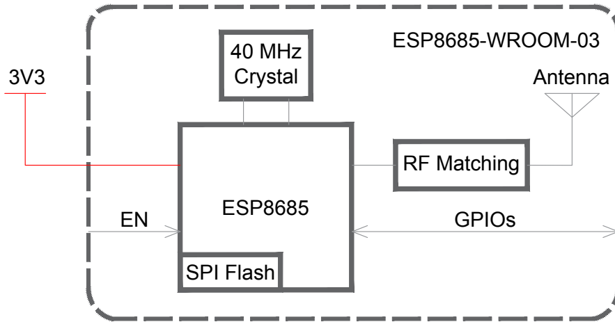
图 2-1. 功能框图
