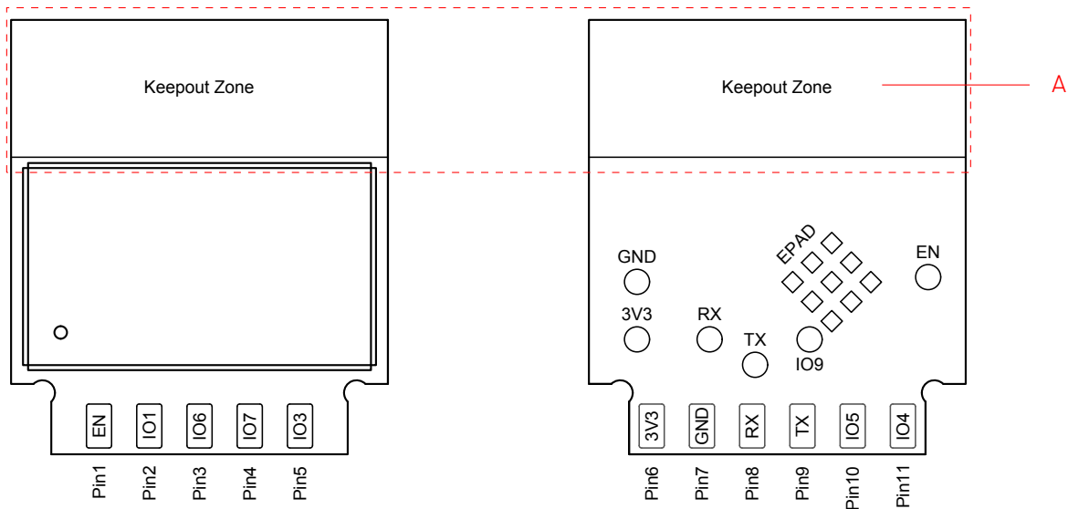
图 3-1. 管脚布局（顶视图和底视图）
