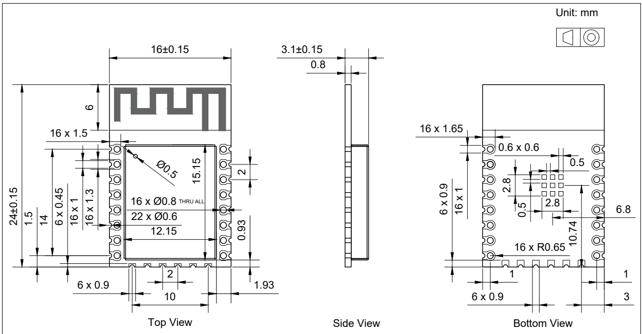
图 10-1. 模组尺寸
