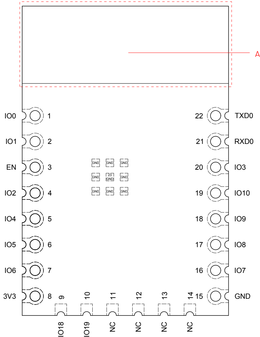
图 3-1. 管脚布局（顶视图）
