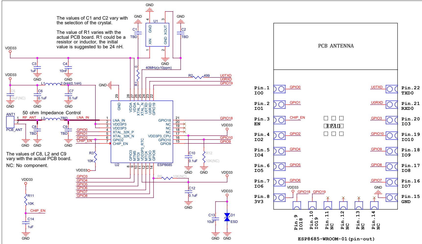
图 8-1. 原理图
