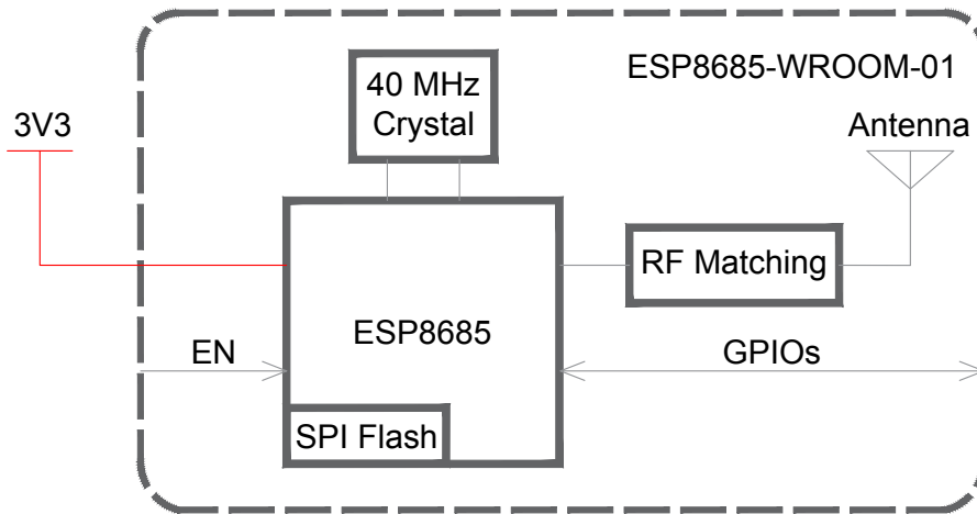
图 2-1. 功能框图
