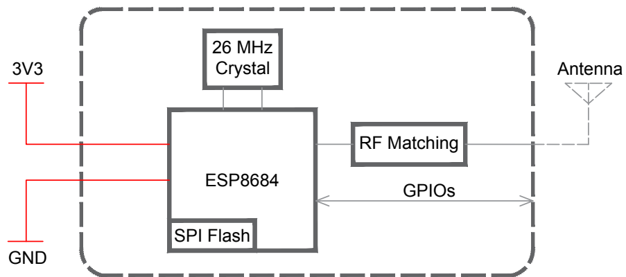
图 1: ESP8684-WROOM-07 功能框图
