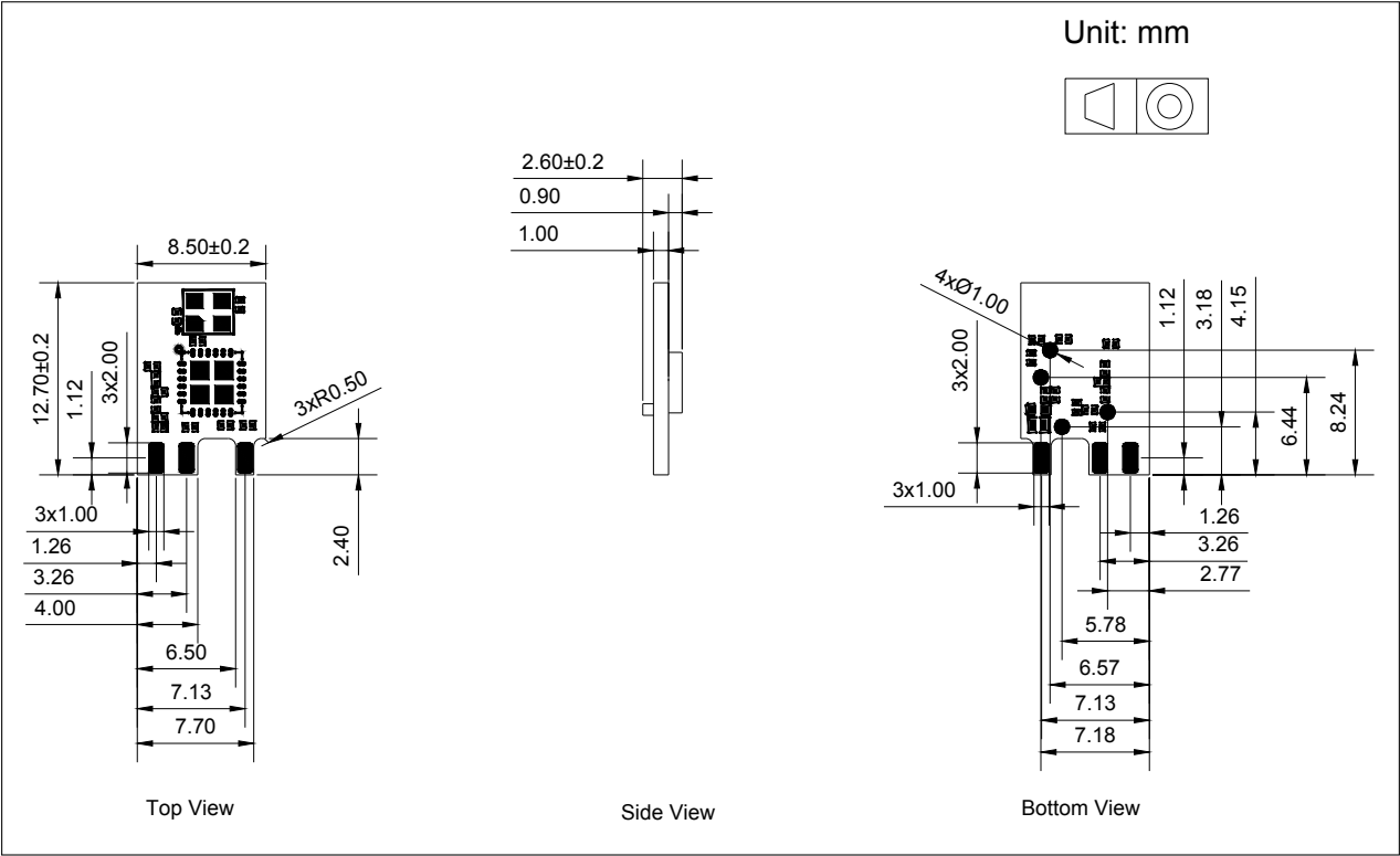
图 6: 模组尺寸
