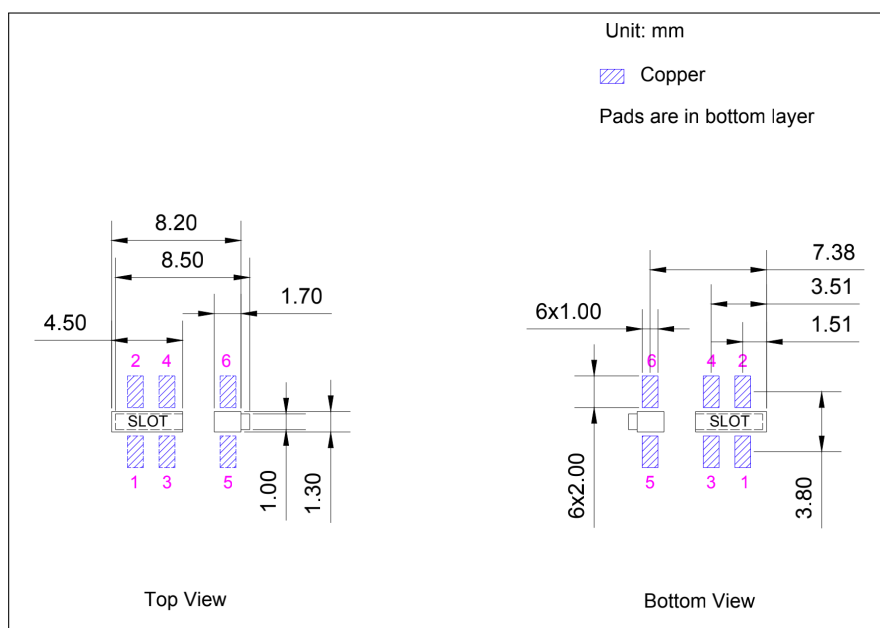
图 7: 推荐 PCB 封装图形
