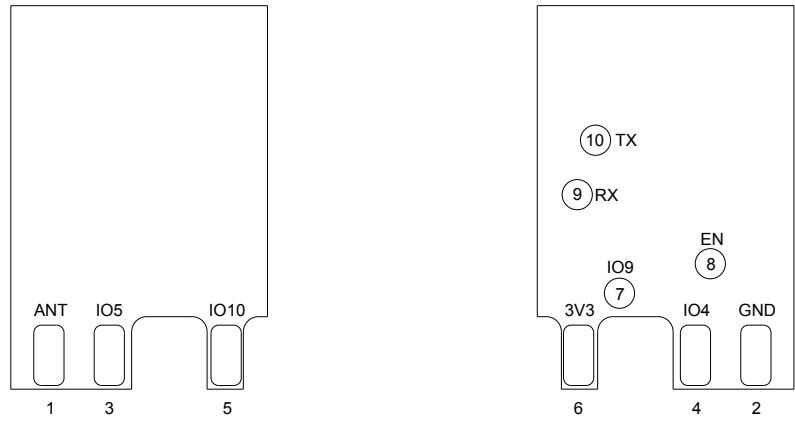
图 2: 管脚布局（顶视图和底视图）
