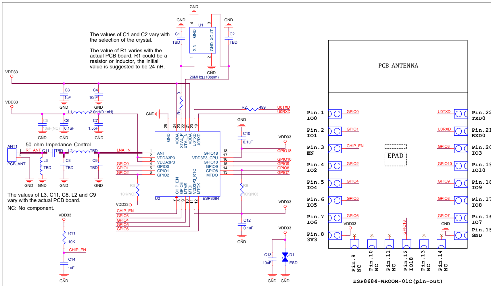
图 4: ESP8684-WROOM-01C 原理图
