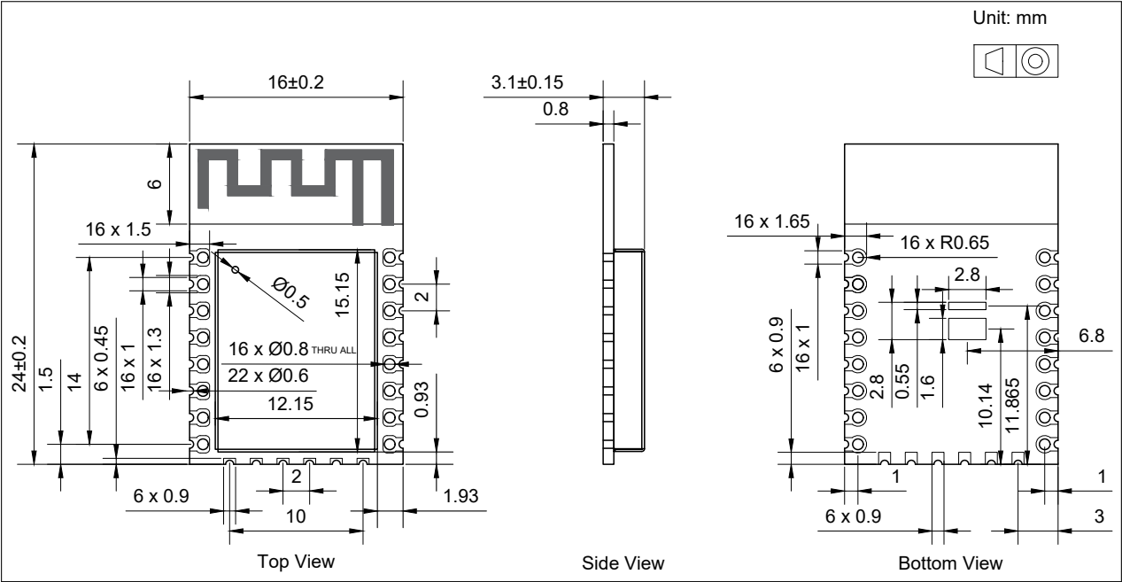
图 6: 模组尺寸
