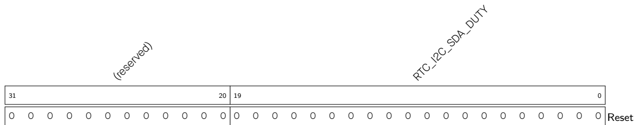
Register 1.16. RTC_I2C_SDA_DUTY_REG (0x030)
