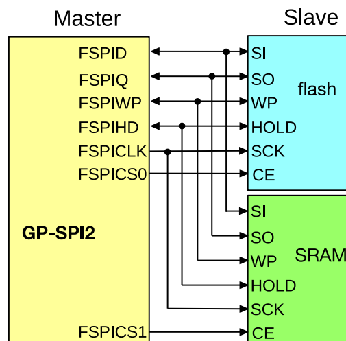
图 24.4-3. 4-bit 模式下 GP-SPI2 连接 Flash 和外部 RAM
