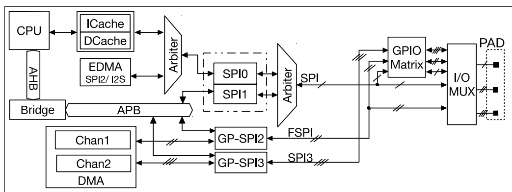
图 24.1-1. SPI 框图
