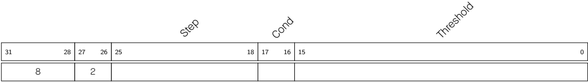
图 1.5-13. 指令类型 - JUMPS
