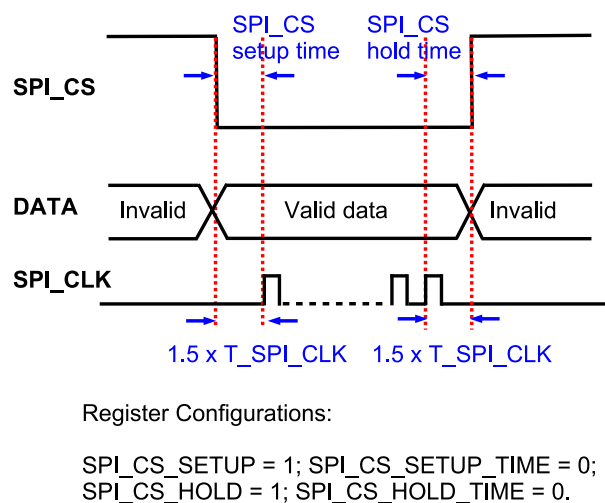
图 24.4-11. GP-SPI2 访问外部 Flash 时推荐的 CS 时序配置
