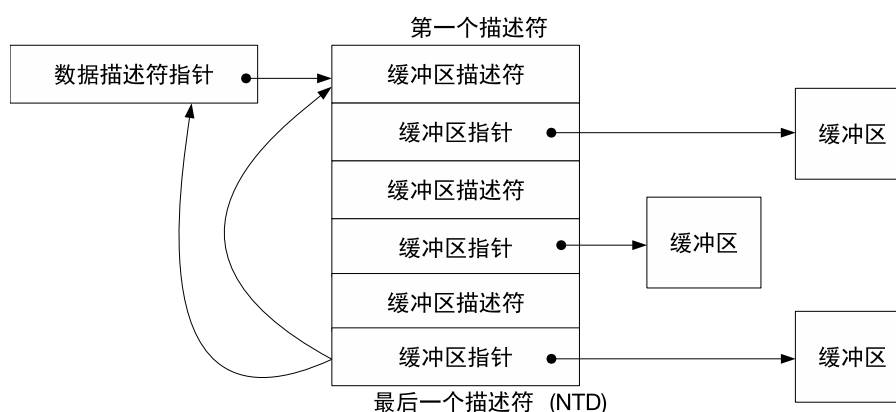
图 28.3-6. Scatter/Gather DMA 链表结构
