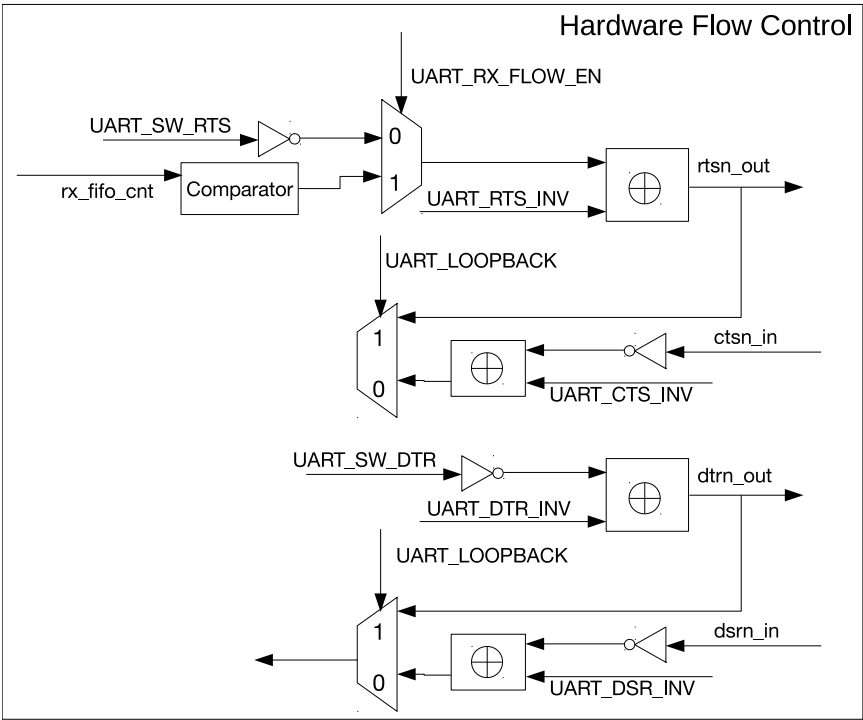
图 23.3-10. 硬件流控图
