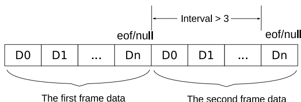
图 2.3-4. EDMA 访问片内 RAM 时的数据帧示意图
