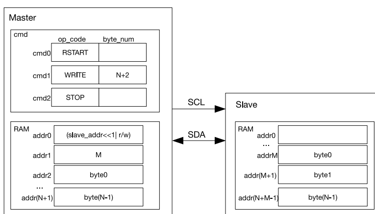
图 25.3-3. I2C Master 写 7-bit 寻址 Slave 的 M 地址 RAM
