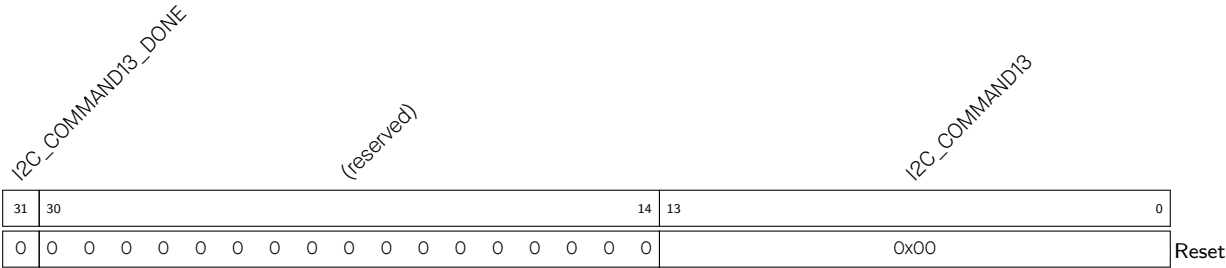
Register 25.39. I2C_COMD13_REG (0x008C)
