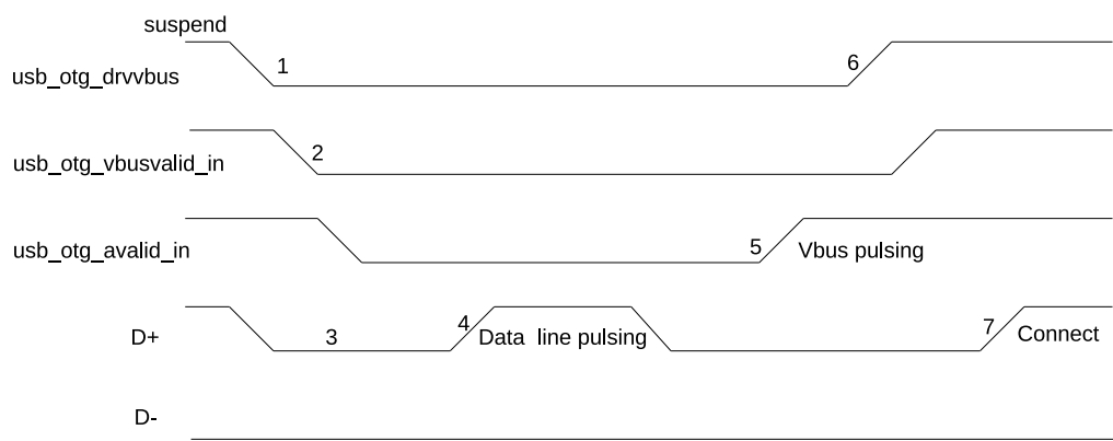
图 28.4-1. A 设备 SRP
