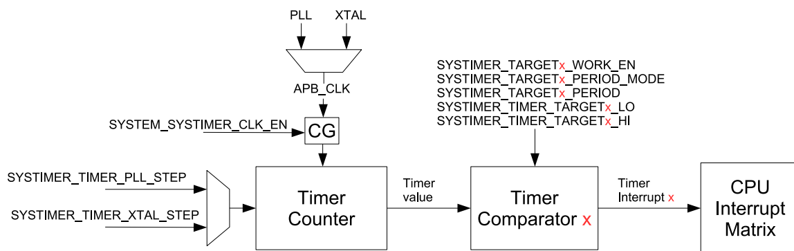
图 10.4-1. 系统定时器结构
