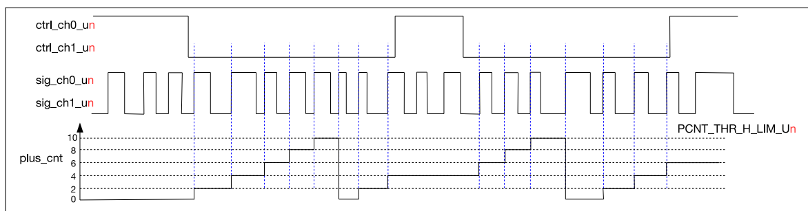
图 27.3-3. 双通道递增计数图
