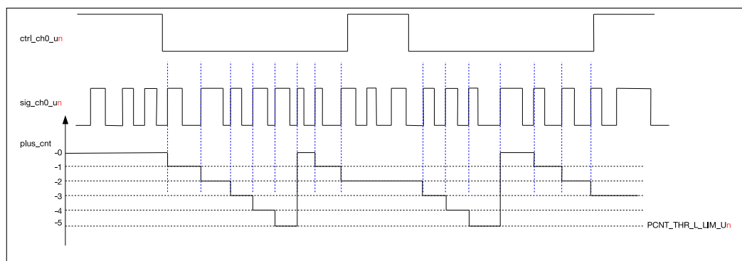
图 27.3-2. 通道 0 递减计数图
