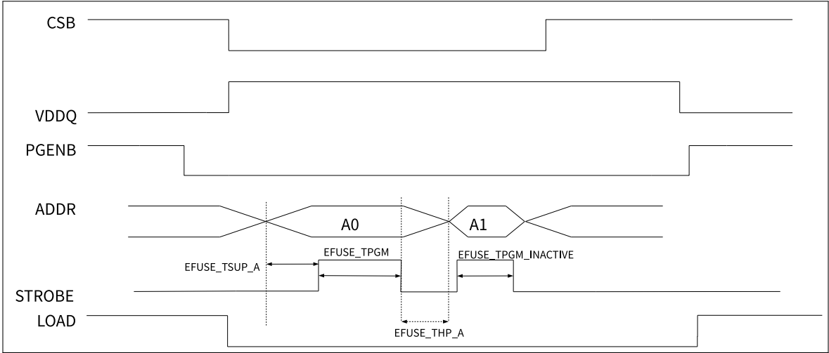
图 4.3-3. eFuse 烧写时序图
