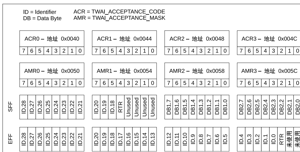
图 29.4-2. 单滤波模式
