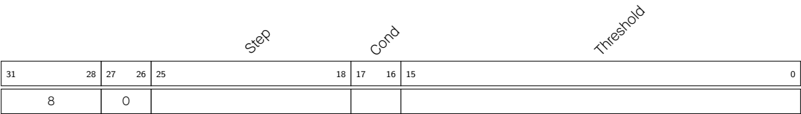
图 1.5-12. 指令类型 - JUMPR
