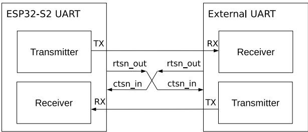
图 23.3-11. 硬件流控信号连接图
