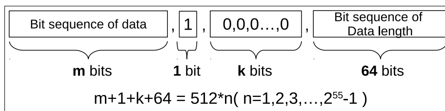
图 19.4-1. HMAC 附加填充位示意图
