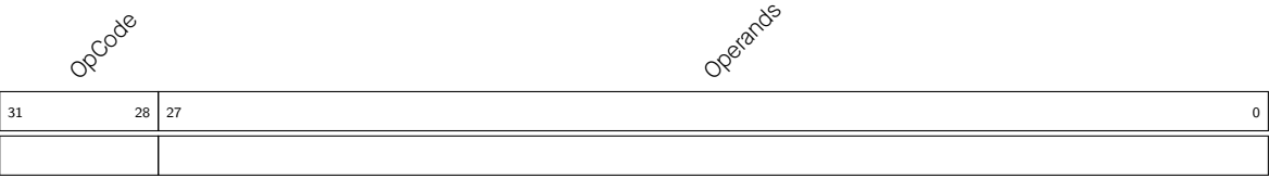
图 1.5-1. ULP-FSM 协处理器的指令格式
