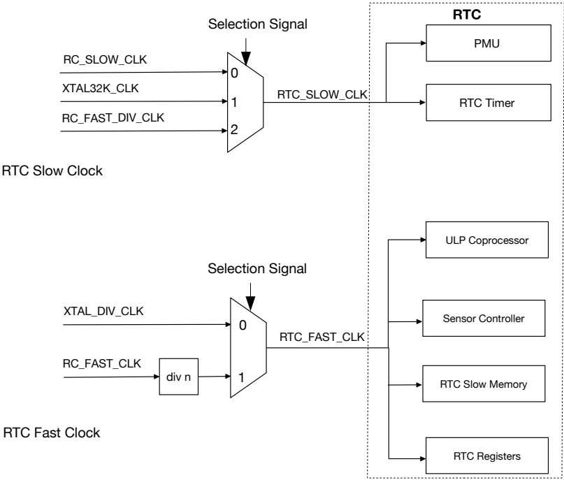
图 9.3-3. RTC 电源域的快速时钟和慢速时钟
