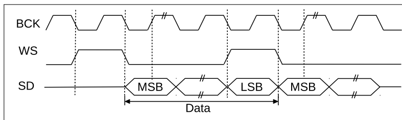
图 26.4-3. PCM 标准
