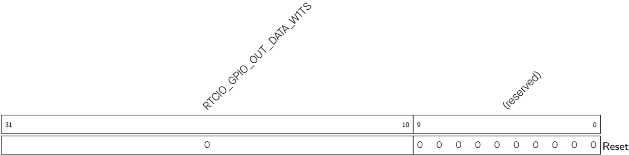
Register 5.53. RTCIO_RTC_GPIO_OUT_W1TS_REG (0x0004)
