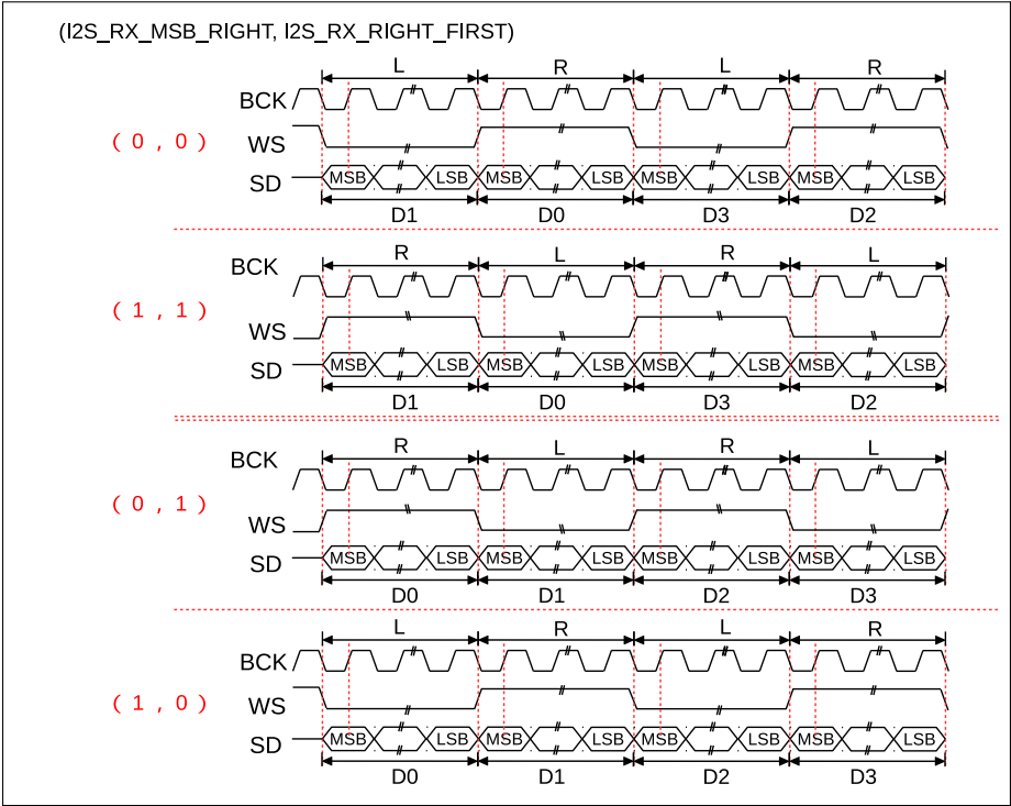
图 26.9-2. I2S_RX_DMA_EQUAL = 0 时，ESP32-S2 I2S 接收数据的控制图
