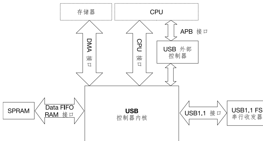
图 28.3-1. OTG_FS 系统架构
