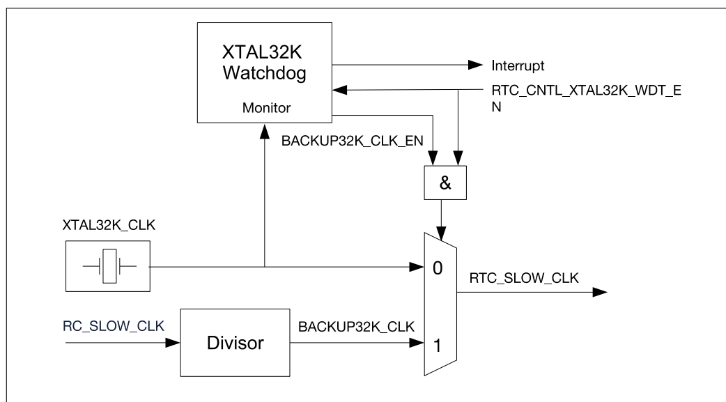
图 13.1-1. XTAL32K 看门狗定时器
