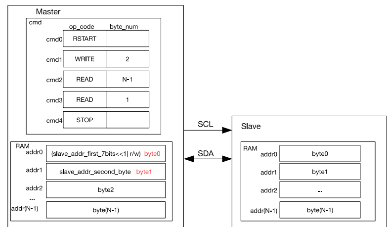
图 25.3-6. I2C Master 读 10-bit 寻址的 Slave
