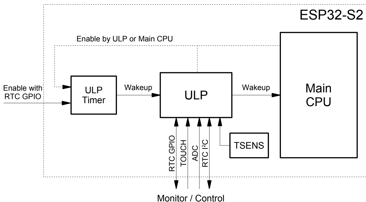
图 1.1-1. 超低功耗协处理器概图
