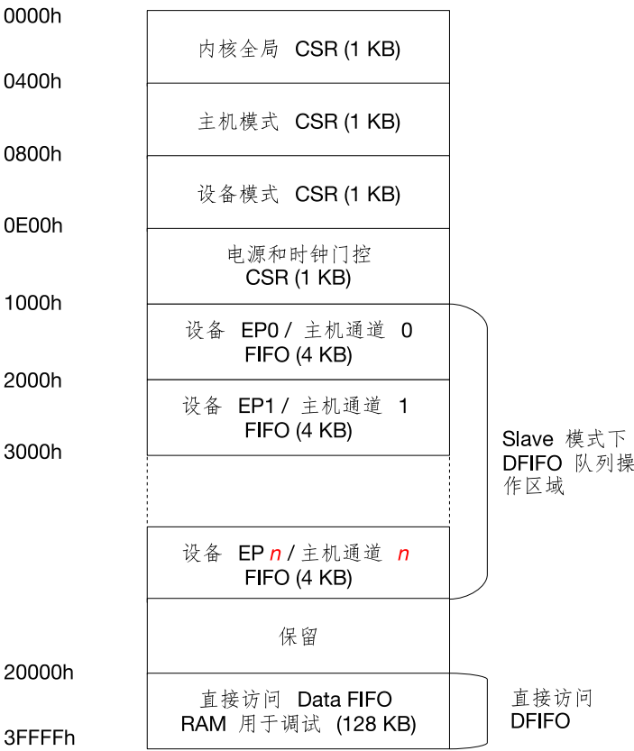
图 28.3-2. 内核地址映射
