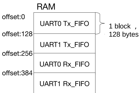
图 23.3-2. UART 共享 RAM 图
