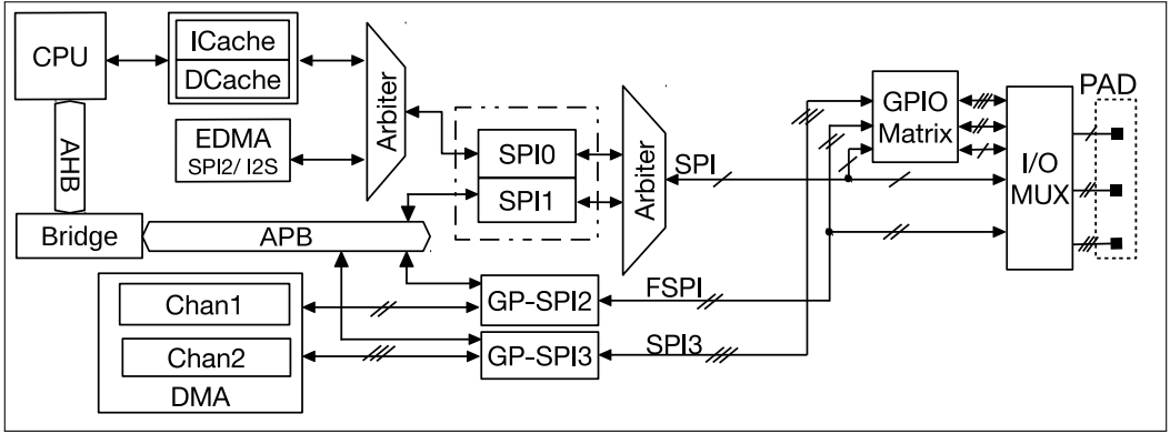
图 24.3-1. GP-SPI2/GP-SPI3 控制器框图
