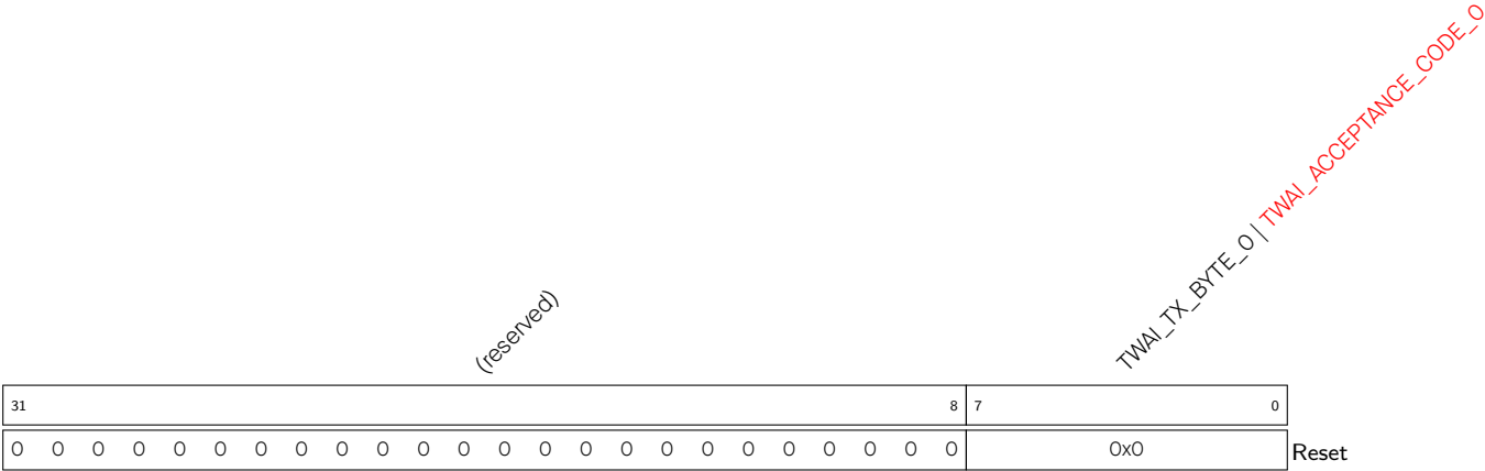
Register 29.5. TWAI_DATA_0_REG (0x0040)
