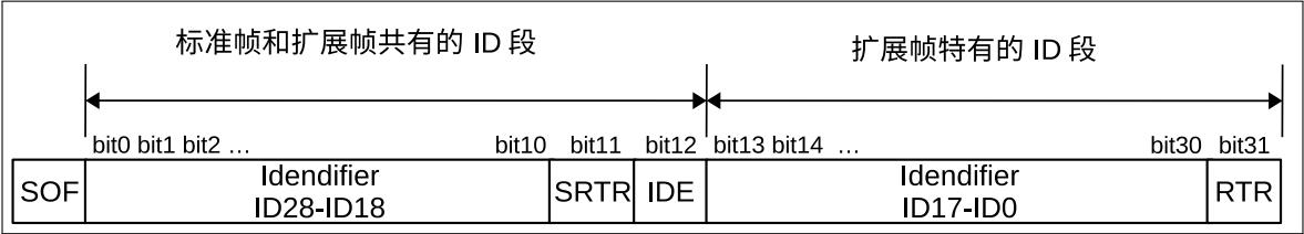
图 29.4-5. 丢失仲裁的 bit 位置
