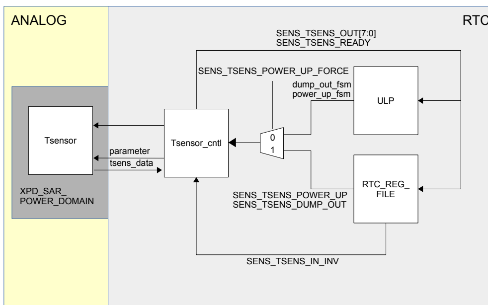
图 32.4-1. 温度传感器结构
