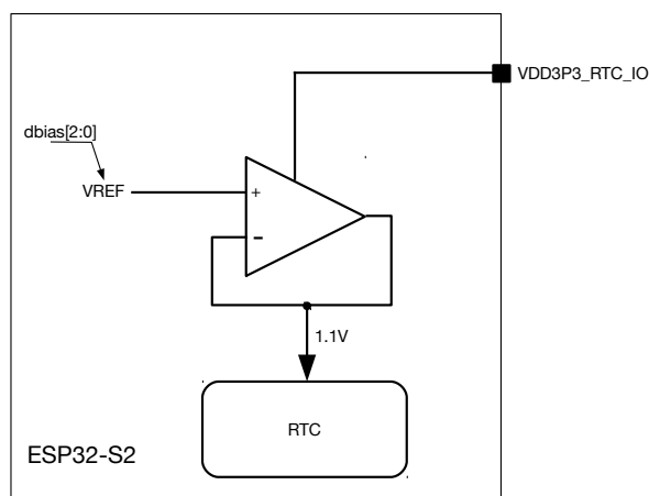
图 9.3-6. 低功耗调压器
