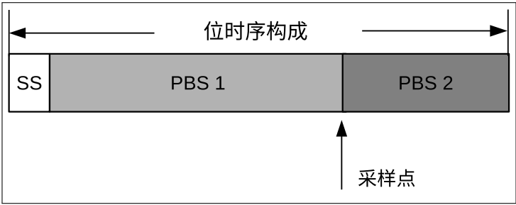
图 29.2-5. 位时序构成
