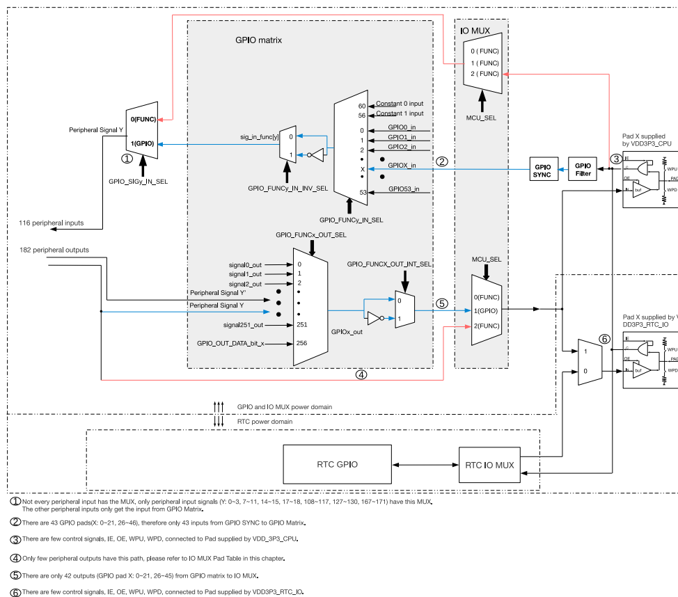
图 5.1-1. IO MUX、RTC IO MUX 和 GPIO 交换矩阵结构框图
