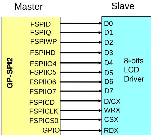
图 24.4-5. GP-SPI2 与 8-bit LCD 驱动的连接方式
