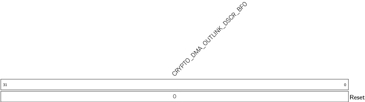
Register 2.41. CRYPTO_DMA_OUT_DSCR_BFO_REG (0x005C)
