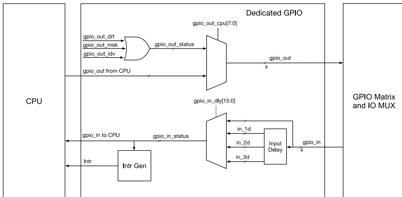
图 5.4-1. 专用 GPIO 模块图
