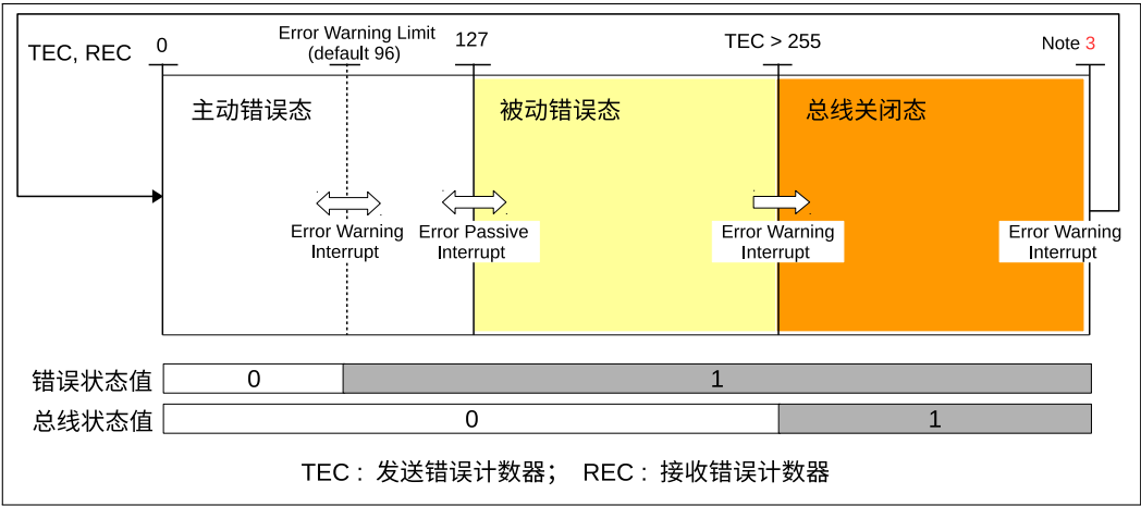
图 29.4-4. 错误状态变化
