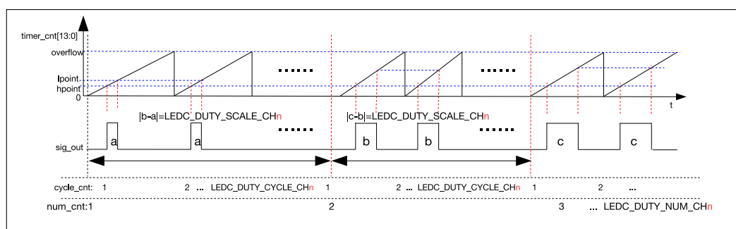
图 30.3-5. 渐变占空比输出信号图
