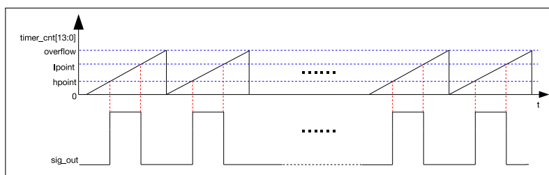
图 30.3-4. LED_PWM 输出信号图
