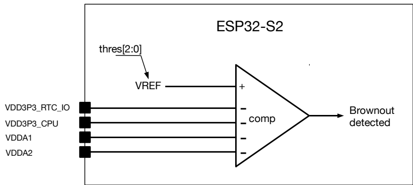
图 9.3-8. 欠压检测器
