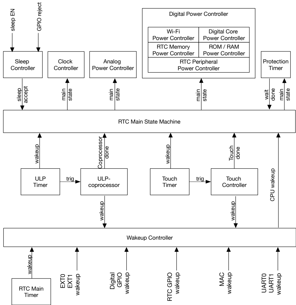
图 9.3-2. 电源管理单元的主要工作流程
