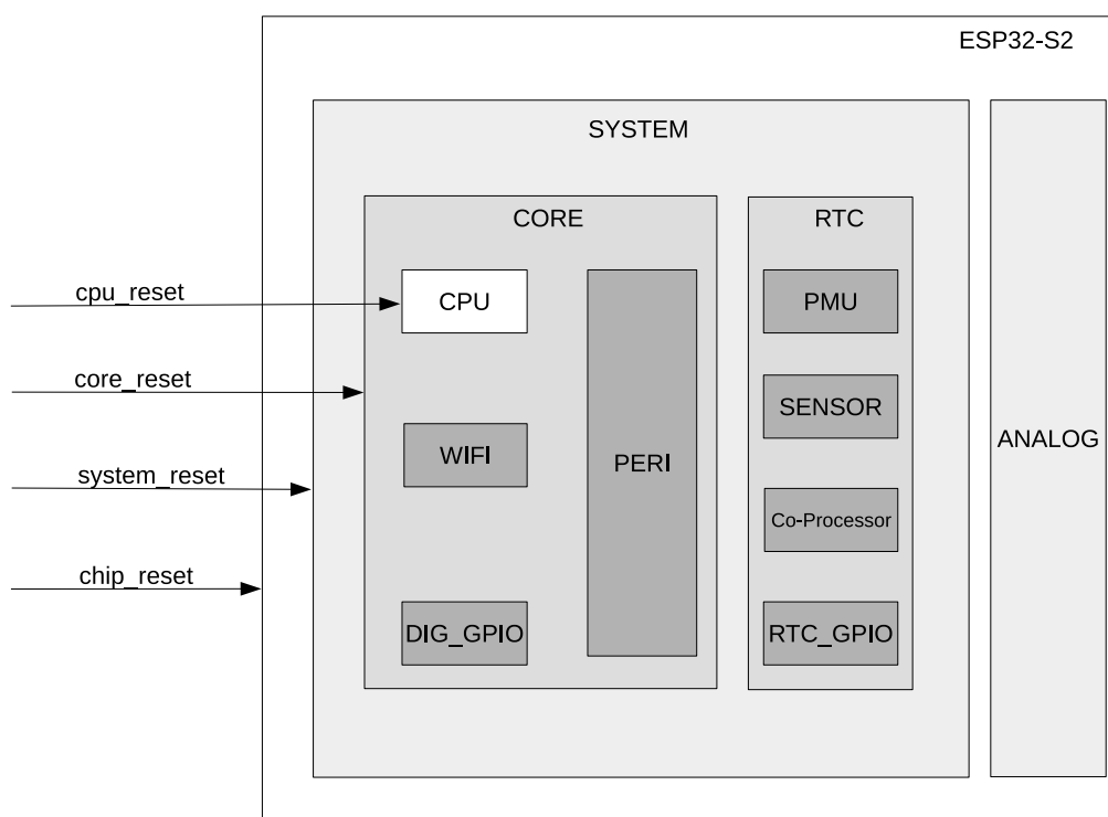
图 6.1-1. 四种复位等级
