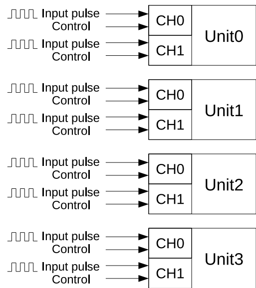
图 27.0-1. PCNT 框图
