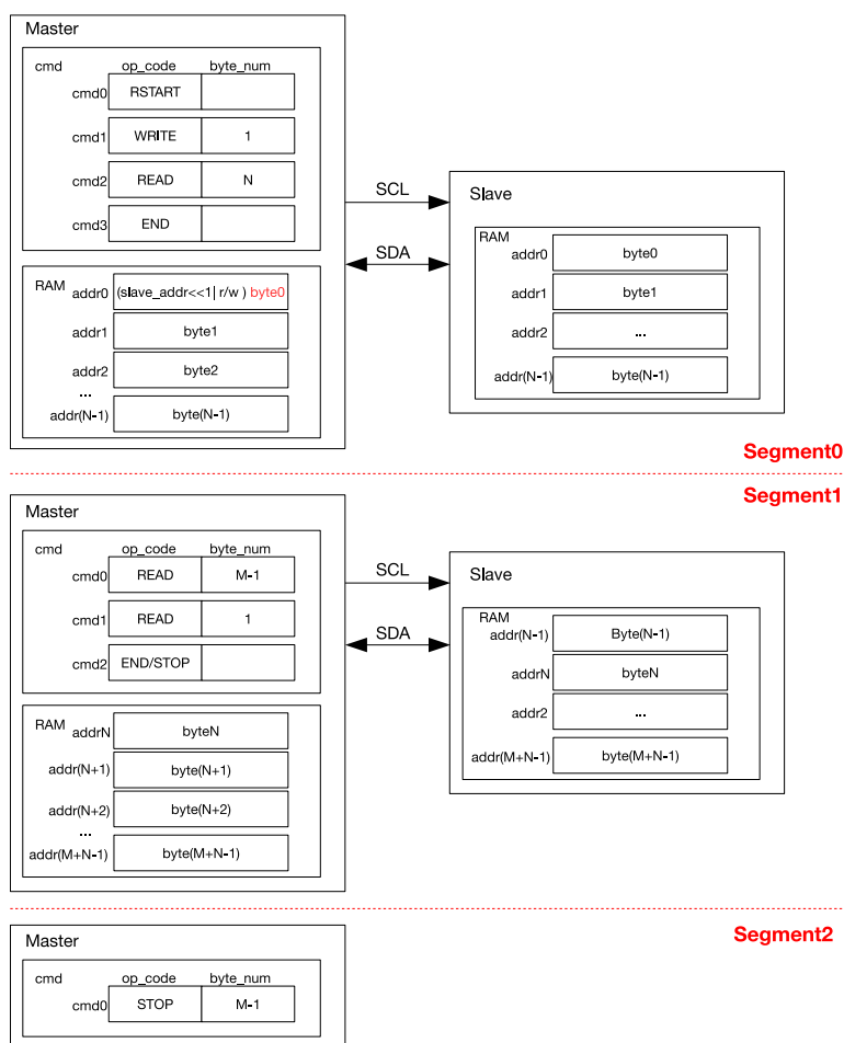
图 25.3-8. I2C Master 分段读 7-bit 寻址的 Slave
