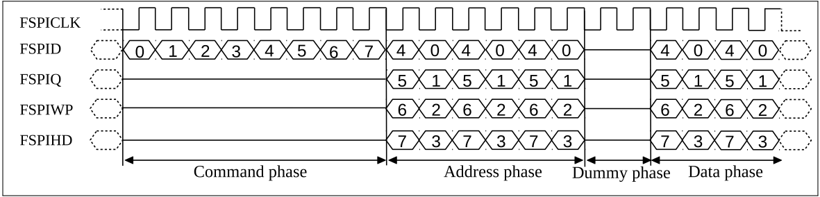
图 24.4-4. GP-SPI2 发送到 Flash 的 SPI Quad 命令序列
