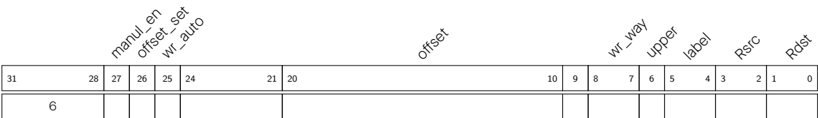
图 1.5-5. 指令类型 - ST
