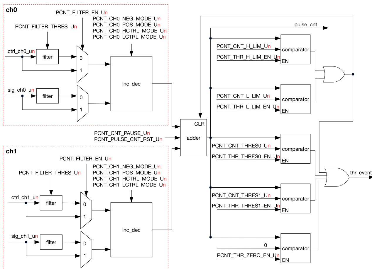
图 27.2-1. PCNT 单元基本架构图
