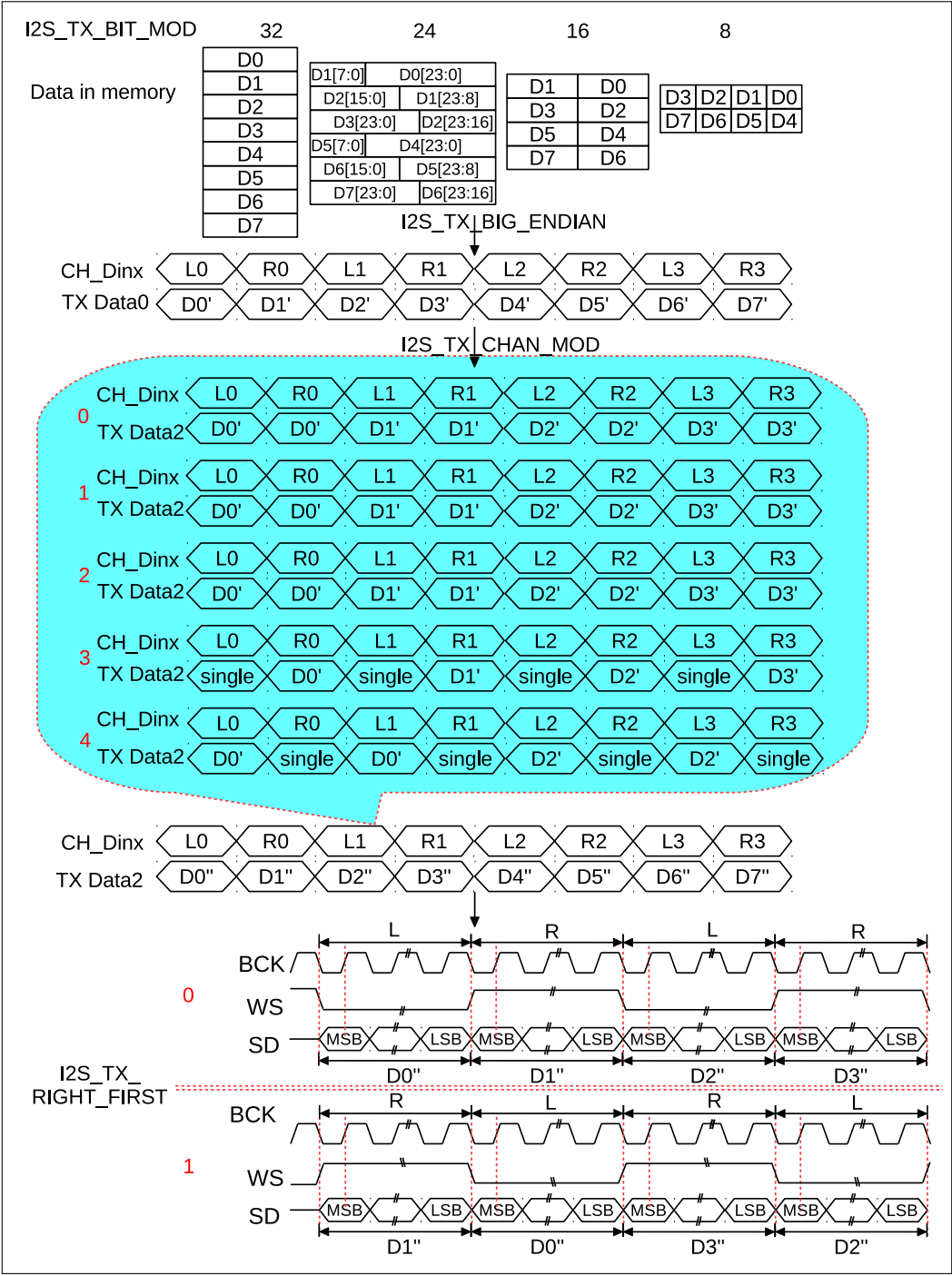
图 26.8-3. I2S_TX_DMA_EQUAL = 1 时，ESP32-S2 I2S 输出数据的控制图
