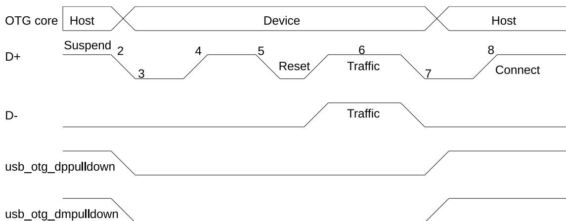
图 28.4-3. A 设备 HNP
