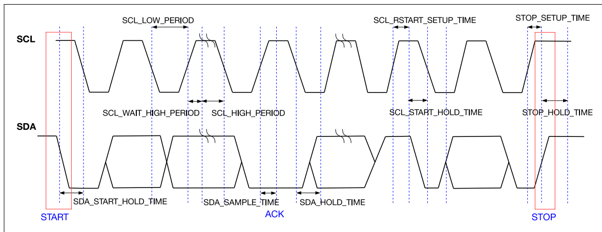
图 25.2-4. I2C 时序图
