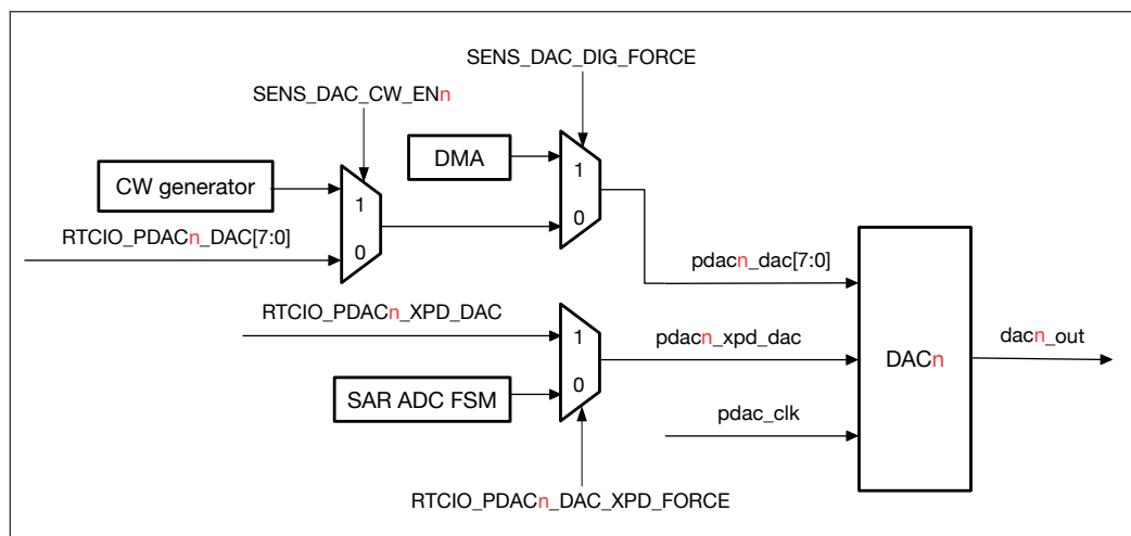
图 32.3-1. DAC 的功能概况
