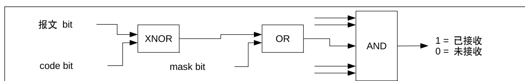
图 29.4-1. 接收滤波器
