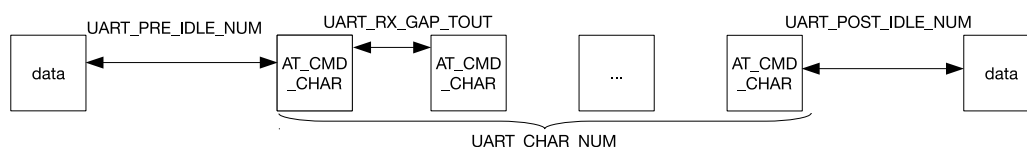
图 23.3-6. AT_CMD 字符格式
