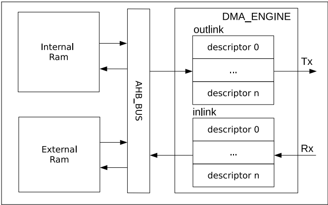
图 2.3-1. DMA 引擎的架构
