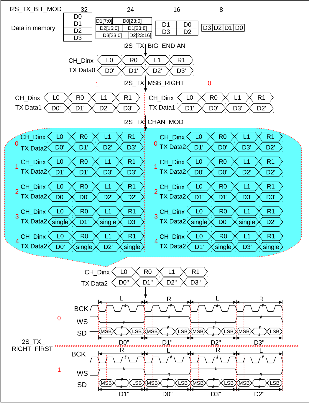
图 26.8-1. 当 I2S_TX_DMA_EQUAL 为零时，ESP32-S2 I2S 发送数据的控制图
