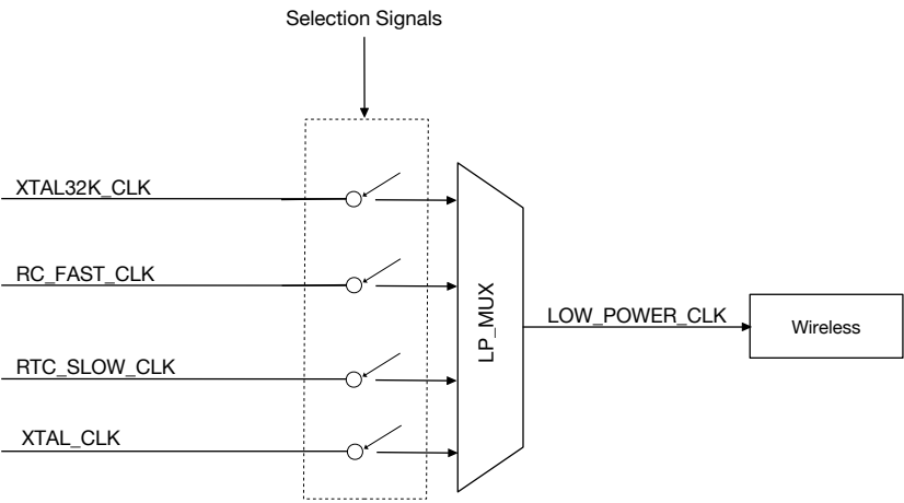
图 9.3-4. RTC 电源域的低功耗时钟
