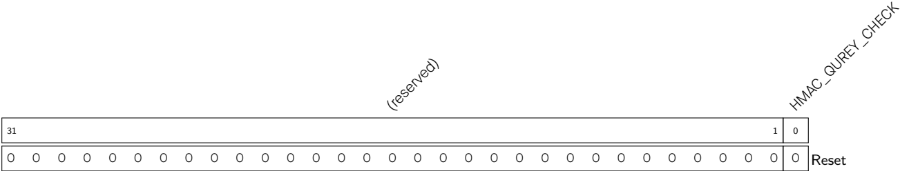
Register 19.9. HMAC_QUERY_ERROR_REG (0x0068)
