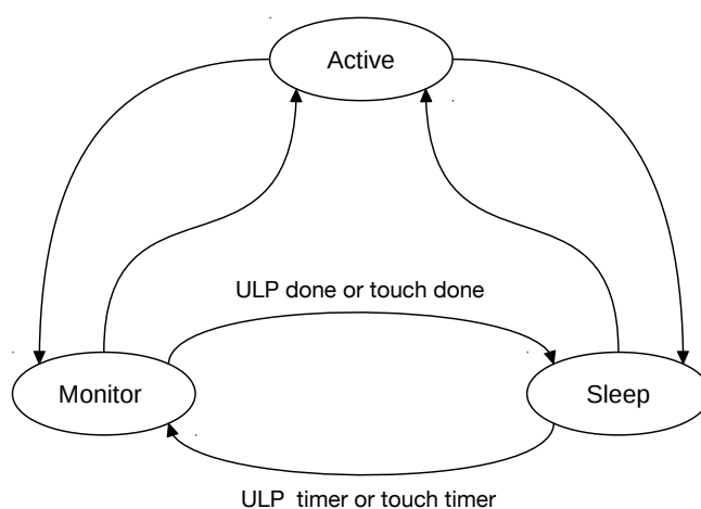
图 9.4-1. RTC 状态转换
