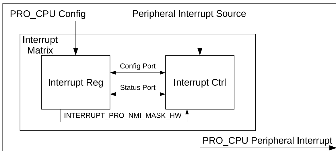
图 8.2-1. 中断矩阵结构图
