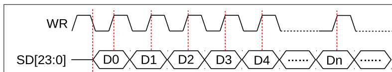
图 26.10-2. LCD 主机发送数据帧格式 1
