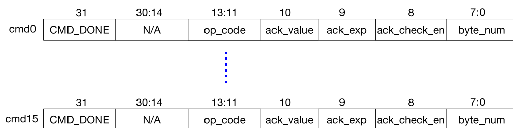
图 25.2-3. I2C 命令寄存器结构
