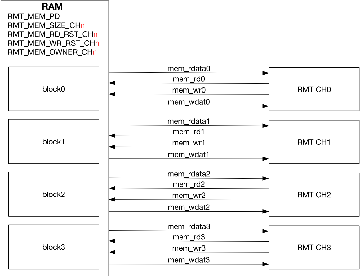
图 31.2-2. RMT 通道
