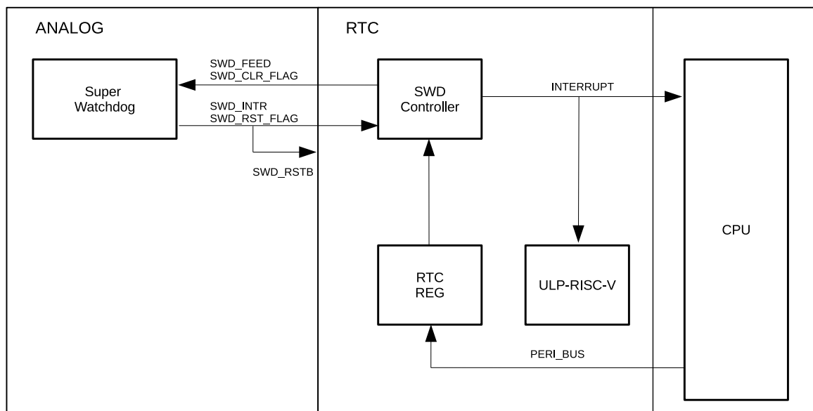
图 12.4-1. 超级看门狗结构
