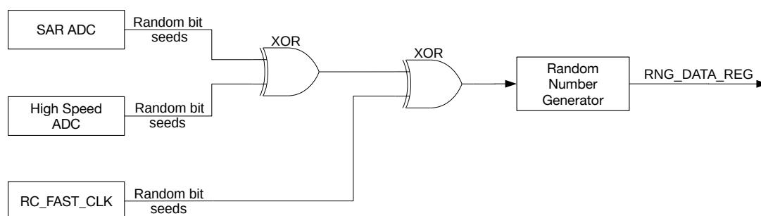
图 22.3-1. 噪声源
