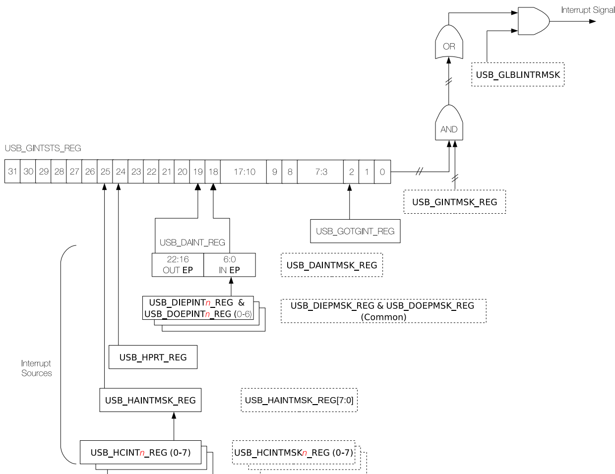
图 28.3-5. OTG_FS 中断层次结构图
