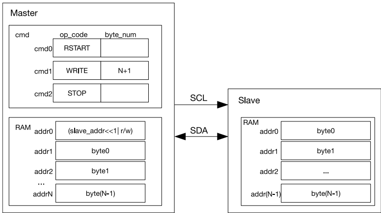
图 25.3-1. I2C Master 写 7-bit 寻址的 Slave
