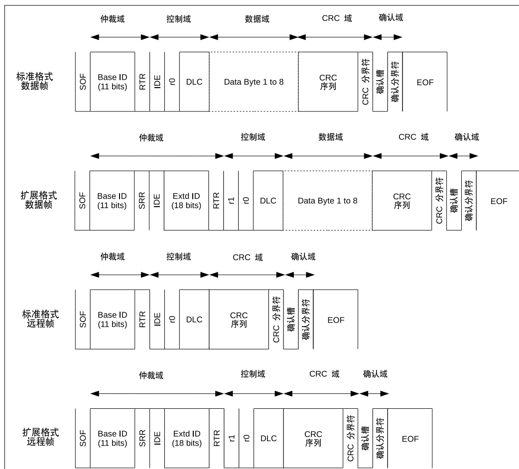
图 29.2-1. 数据帧和远程帧中的位域
