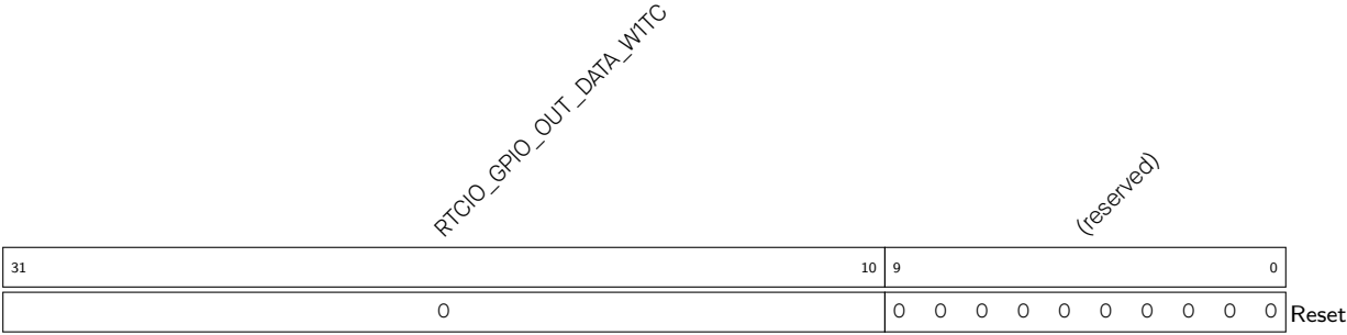
Register 5.54. RTCIO_RTC_GPIO_OUT_W1TC_REG (0x0008)
