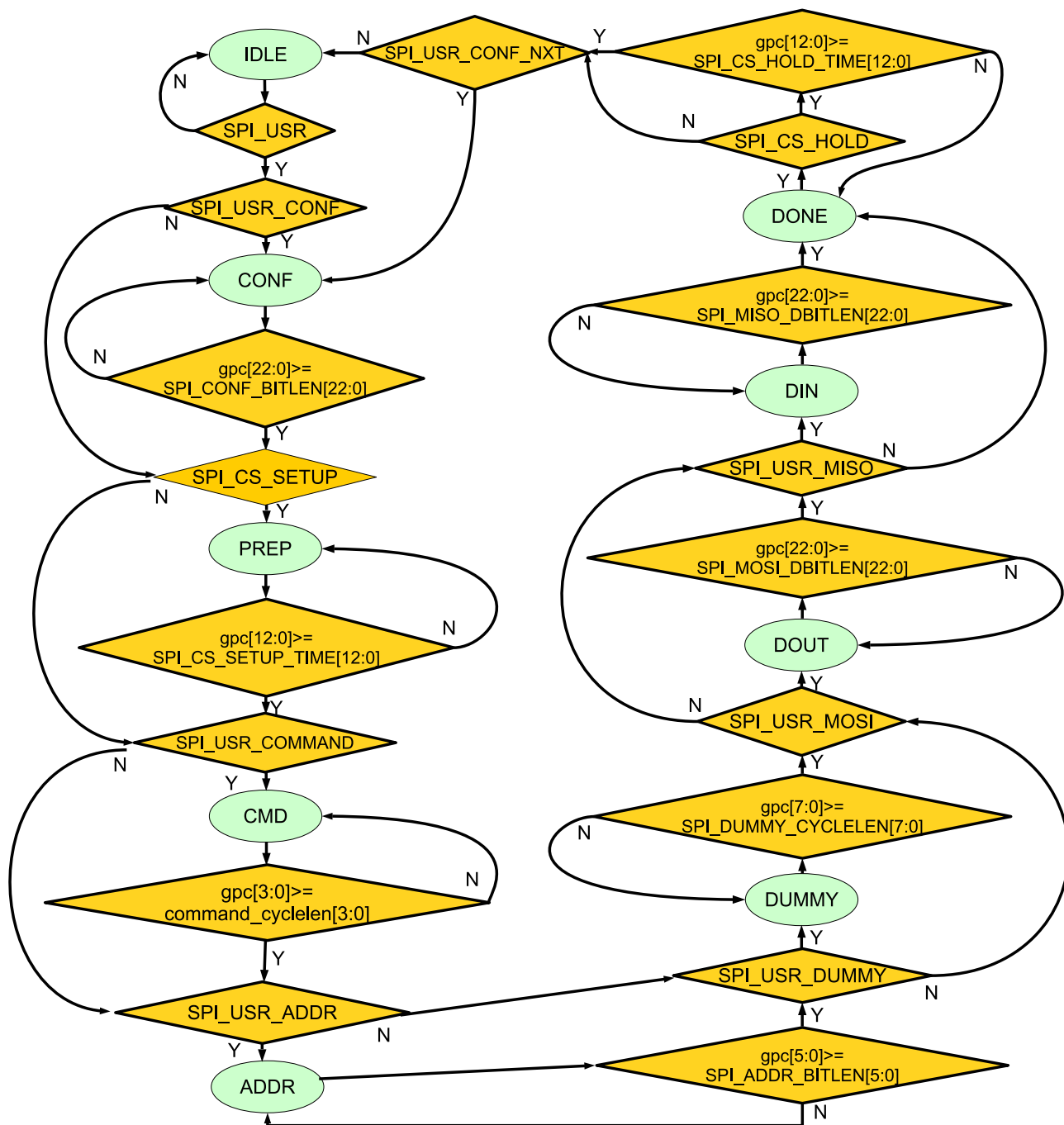
图 24.4-1. GP-SPI2 主机模式流程图
