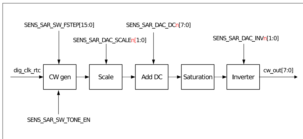
图 32.3-2. 余弦波形生成器的工作流程
