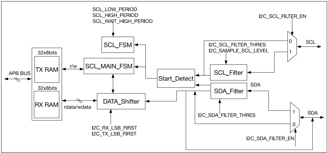
图 25.2-2. I2C Slave 基本架构
