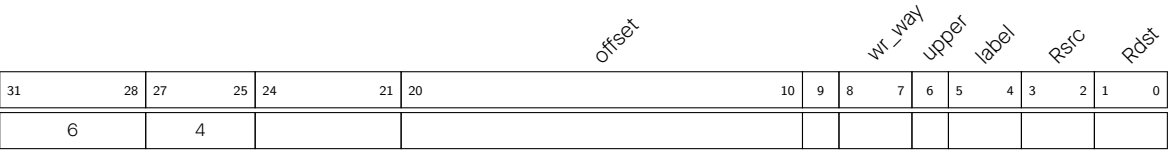
图 1.5-9. 指令类型 - 指定地址模式的数据存储
