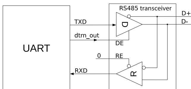
图 23.3-7. RS485 模式驱动控制结构图
