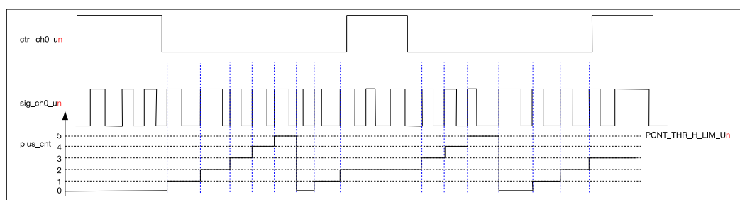
图 27.3-1. 通道 0 递增计数图
