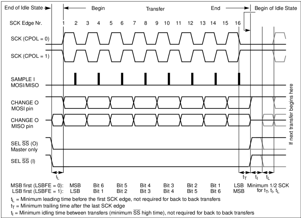
图 24.9-2. SPI 时钟模式 1 和时钟模式 3
