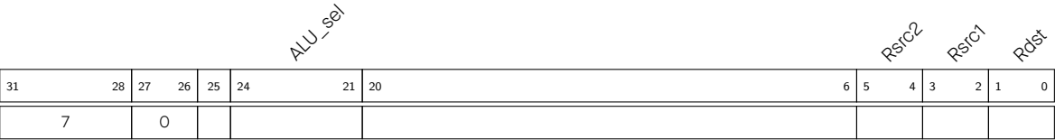
图 1.5-2. 指令类型 - 对寄存器数值的 ALU 运算
