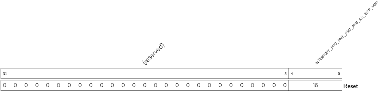
Register 8.56. INTERRUPT_PRO_PMS_PRO_AHB_ILG_INTR_MAP_REG (0x0138)
