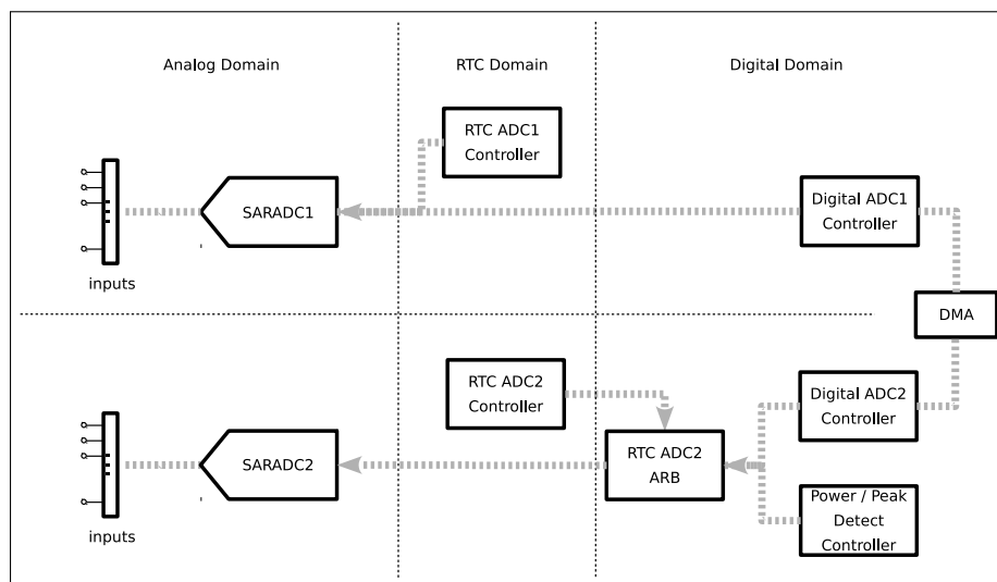
图 32.2-1. SAR ADC 概图
