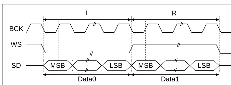
图 26.4-2. MSB 对齐标准
