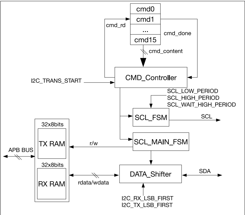
图 25.2-1. I2C Master 基本架构
