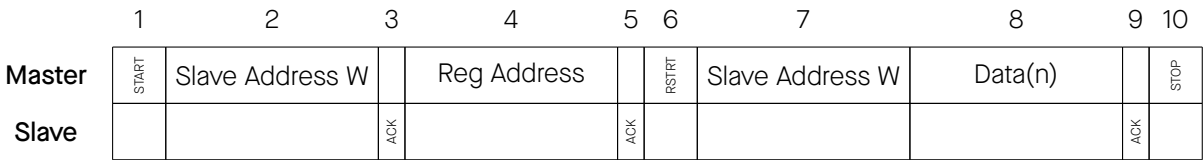
图 1.7-2. I2C 写操作
