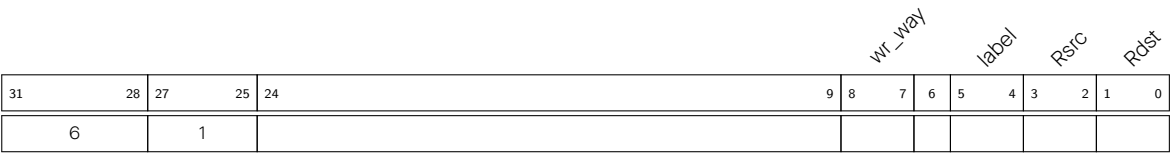
图 1.5-7. 指令类型 - 地址自增模式的数据存储 (ST-AUTO-DATA)
