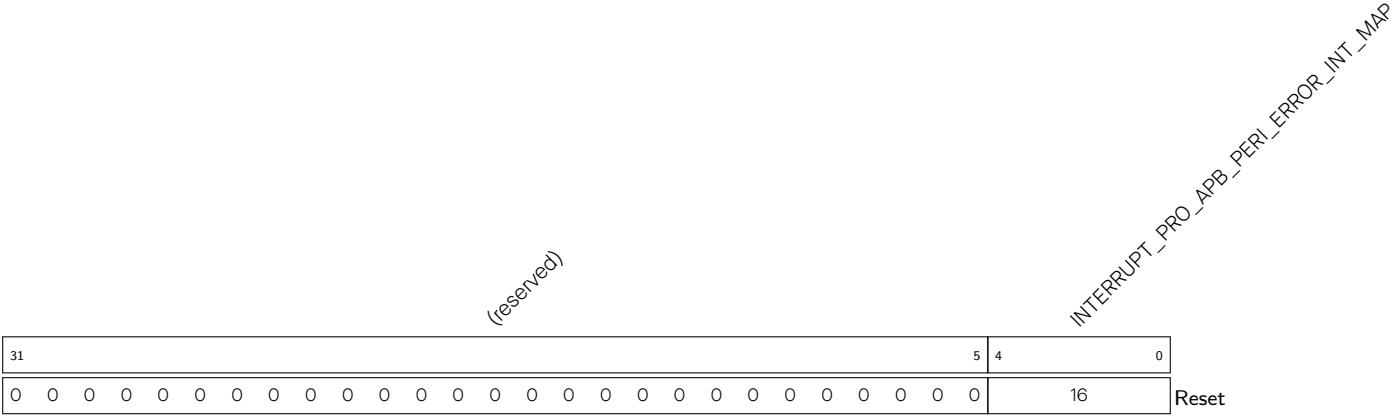
Register 8.68. INTERRUPT_PRO_APB_PERI_ERROR_INT_MAP_REG (0x0170)
