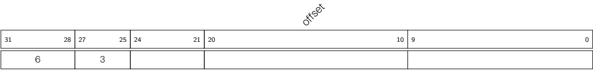
图 1.5-6. 指令类型 - 地址自增模式的基地址偏移 (ST-OFFSET)
