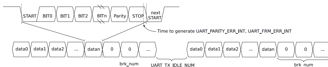
图 23.3-5. UART 数据帧结构
