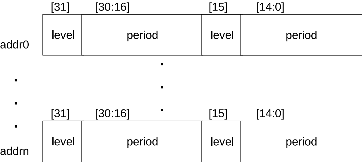
图 31.2-3. RAM 中脉冲编码结构
