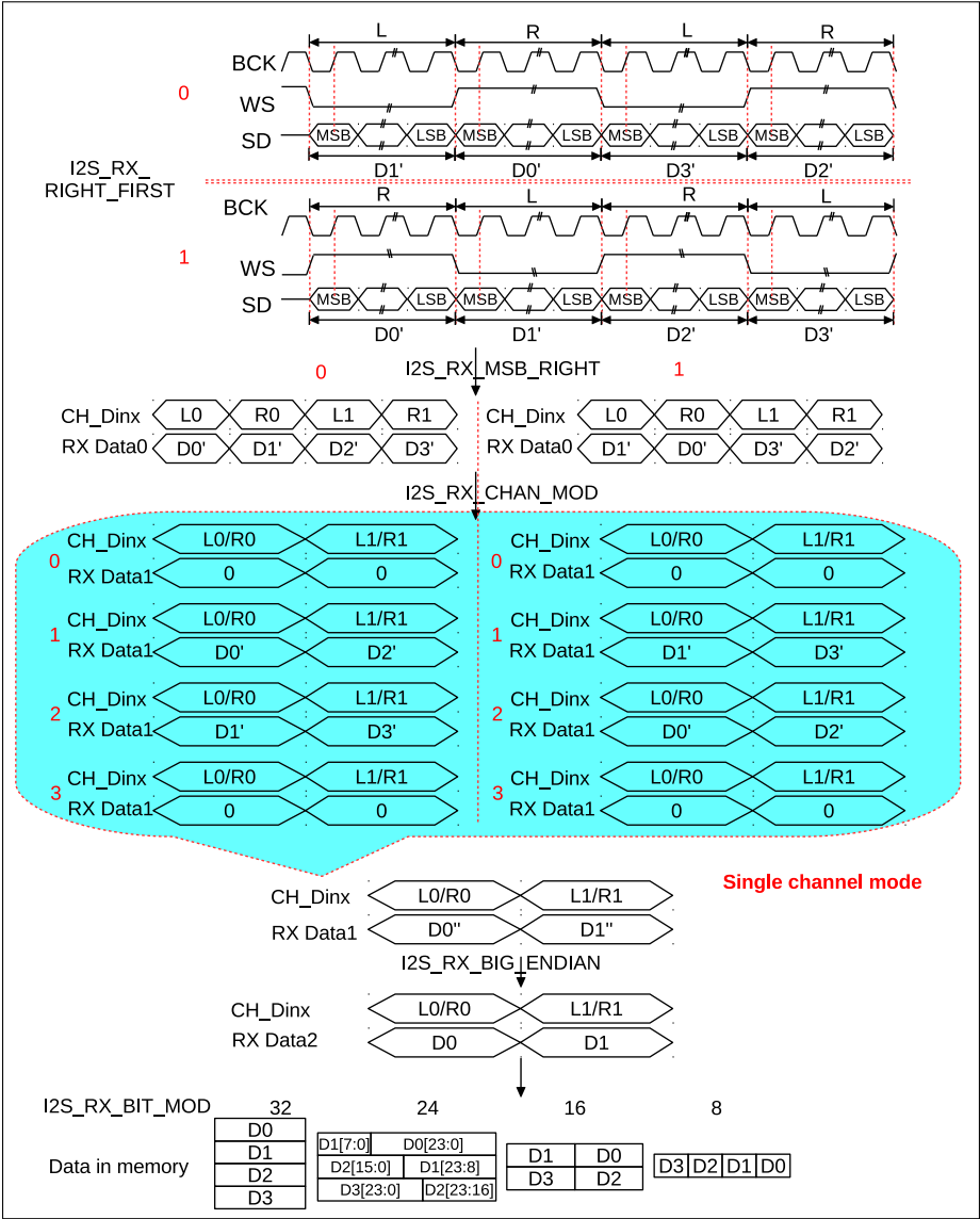
图 26.9-3. I2S_RX_DMA_EQUAL = 1 时，ESP32-S2 I2S 接收数据的控制图
