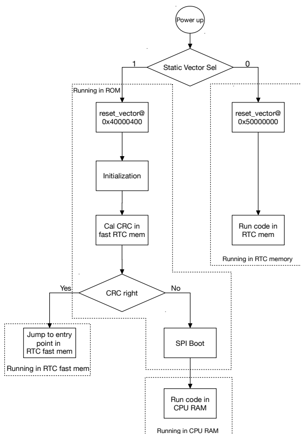
图 9.5-1. ESP32-S2 启动流程图
