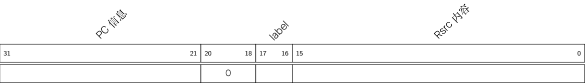
图 1.5-8. MEM[Rdst + Offset] 写全字
