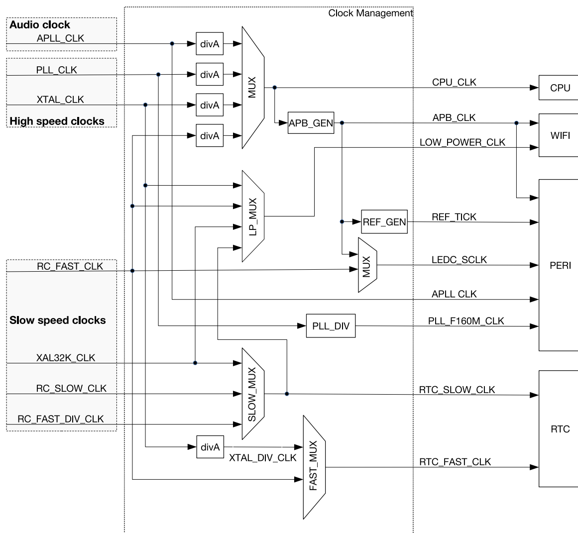
图 6.2-1. 系统时钟
