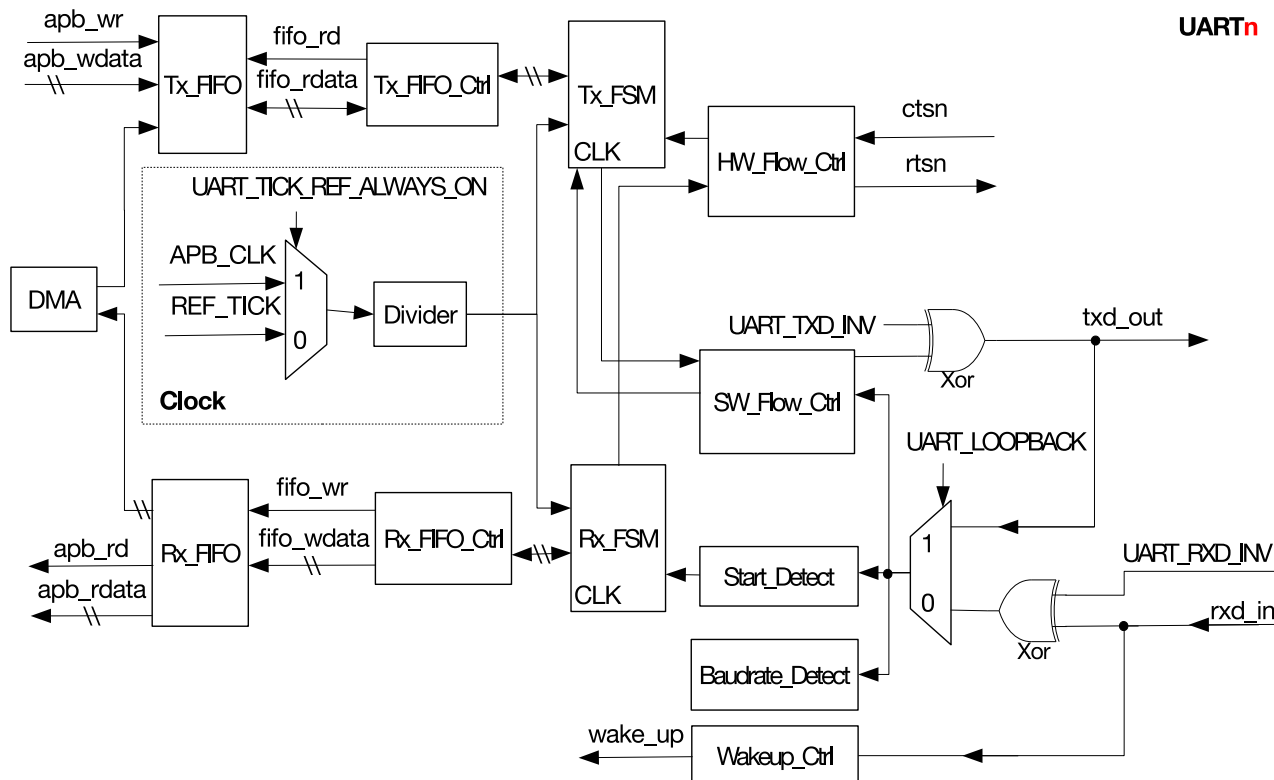
图 23.3-1. UART 基本架构图
