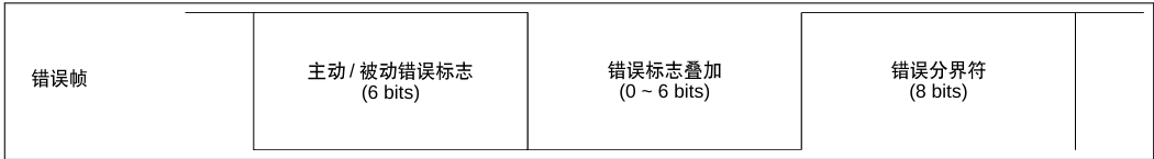
图 29.2-2. 错误帧中的位域
