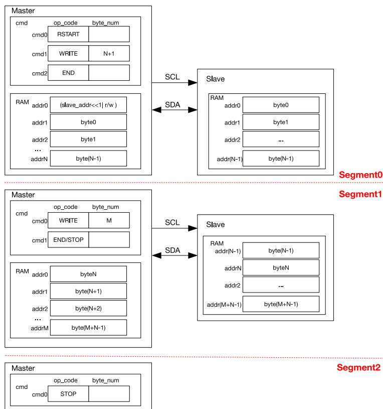
图 25.3-4. I2C Master 分段写 7-bit 寻址的 Slave
