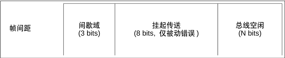
图 29.2-4. 帧间距中的域
