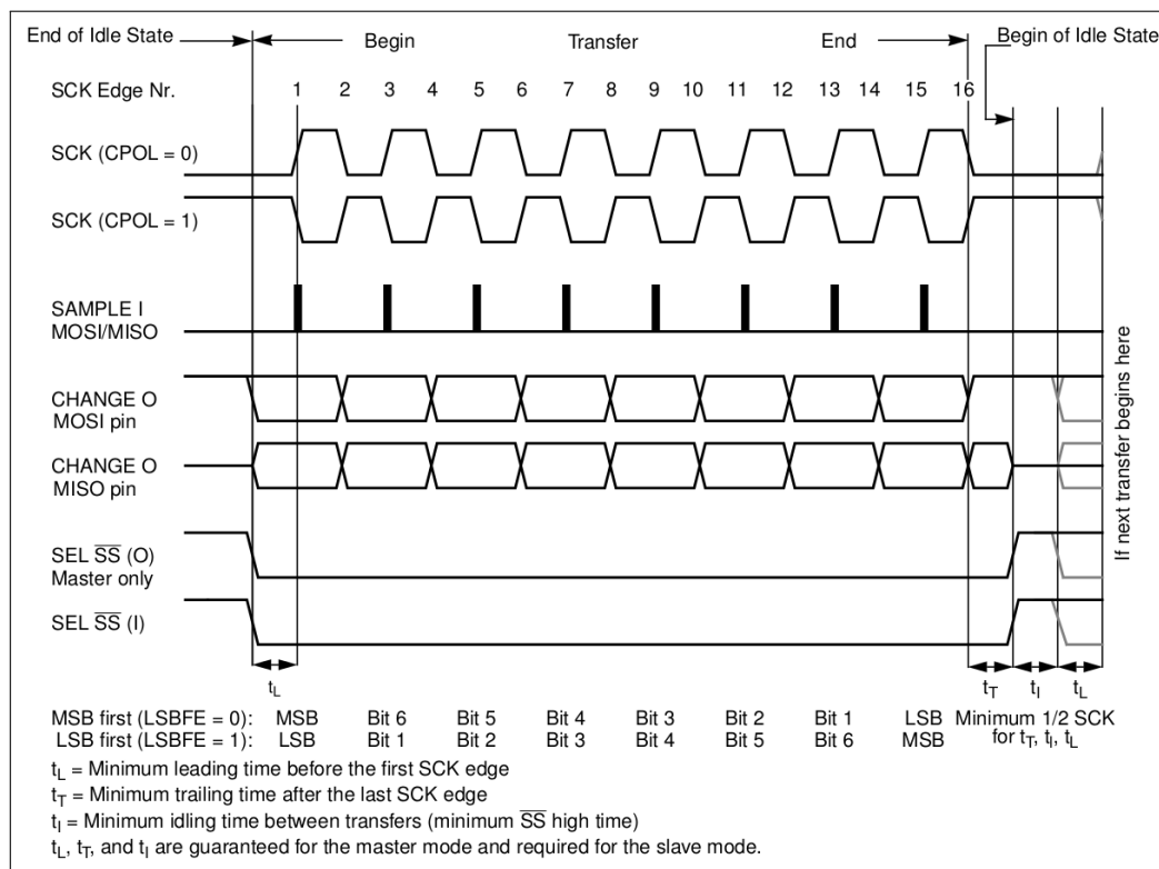
图 24.9-1. SPI 时钟模式 0 和时钟模式 2
