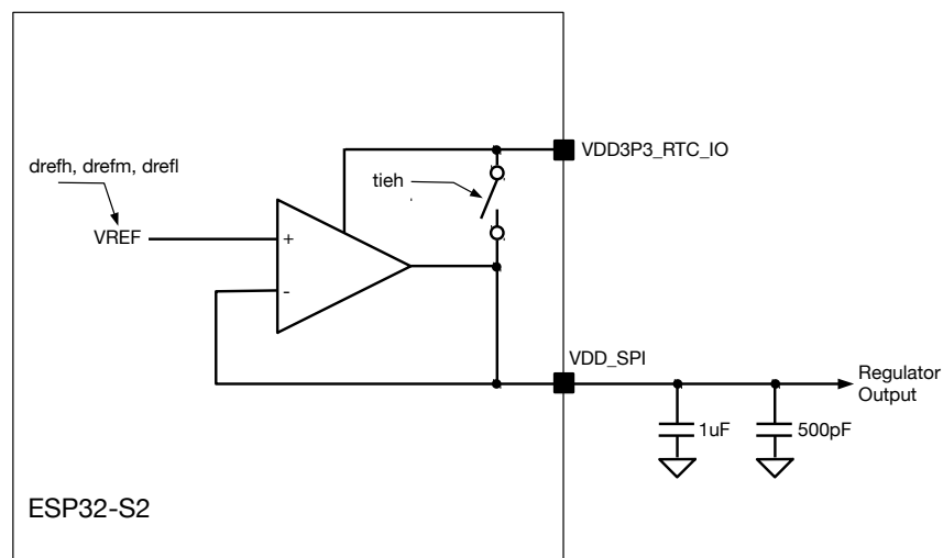
图 9.3-7. Flash 调压器
