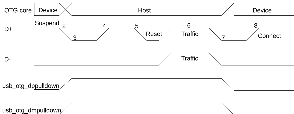
图 28.4-4. B 设备 HNP
