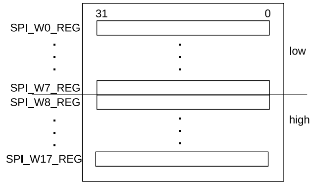
图 24.7-1. CPU 控制模式下使用的数据 Buffer
