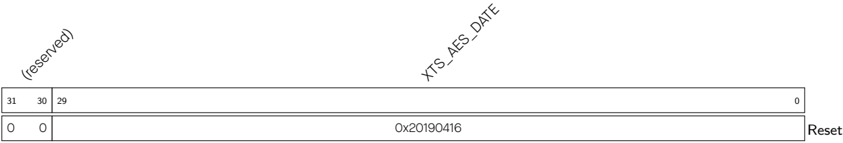
Register 21.9. XTS_AES_DATE_REG (0x015C)
