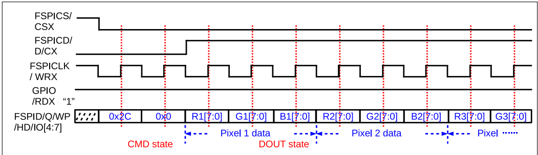
图 24.4-6. 发送至 8-bit LCD 驱动的写命令序列
