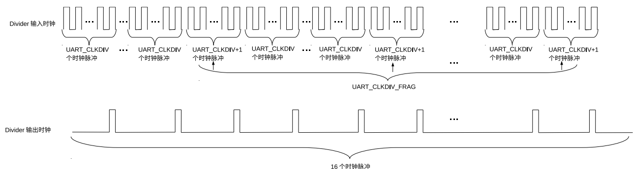
图 23.3-3. UART 控制器分频
