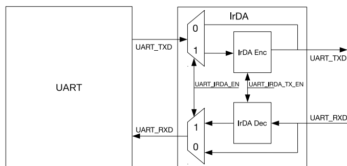
图 23.3-9. IrDA 编解码结构图
