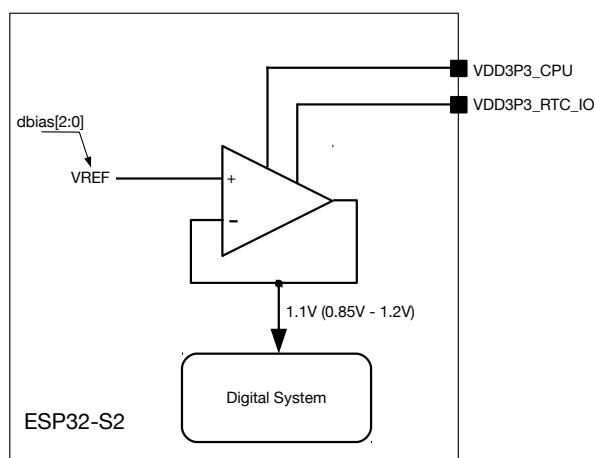
图 9.3-5. 数字系统调压器
