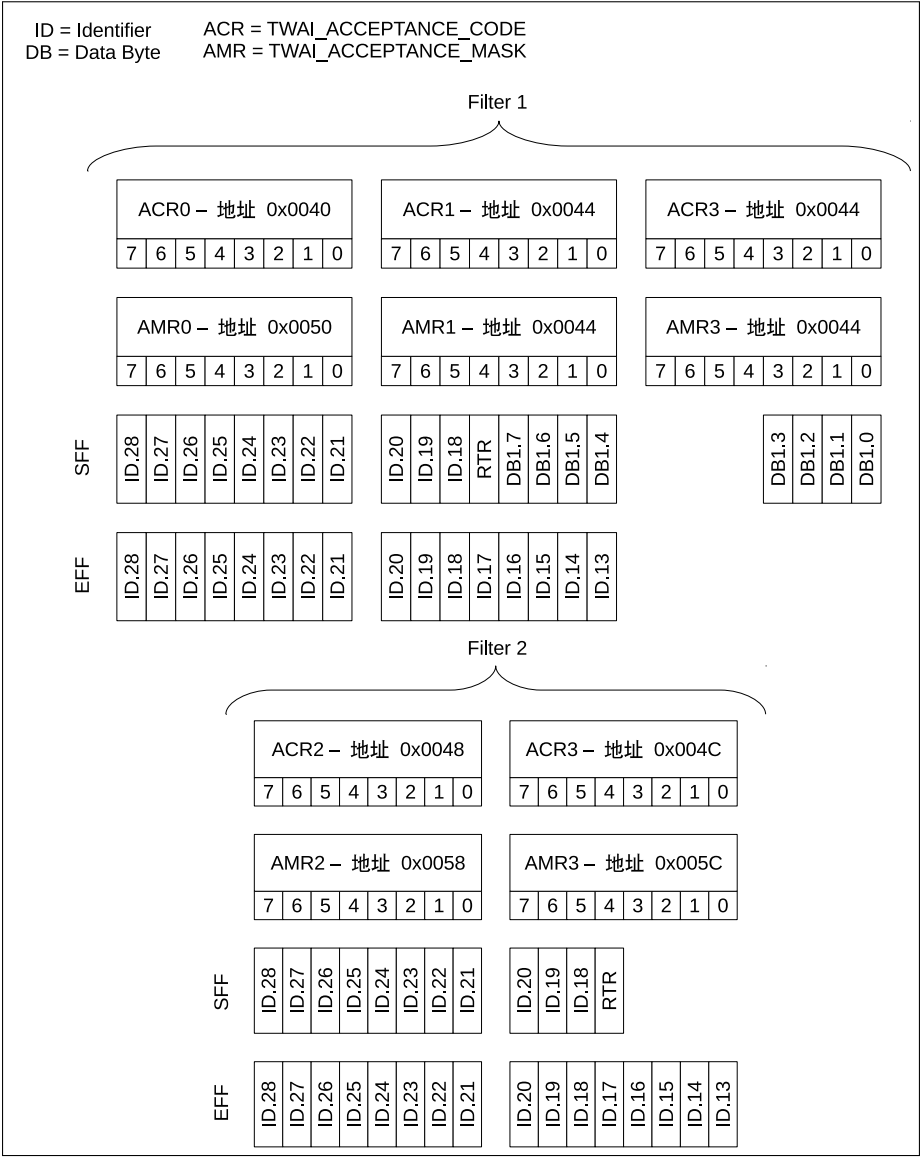
图 29.4-3. 双滤波模式
