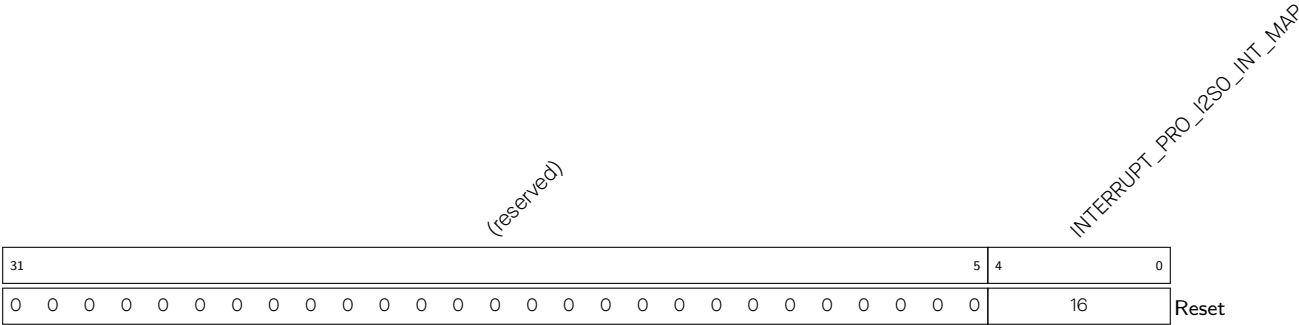
Register 8.21. INTERRUPT_PRO_I2SO_INT_MAP_REG (0x008C)
