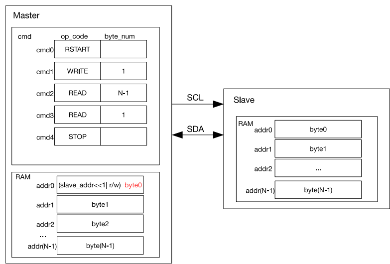
图 25.3-5. I2C Master 读 7-bit 寻址的 Slave
