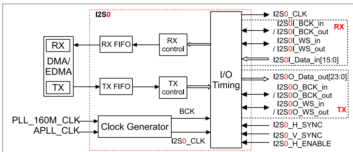
图 26.2-1. ESP32-S2 I2S 系统框图
