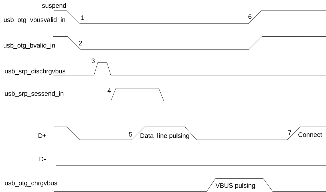
图 28.4-2. B 设备 SRP
