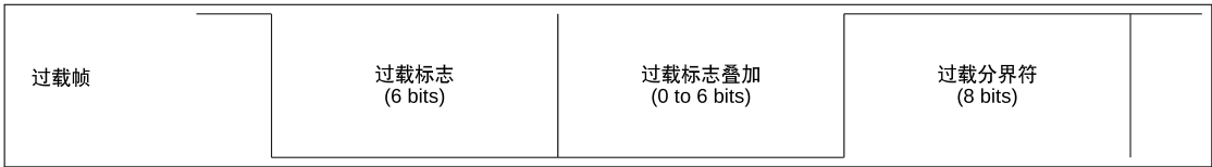
图 29.2-3. 过载帧中的位域
