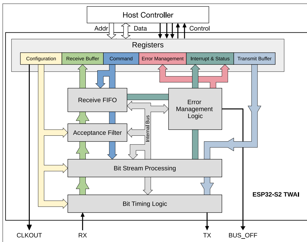
图 29.3-1. TWAI 概略图
