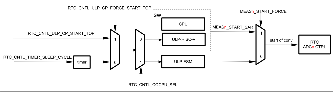
图 32.2-3. RTC ADC 控制器功能概况
