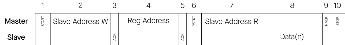
图 1.7-1. I2C 读操作
