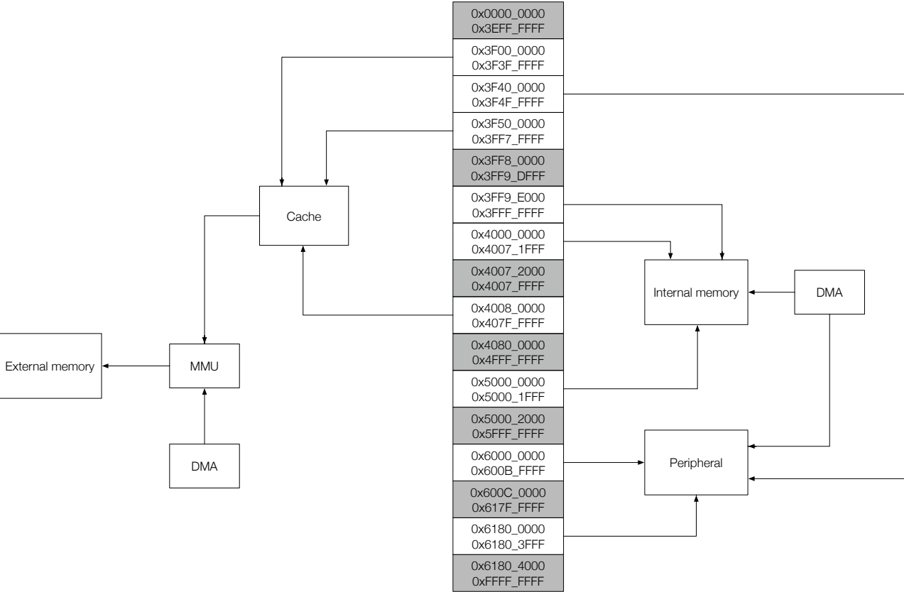
图 3.2-1. 系统结构与地址映射结构
