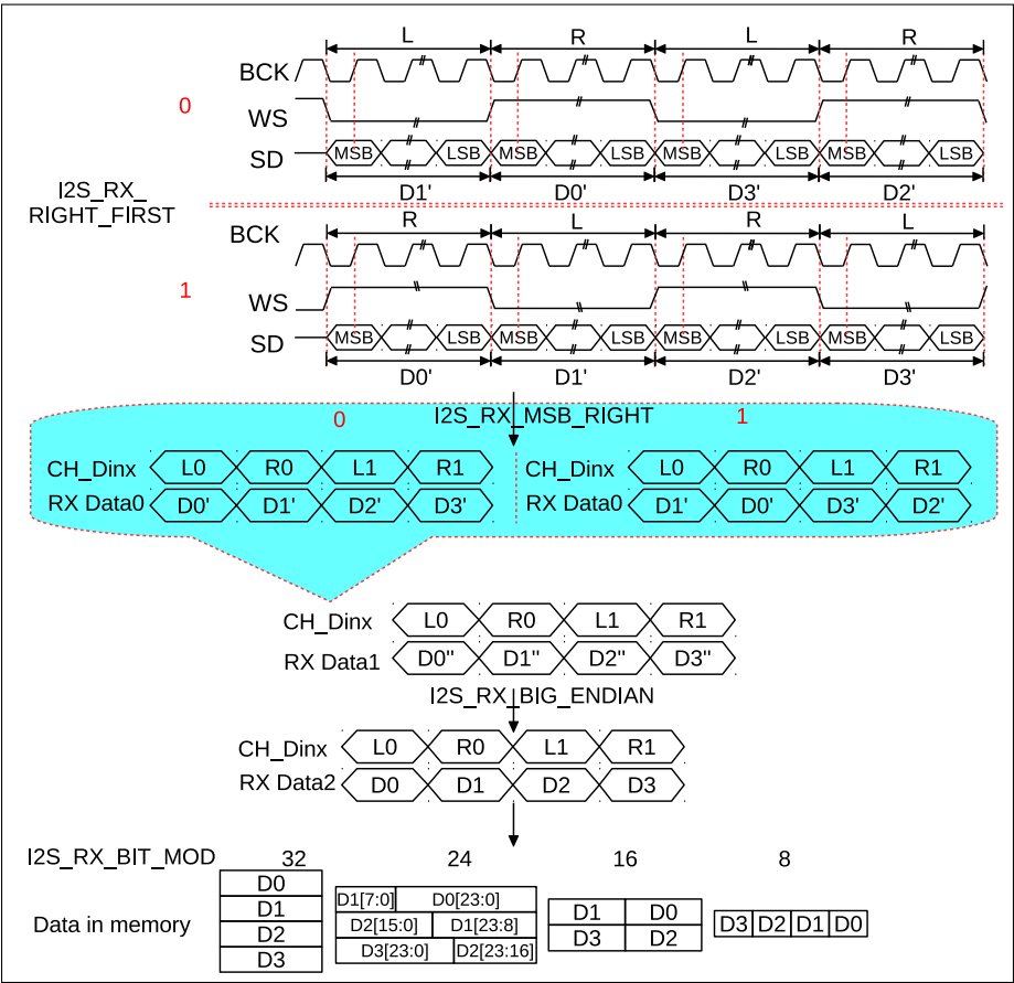
图 26.9-1. I2S_RX_DMA_EQUAL = 0 时，ESP32-S2 I2S 接收数据的控制图
