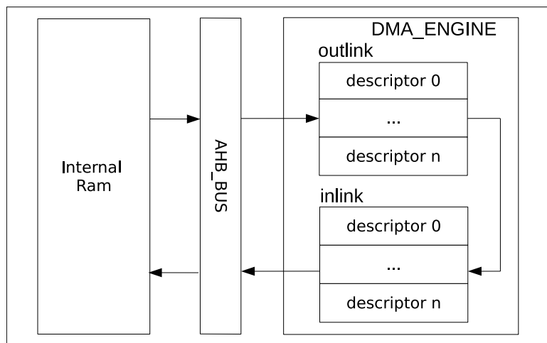
图 2.4-1. Copy DMA 引擎架构
