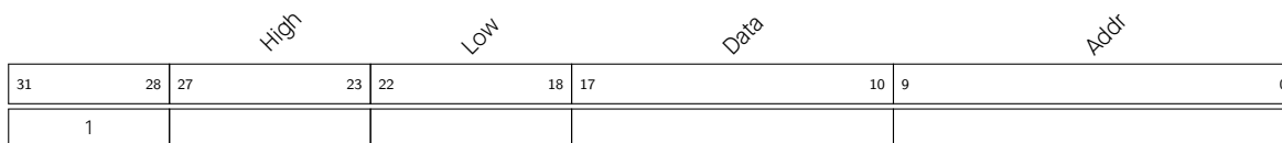
图 1.5-20. 指令类型 - REG_WR
