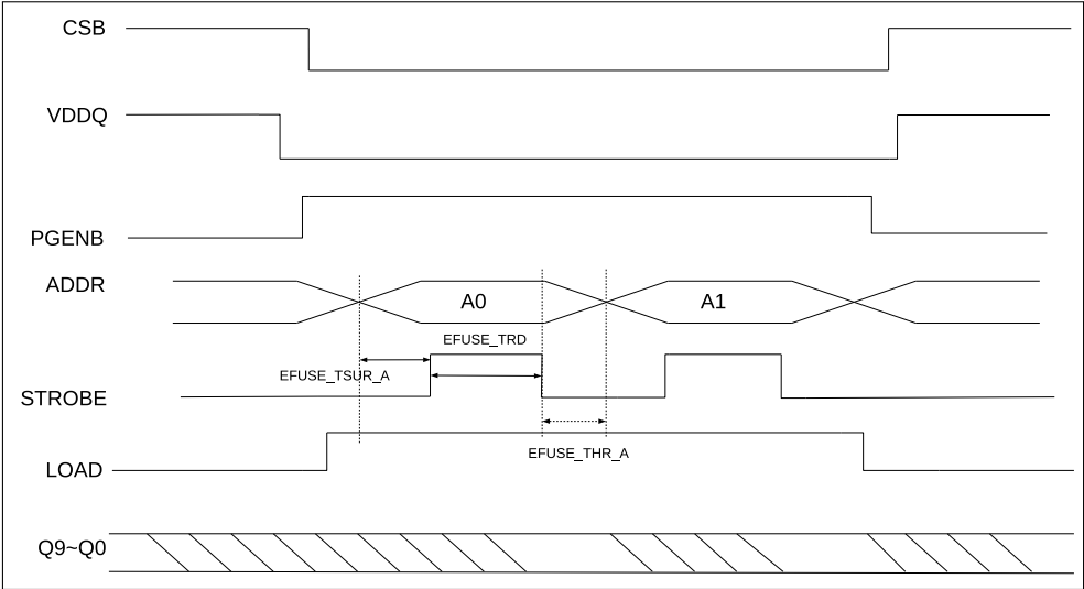
图 4.3-4. eFuse 读取时序图
