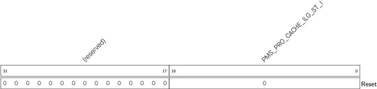
Register 14.47. PMS_PRO_CACHE_3_REG (0x0084)
