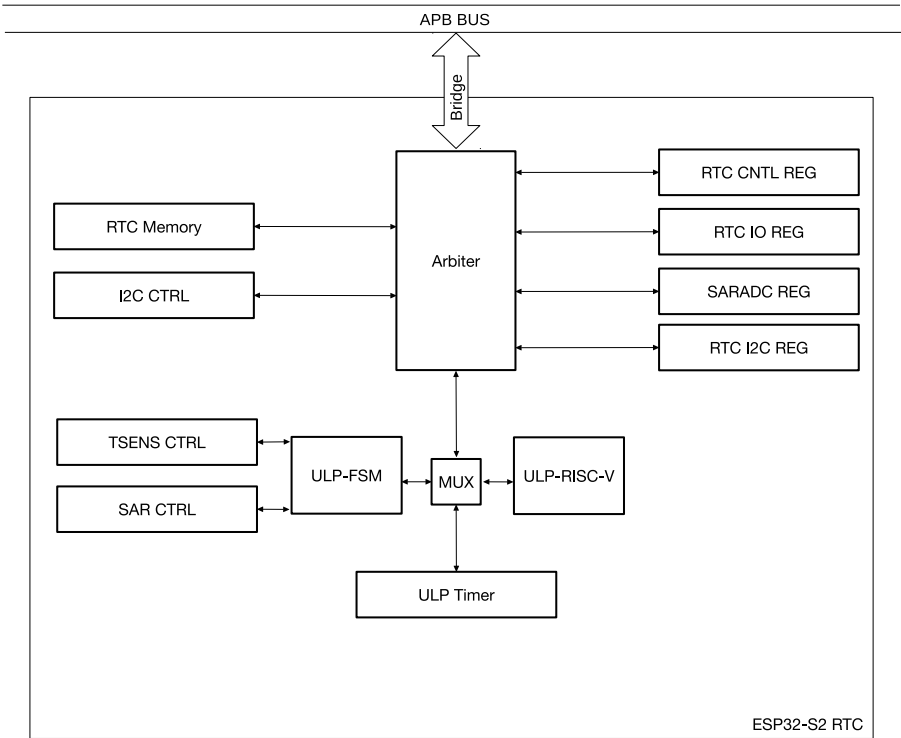
图 1.2-1. 超低功耗协处理器基本架构
