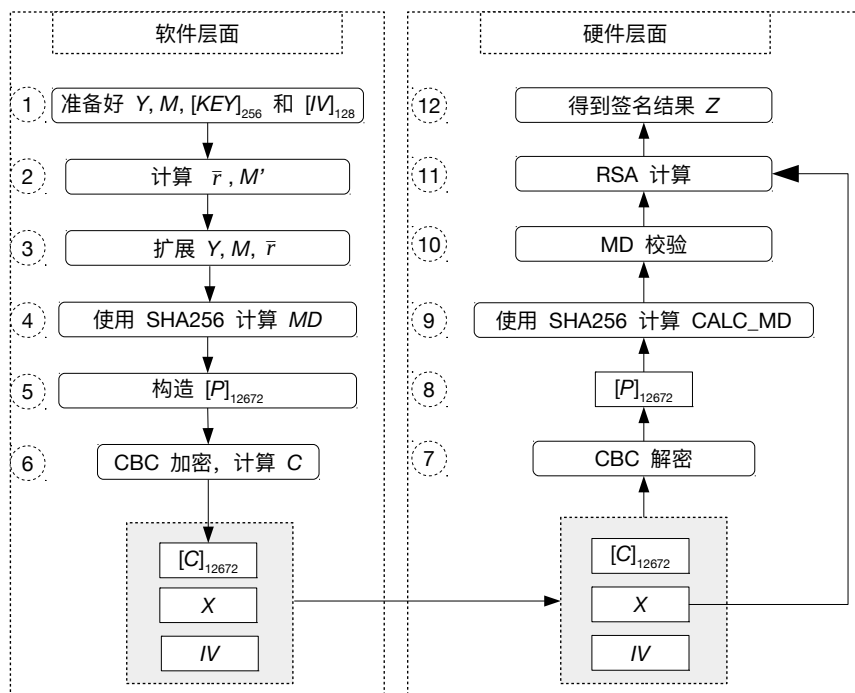
图 20.3-1. 软件准备工作与硬件工作流程
