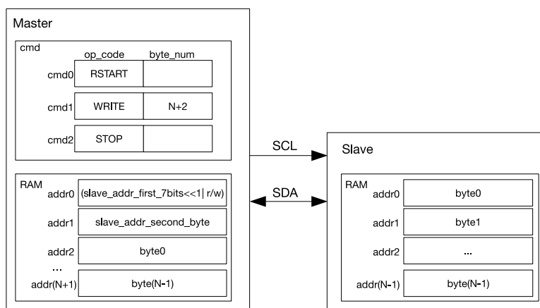
图 25.3-2. I2C Master 写 10-bit 寻址的 Slave
