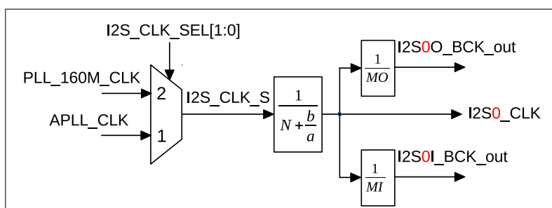
图 26.5-1. I2S 时钟
