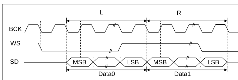
图 26.4-1. Philips 标准
