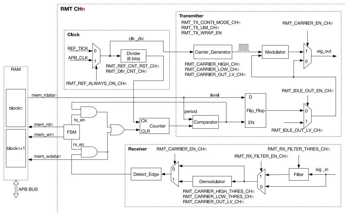
图 31.2-1. RMT 结构框图
