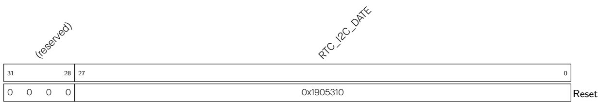
Register 1.44. RTC_I2C_DATE_REG (0x00FC)
