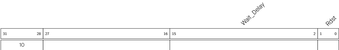
图 1.5-17. 指令类型 - TSENS
