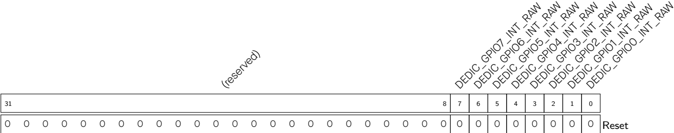
Register 5.48. DEDIC_GPIO_INTR_RAW_REG (0x0020)
