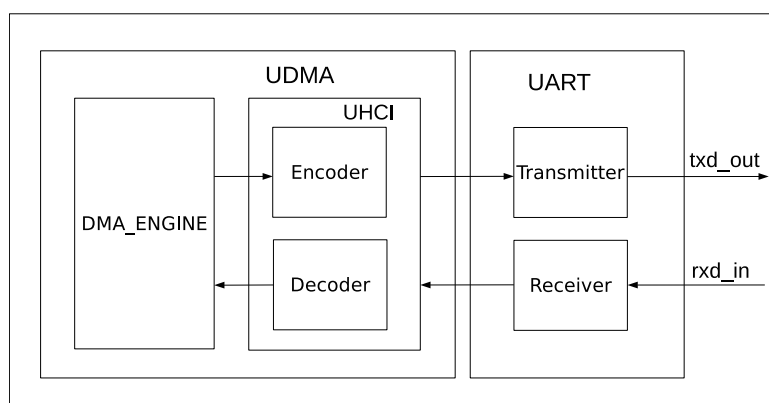
图 2.5-1. UDMA 模式数据传输
