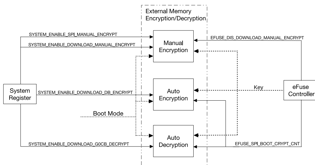
图 21.3-1. 片外存储器加解密模块架构
