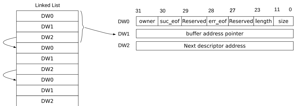
图 2.3-2. 链表结构图
