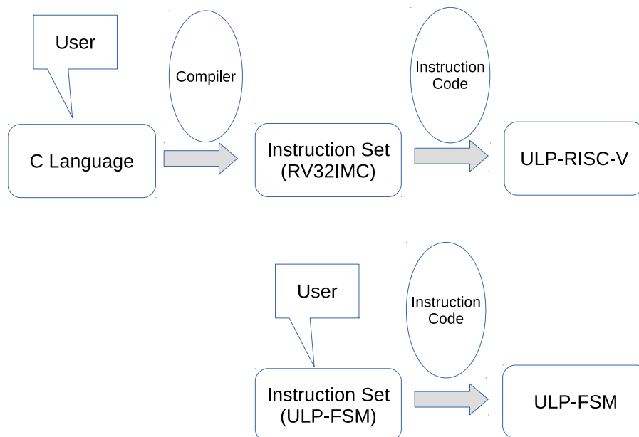
图 1.3-1. 编程流程图
