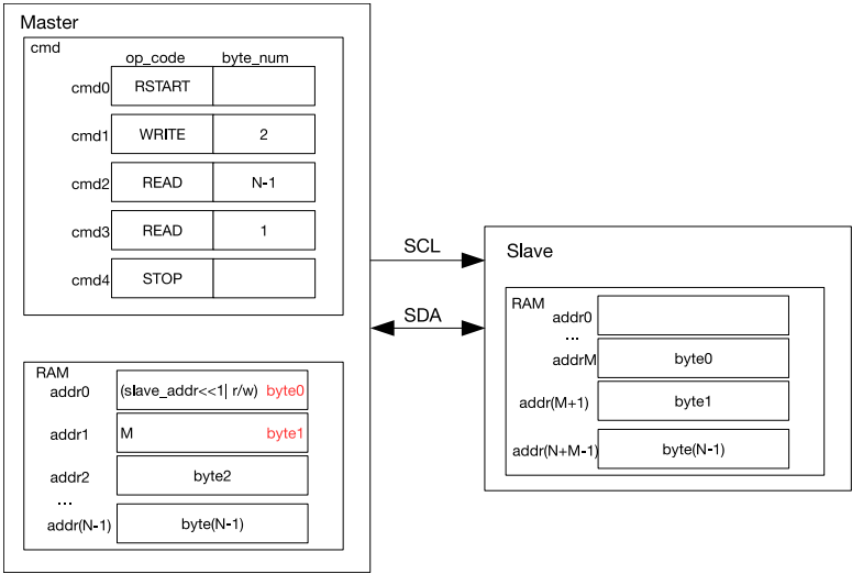
图 25.3-7. I2C Master 从 7-bit 寻址 Slave 的 M 地址读取 N 个数据
