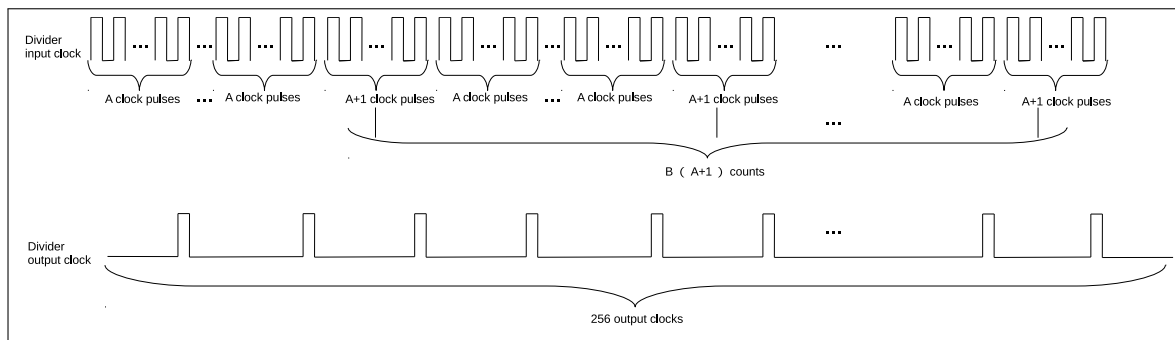
图 30.3-3. LED_PWM 分频器
