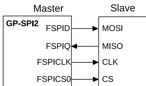
图 24.4-2. GP-SPI2 主机使用全双工模式与 SPI 从机通信框图
