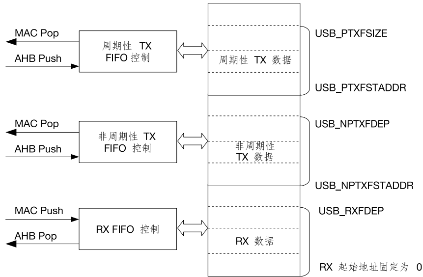
图 28.3-3. 主机模式 FIFO
