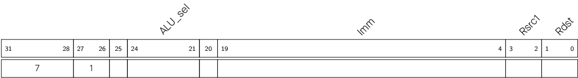
图 1.5-3. 指令类型 - 对指令立即值的 ALU 运算
