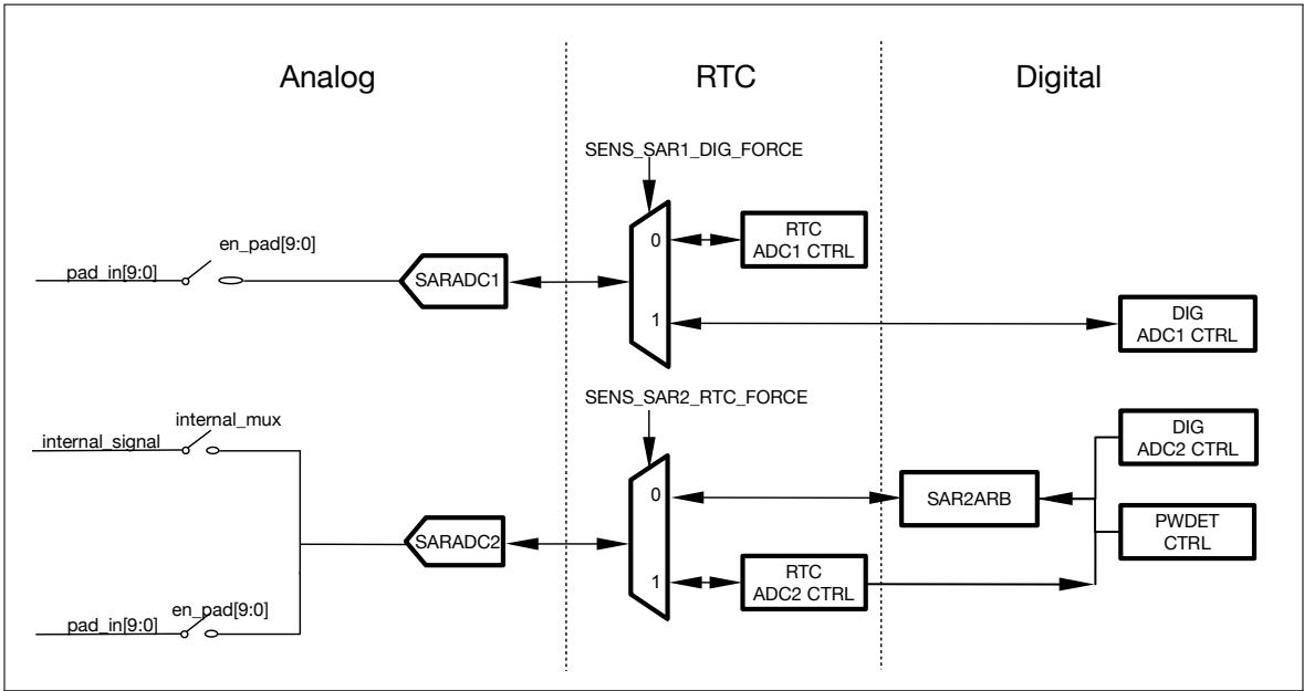
图 32.2-2. SAR ADC 的功能概况
