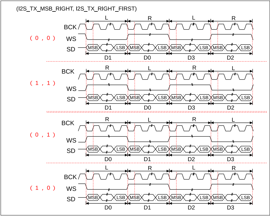
图 26.8-2. I2S_TX_CHAN_MOD[2:0] = 0 且 I2S_TX_DMA_EQUAL = 0 时，ESP32-S2 I2S 输出数据的波形图
