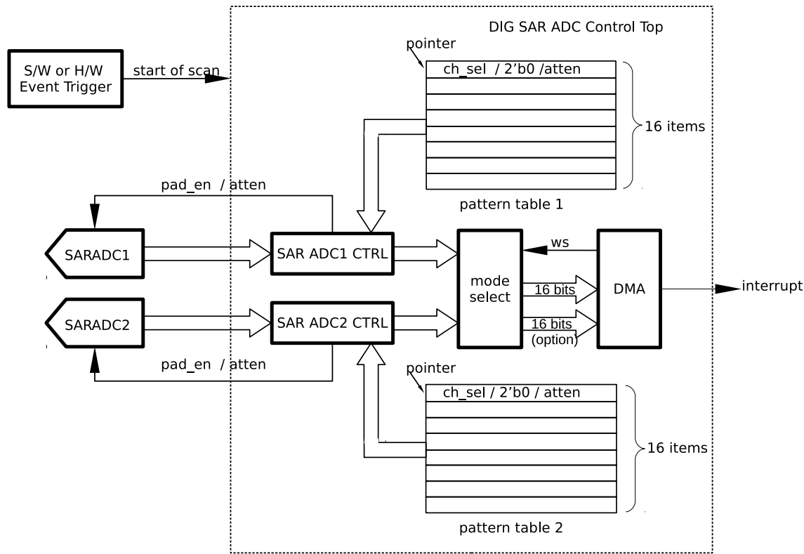
图 32.2-4. DIG ADC 控制器概况
