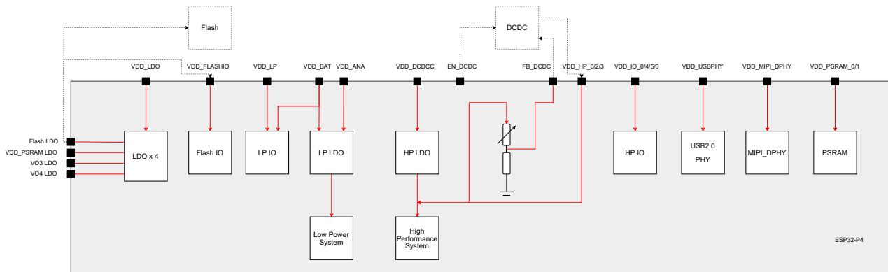
图 2-2. ESP32-P4 电源管理
