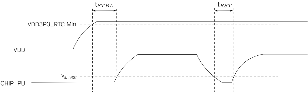
图 7: 上电和复位时序参数图
