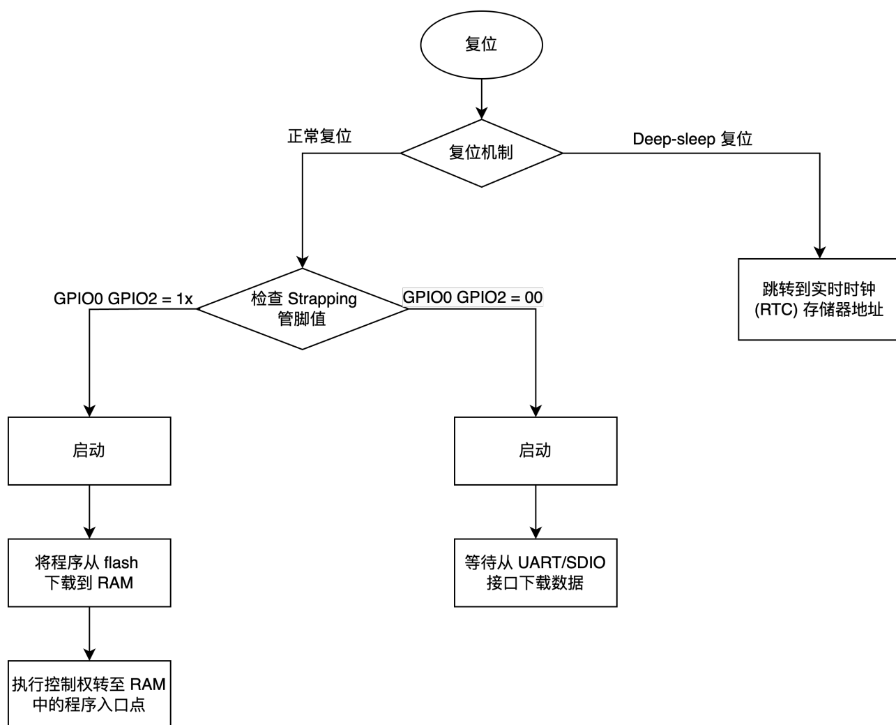
图 6: 芯片启动流程
