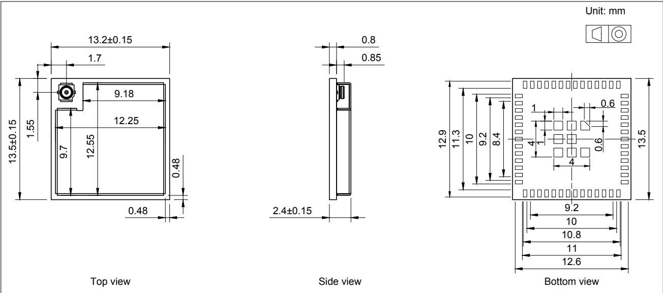
图 12: ESP32-MINI-1U 模组尺寸
