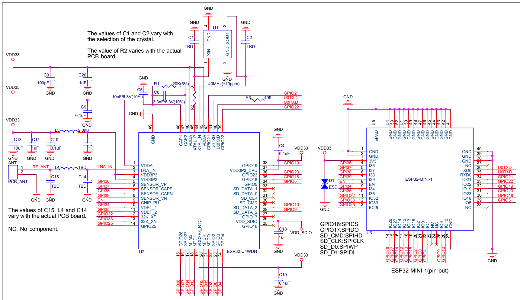
图 8: ESP32-MINI-1 原理图
