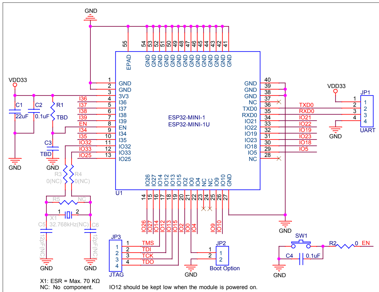
图 10: 外围设计原理图
