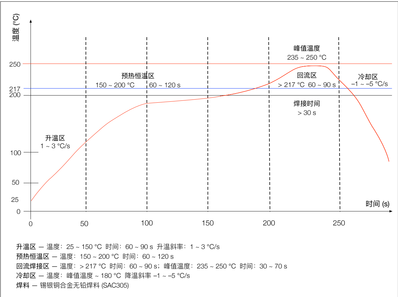
图 16: 回流焊温度曲线
