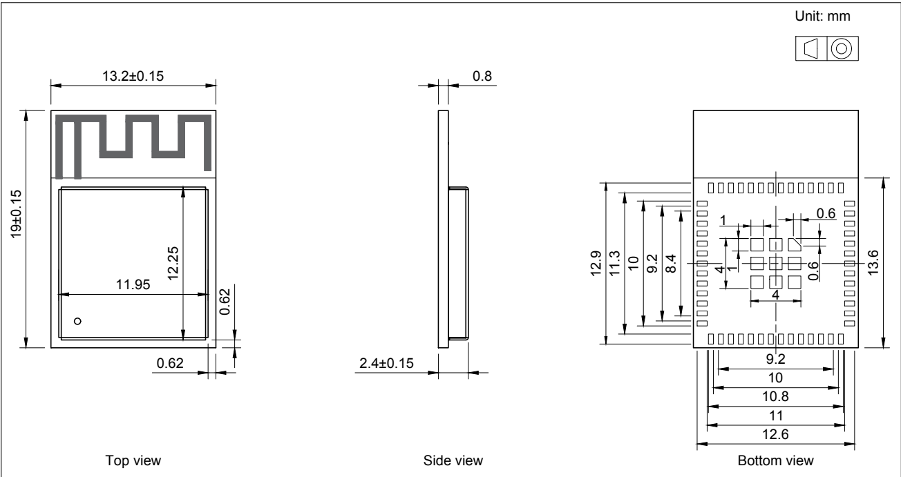
图 11: ESP32-MINI-1 模组尺寸
