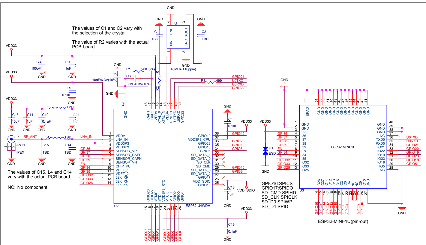
图 9: ESP32-MINI-1U 原理图
