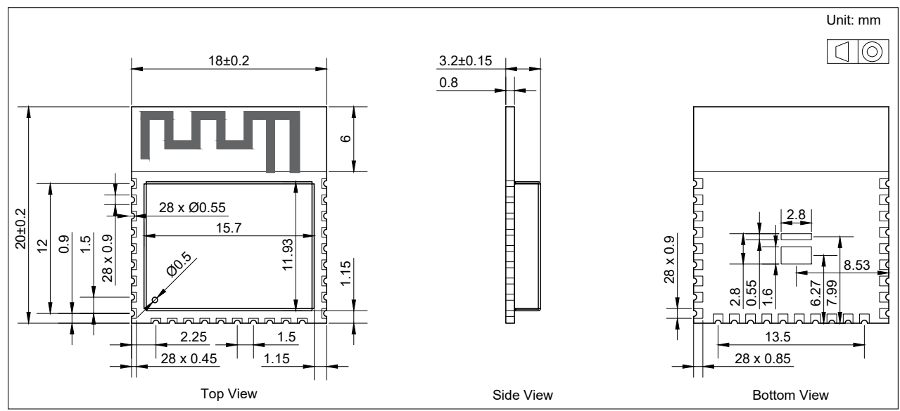
图 6: 模组尺寸
