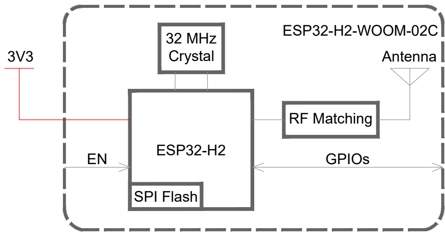
图 1: 功能框图
