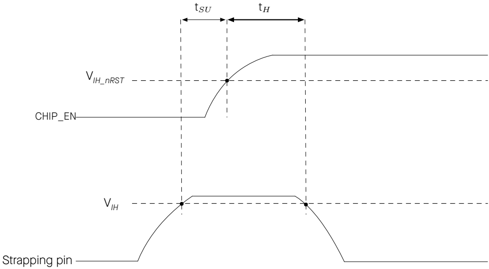
图 3: Strapping 管脚的时序参数图
