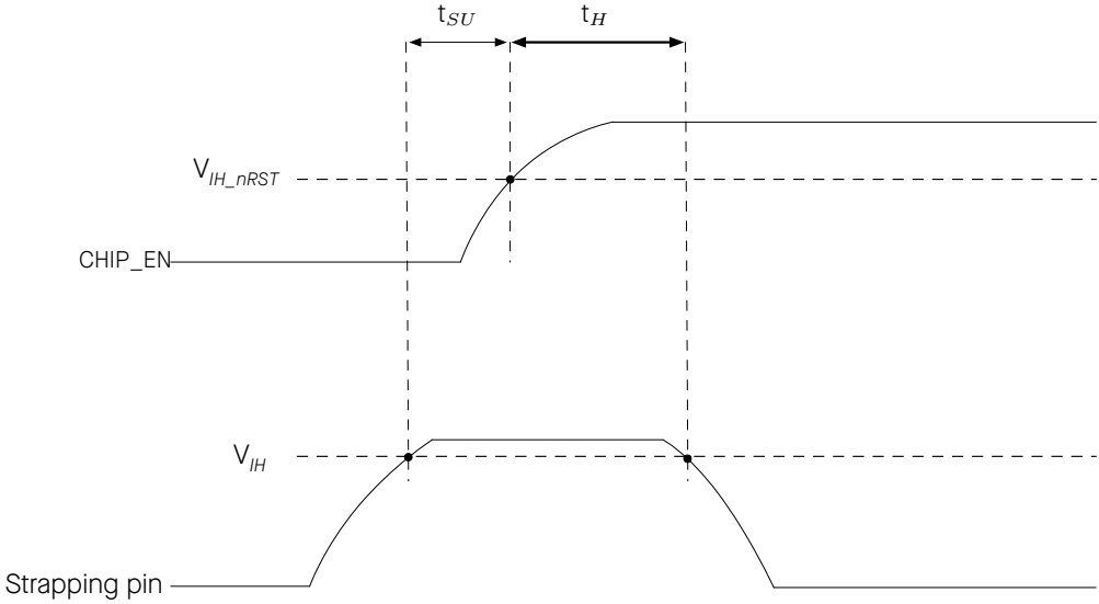
图 4: Strapping 管脚的时序参数图
