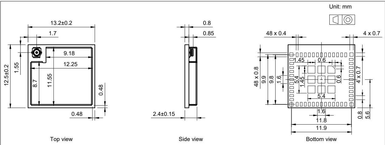
图 9: ESP32-H2-MINI-1U 尺寸
