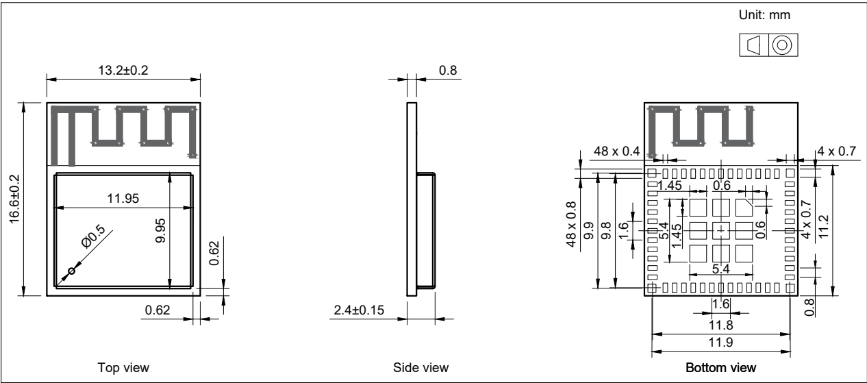
图 8: ESP32-H2-MINI-1 尺寸
