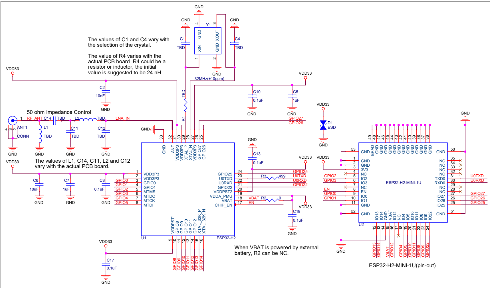
图 6: ESP32-H2-MINI-1U 原理图
