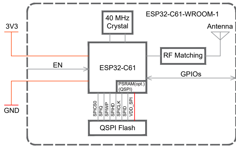
图 2: ESP32-C61-WROOM-1 功能框图
