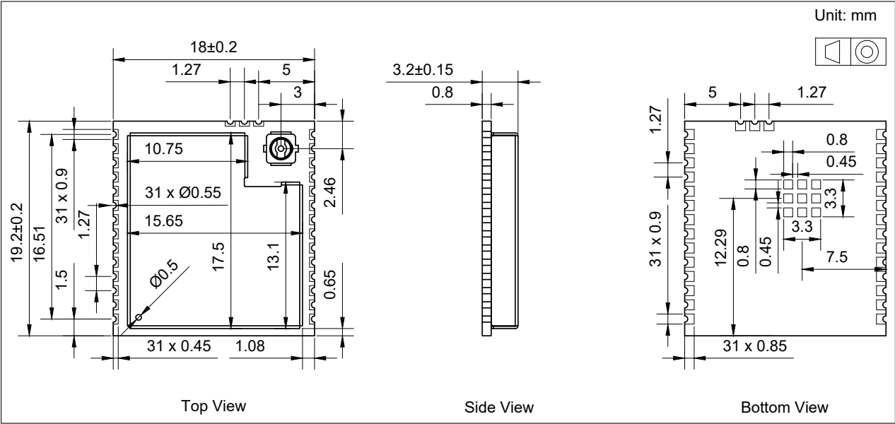
图 12: ESP32-C61-WROOM-1U 模组尺寸
