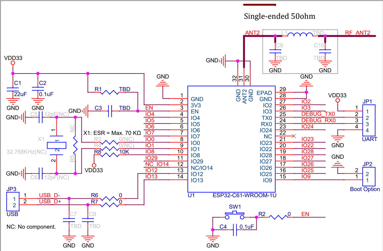
图 10: ESP32-C61-WROOM-1U 外围设计原理图
