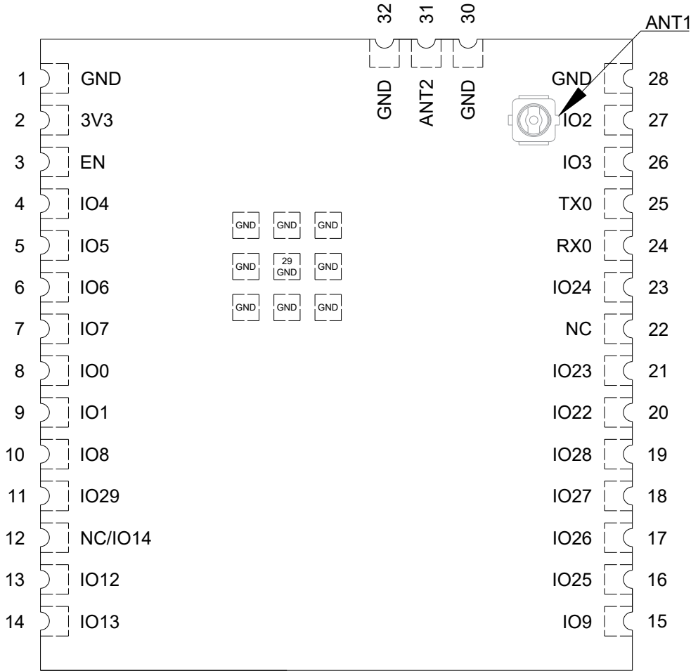
图 5: ESP32-C61-WROOM-1U 管脚布局（顶视图）
