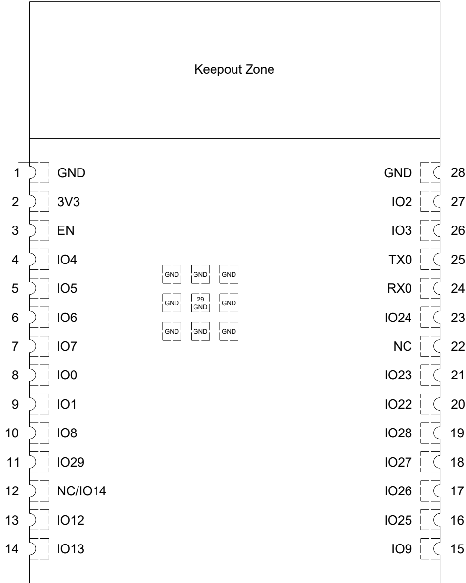
图 4: ESP32-C61-WROOM-1 管脚布局（顶视图）
