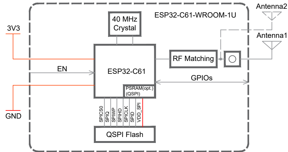
图 3: ESP32-C61-WROOM-1U 功能框图
