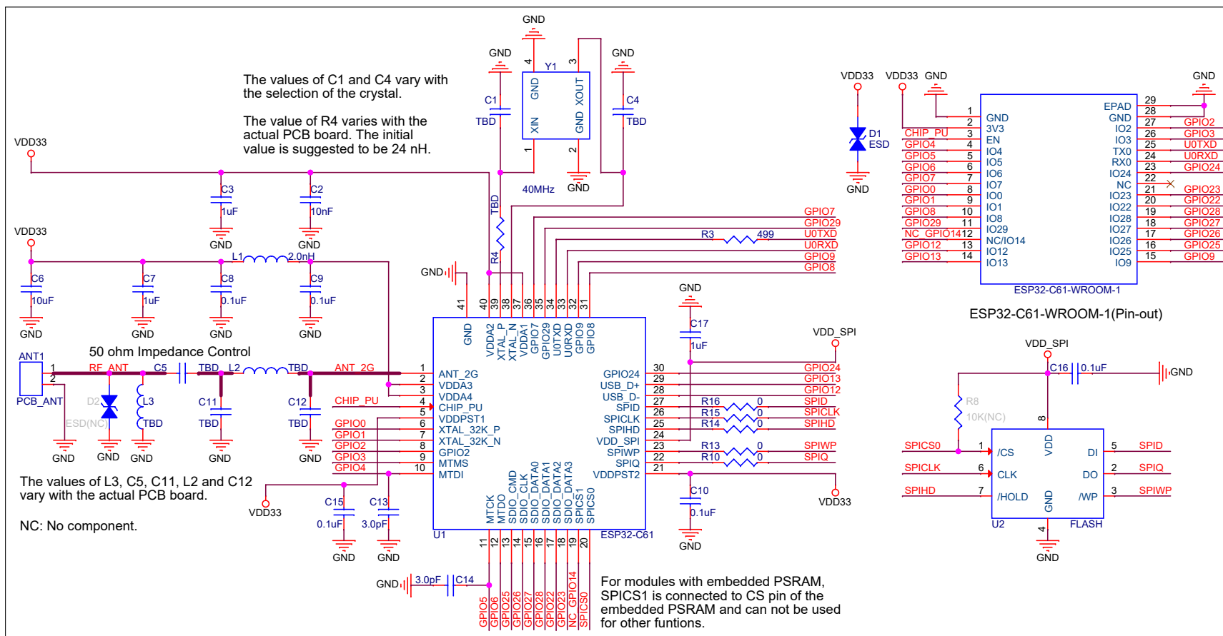
图 7: ESP32-C61-WROOM-1 原理图
