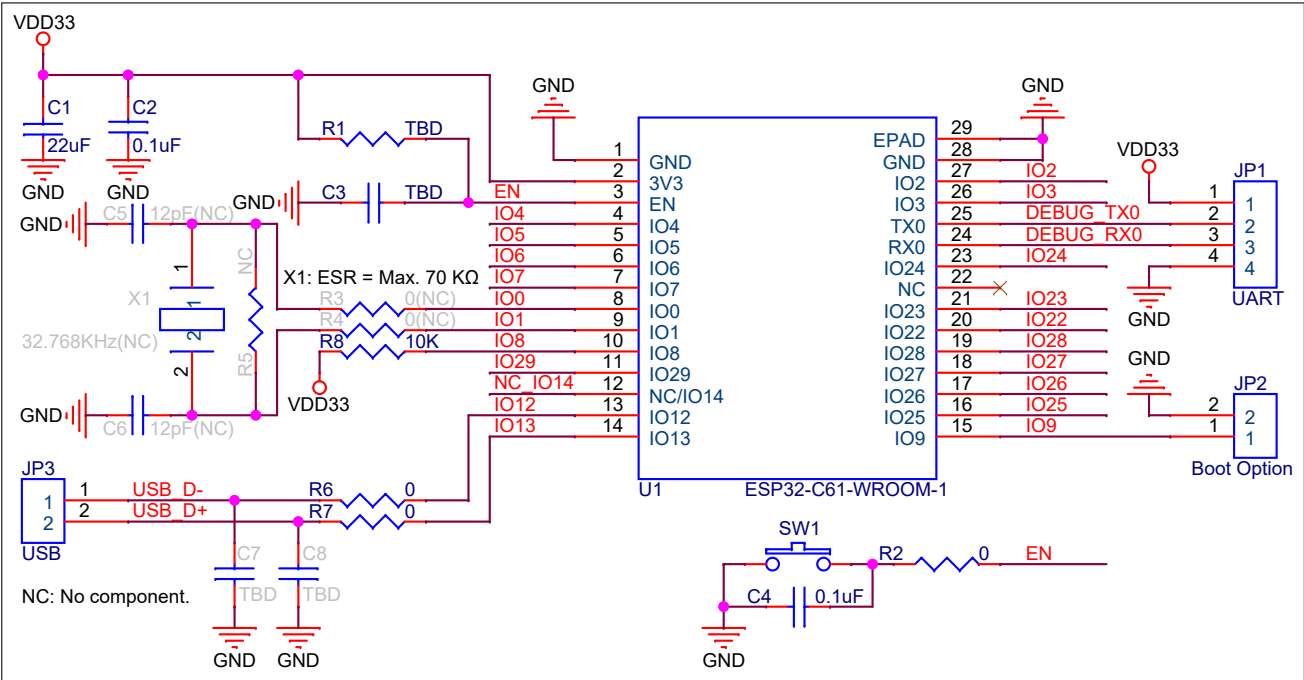
图 9: ESP32-C61-WROOM-1 外围设计原理图
