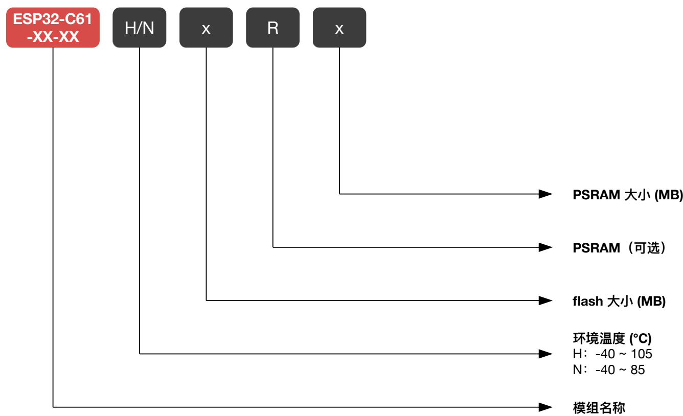
图 1: ESP32-C61 模组型号命名规则
