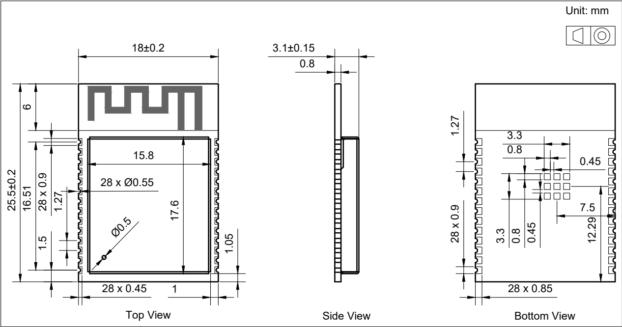
图 11: ESP32-C61-WROOM-1 模组尺寸
