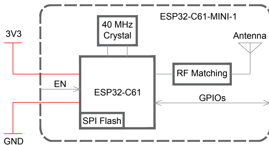
图 2: ESP32-C61-MINI-1 功能框图
