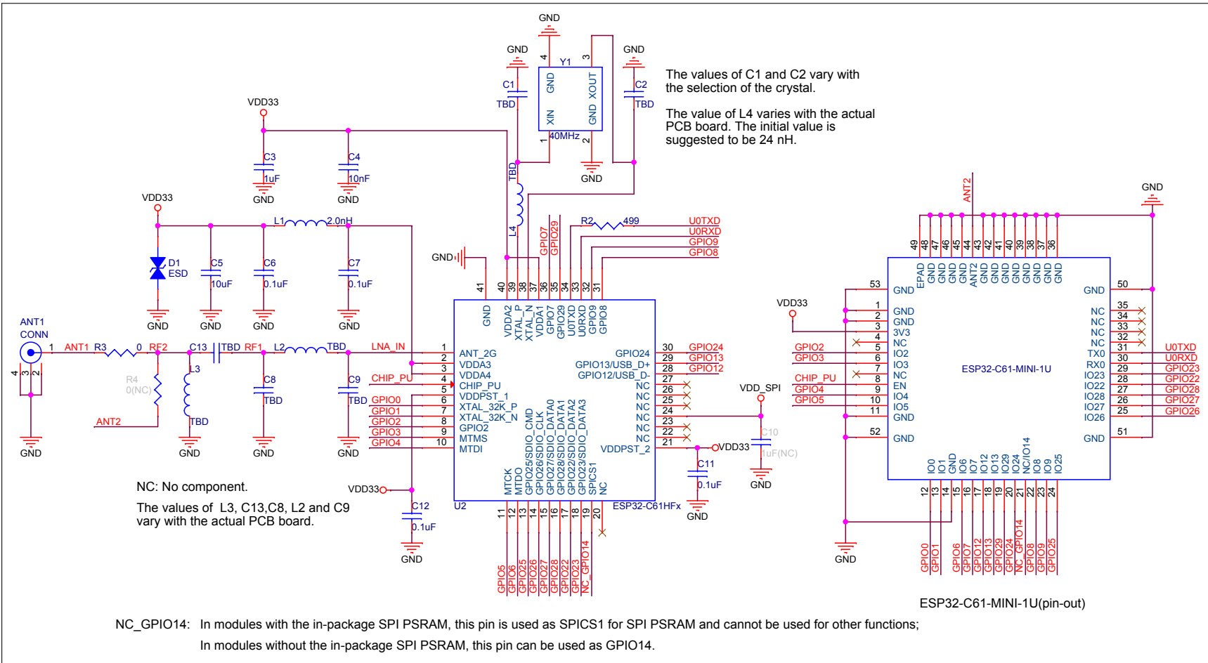
图 8: ESP32-C61-MINI-1U 原理图
