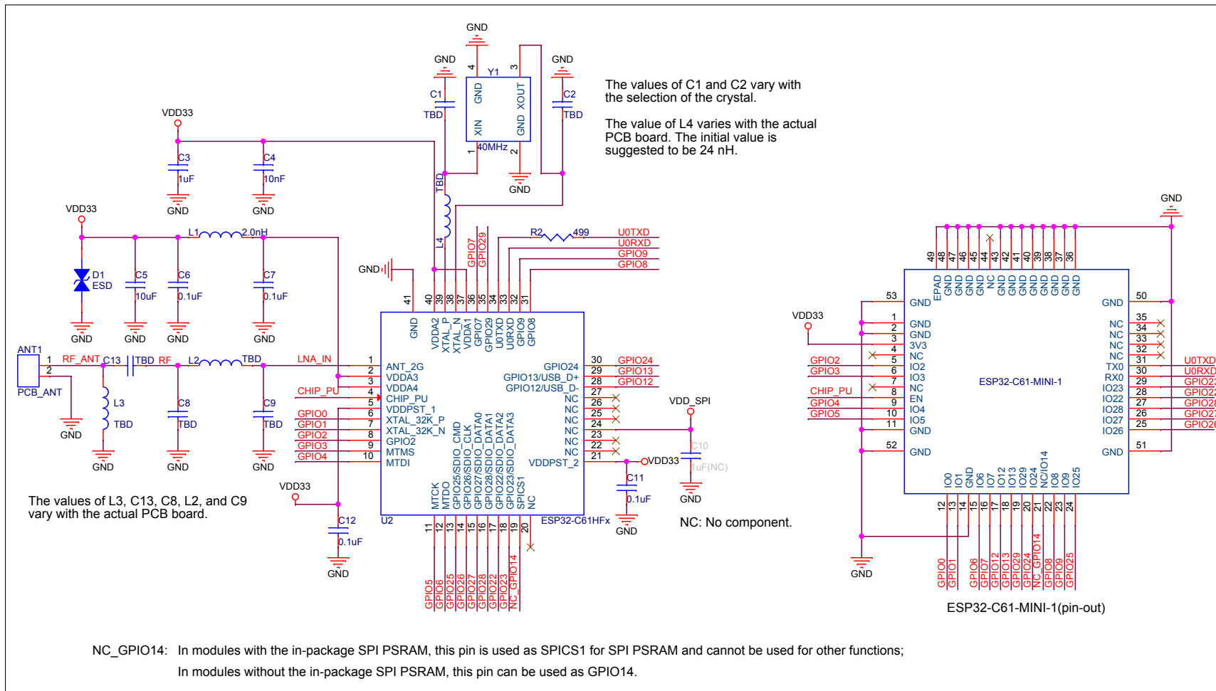
图 7: ESP32-C61-MINI-1 原理图
