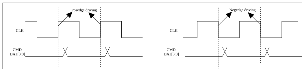
图 39.5-9. 输出时序图
