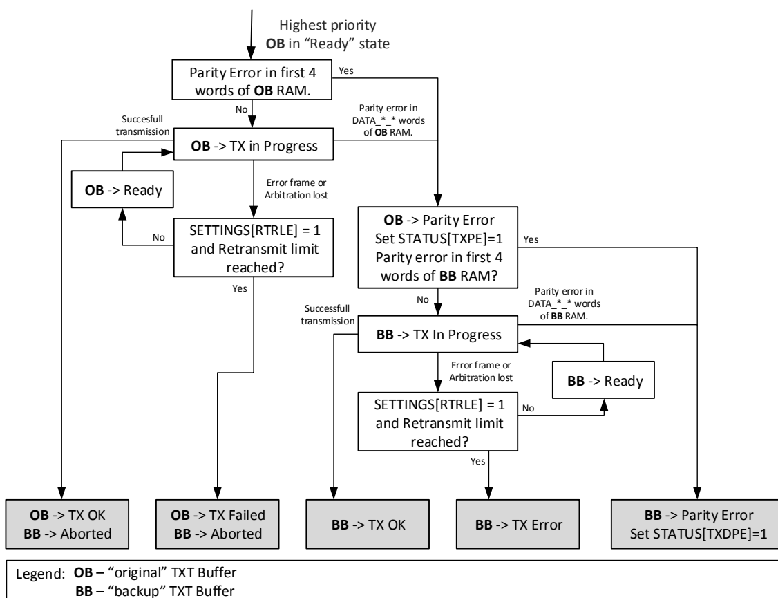
图 38.3-16. TX buffer 备份模式工作流程
