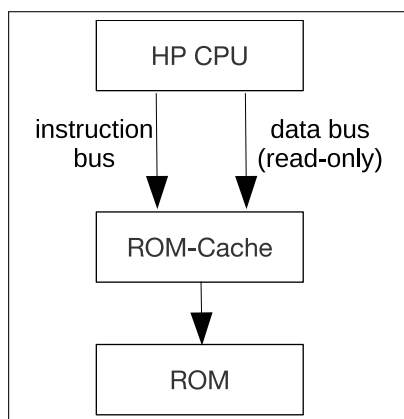
图 6.3-2. ROM-Cache 系统结构
