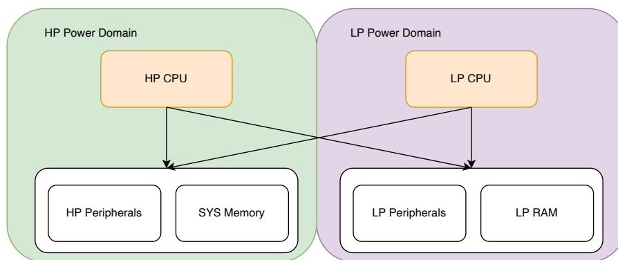
图 4.0-1. LP CPU 概览
