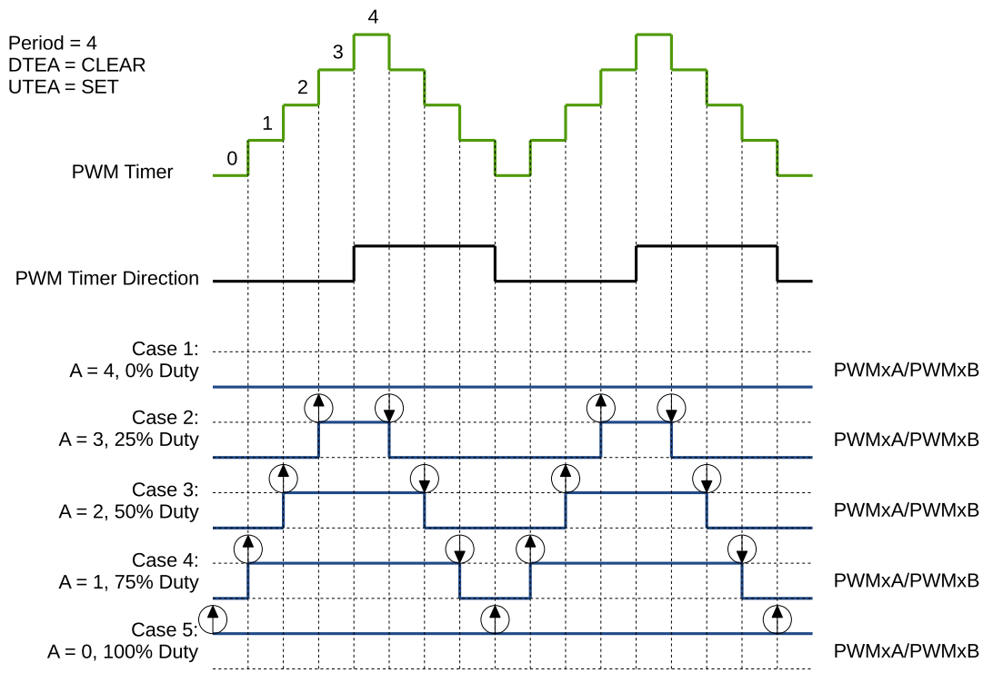
图 41.3-13. 递增递减模式下的对称波形
