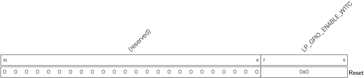
Register 8.48. LP_GPIO_ENABLE_W1TC_REG (0x0018)
