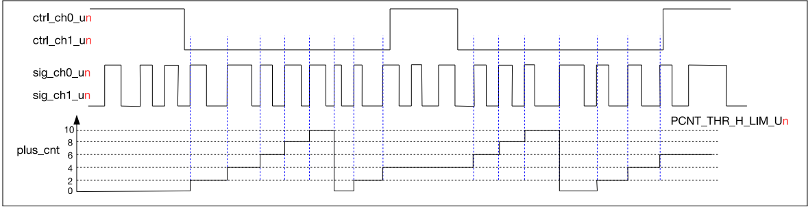
图 36.3-3. 双通道递增计数图
