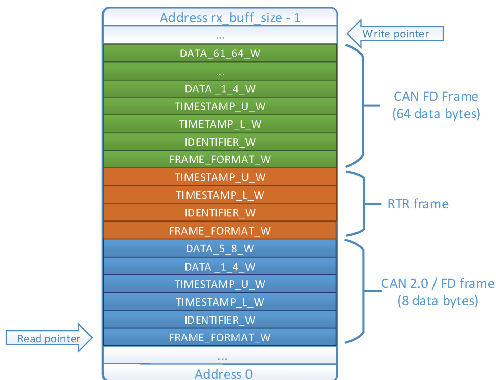
图 38.3-12. RX buffer
