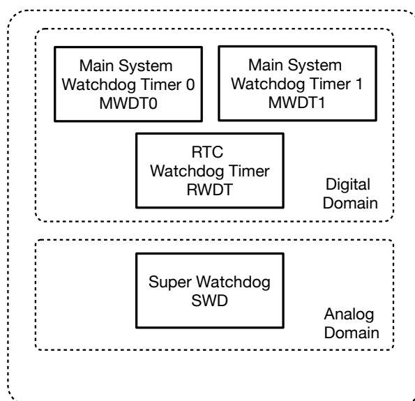
图 16.1-1. 看门狗定时器概览
