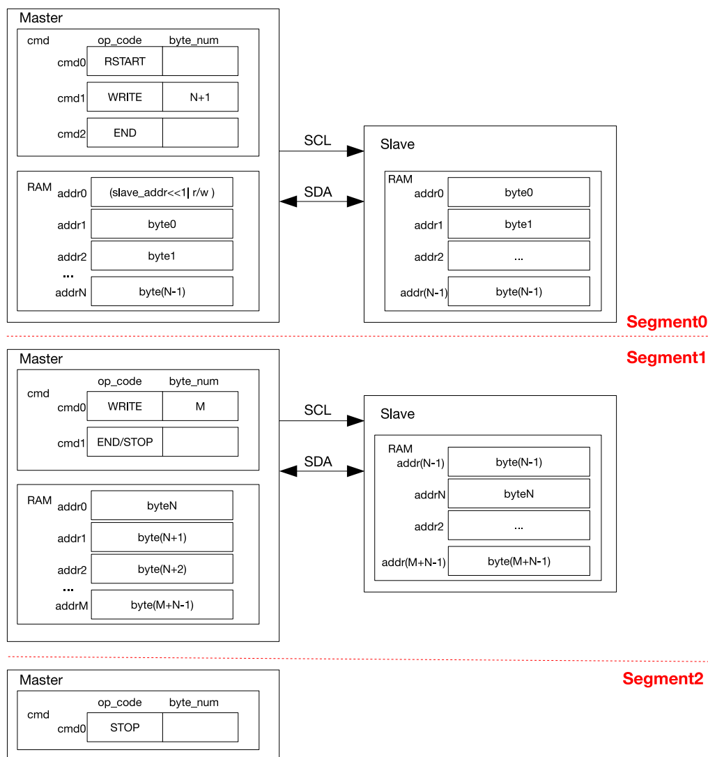
图 34.7-4. I2C 主机分段写 7 位寻址的从机
