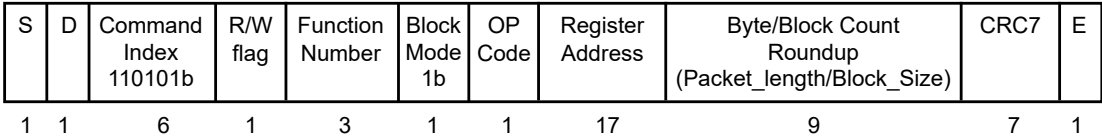
图 39.5-2. CMD53 内容
