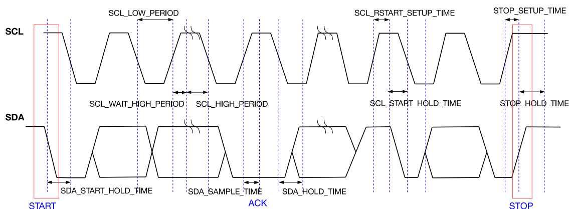
图 34.4-1. I2C 时序图
