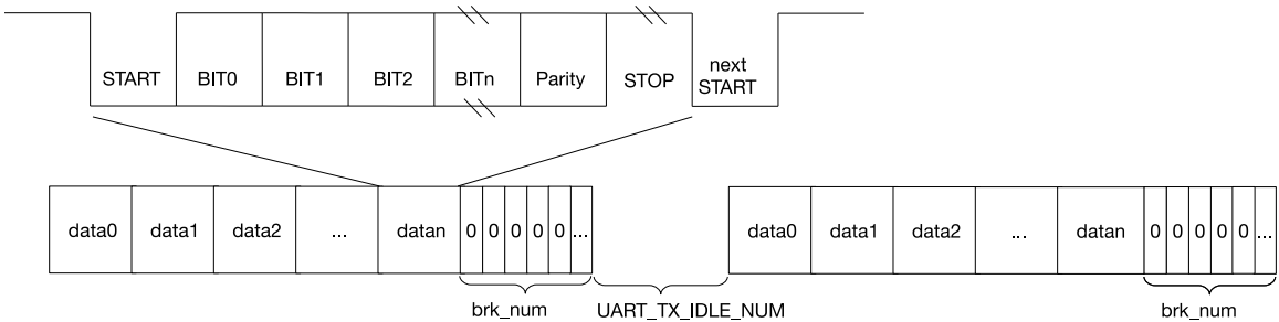
图 32.4-3. UART 数据帧结构
