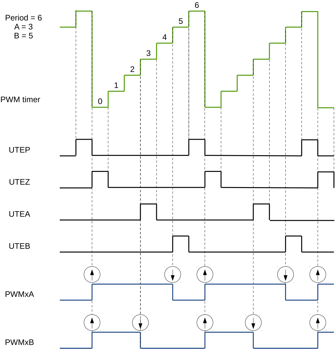
图 41.3-14 至图 41.3-17 的 PWM 波形描述了常见的 PWM 生成器配置。
