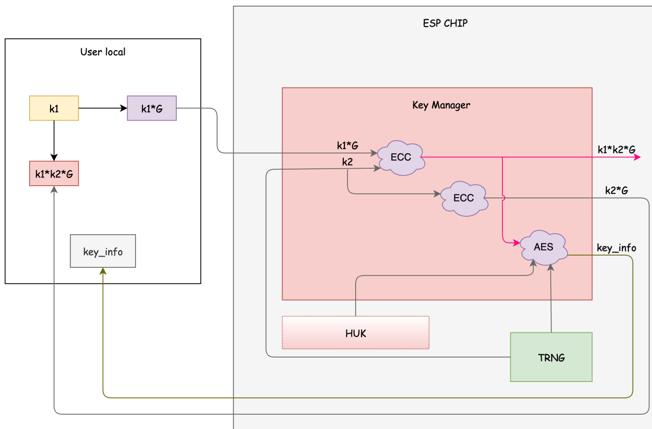
图 31.6-2. ECDHO 部署模式
