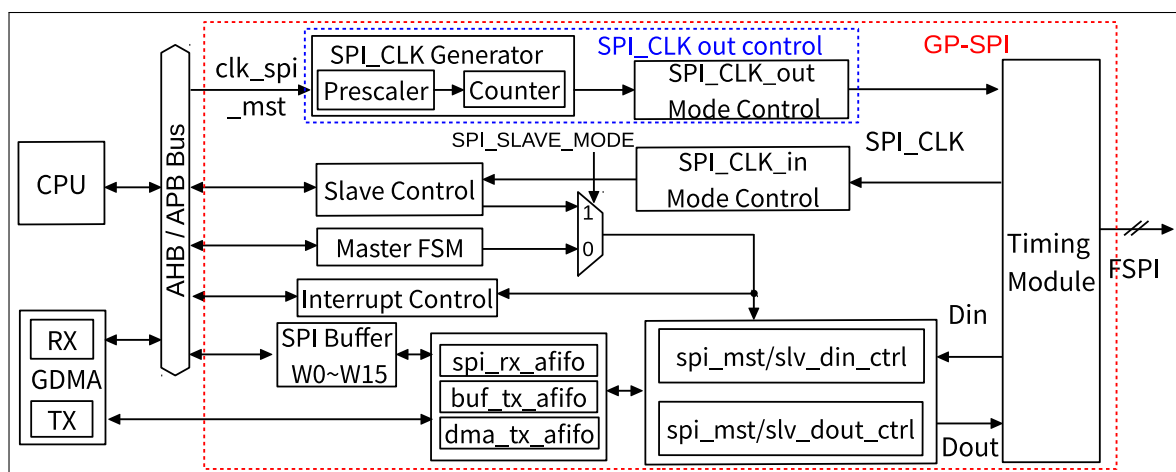
图 33.5-2. GP-SPI2 功能块图
