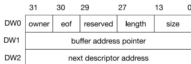
图 39.5-5. SDIO 从机 DMA 链表描述符结构
