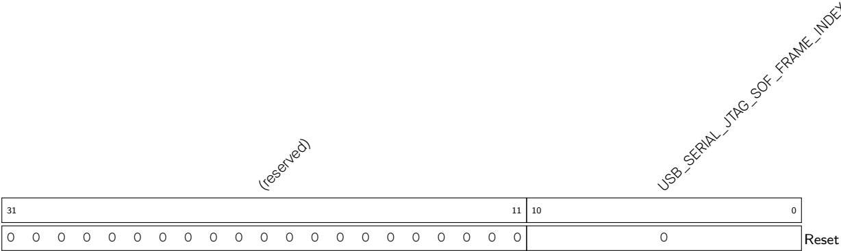
Register 37.19. USB_SERIAL_JTAG_FRAM_NUM_REG (0x0024)
