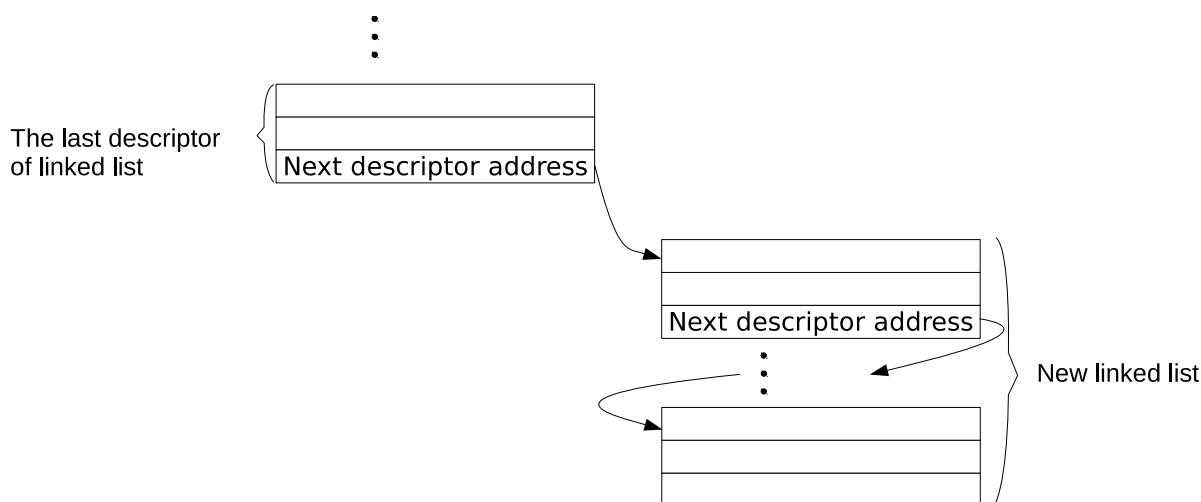
图 5.4-2. 链表关系图
