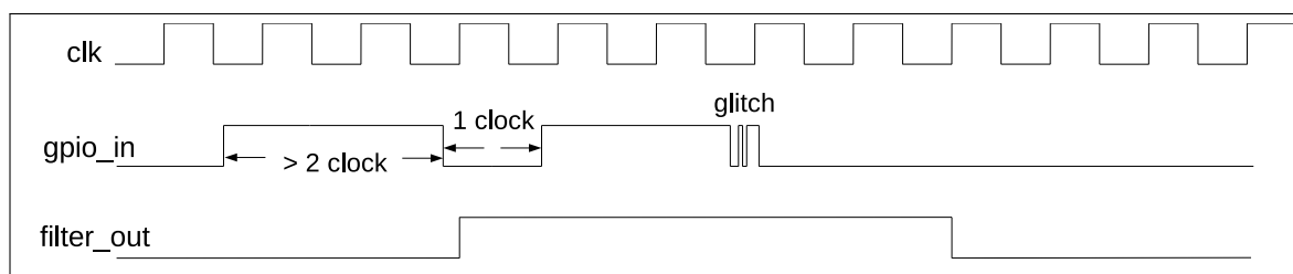
图 8.4-2. GPIO 输入信号滤波时序图
