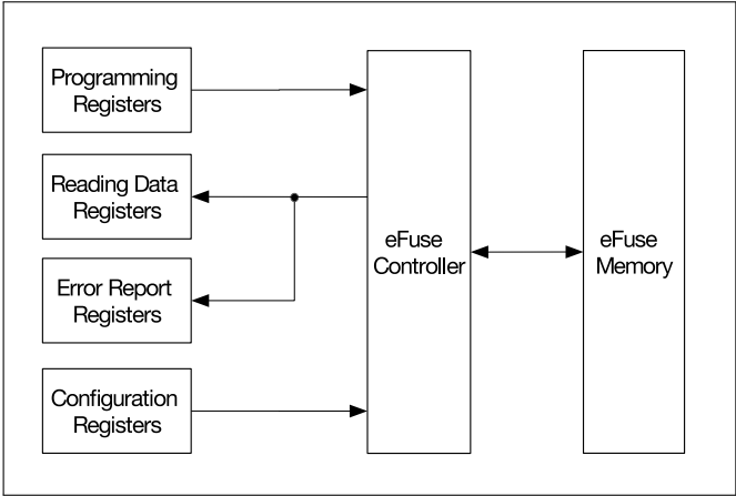
图 7.3-1. eFuse 系统数据通路
