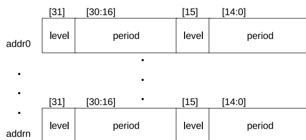
图 42.3-2. RAM 中脉冲编码结构
