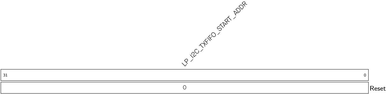
Register 34.67. LP_I2C_TXFIFO_START_ADDR_REG (0x0100)
