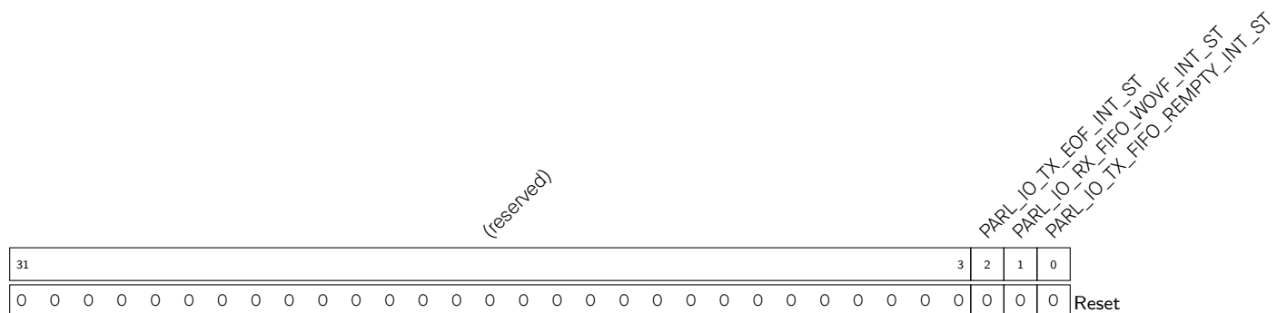
Register 43.13. PARL_IO_INT_ST_REG (0x0030)
