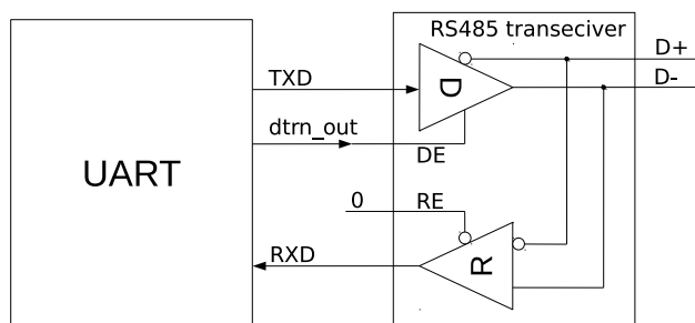
图 32.4-5. RS485 模式驱动控制结构图
