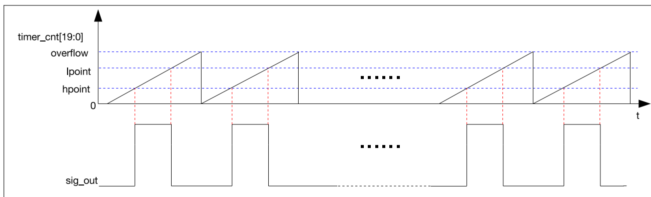
图 40.4-3. LED PWM 输出信号图
