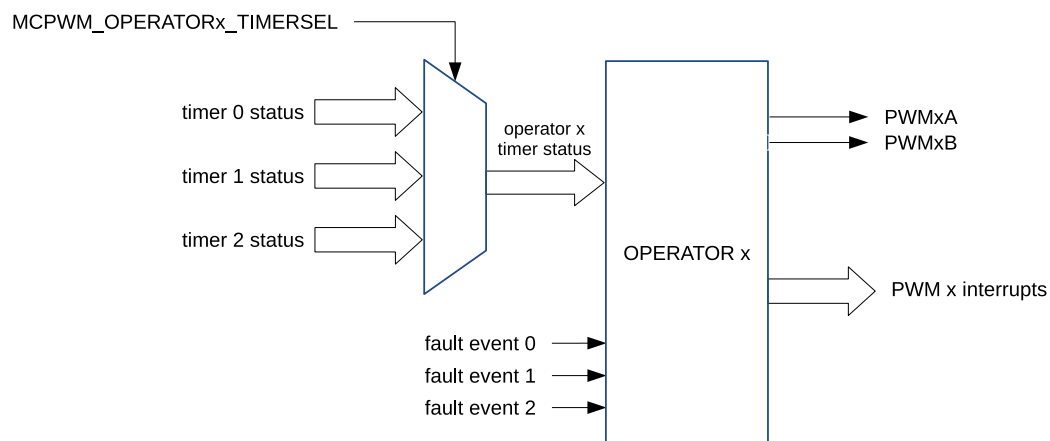
图 41.3-2. 操作器模块
