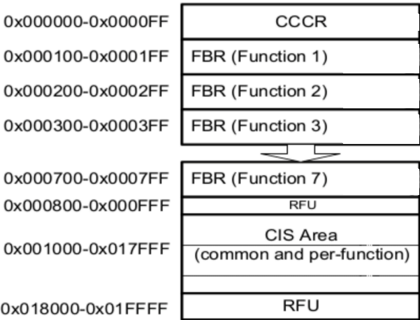
图 39.5-3. function 0 地址空间
