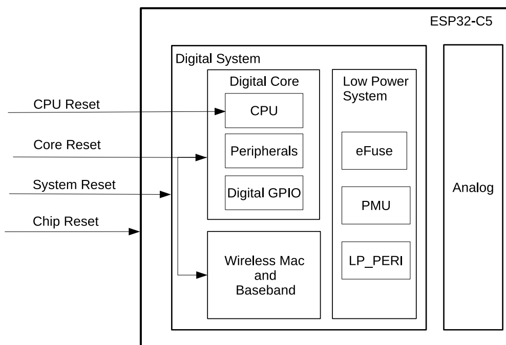
图 9.1-1. 四种复位等级
