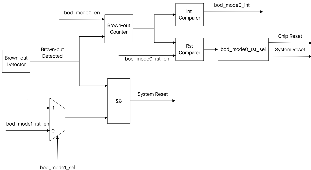
图 21.3-2. 欠压检测器处理方式
