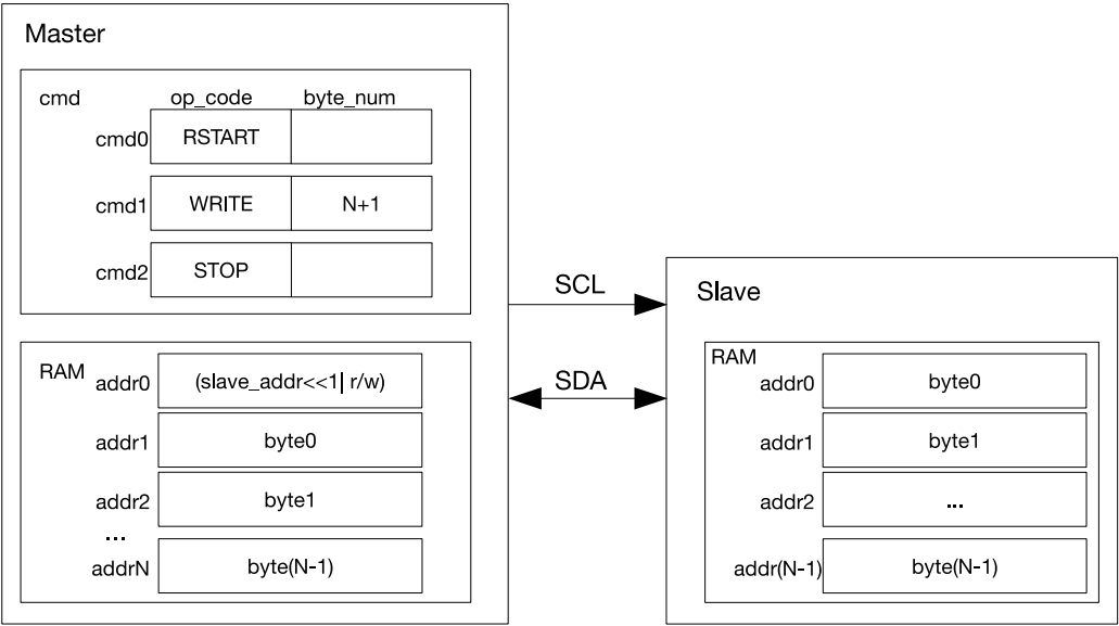
图 34.7-1. I2C 主机写 7 位寻址的从机
