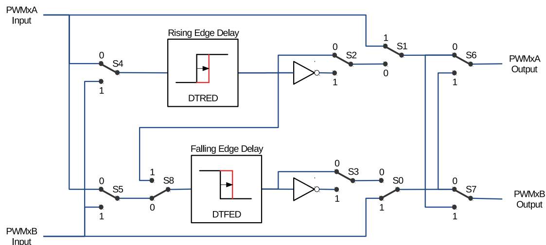
图 41.3-21. 死区模块的开关拓扑
