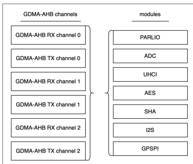
图 5.1-1. 共用 GDMA 通道的模块
