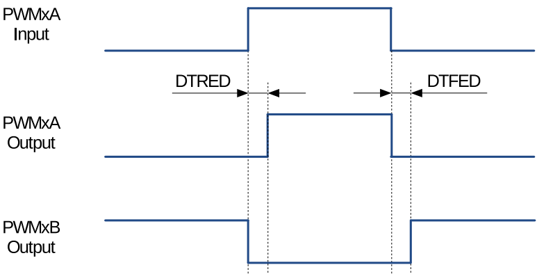
图 41.3-22. 高电平有效互补 (AHC) 死区波形
