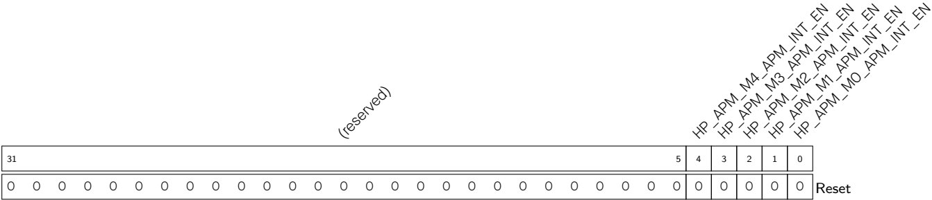
Register 18.26. HP_APM_INT_EN_REG (0x0118)
