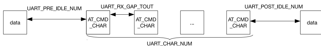
图 32.4-4. AT_CMD 字符格式
