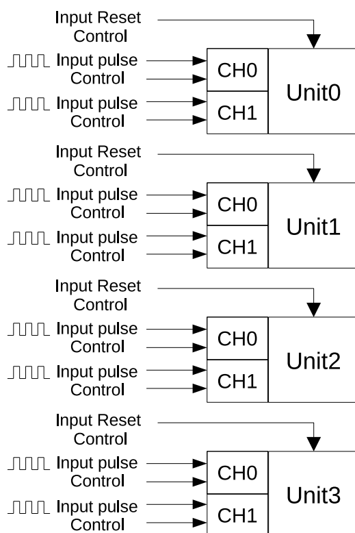
图 36.0-1. PCNT 框图
