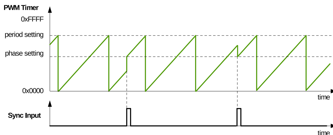
图 41.3-5. 递增计数模式波形
