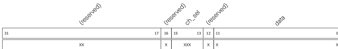
图 46.5-8. GDMA 数据格式
