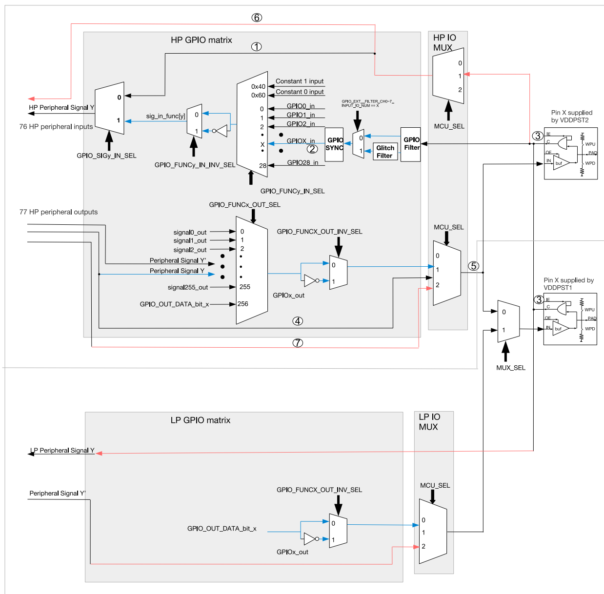
图 8.3-1. HP GPIO 交换矩阵、HP IO MUX、LP GPIO 交换矩阵和 LP IO MUX 框图
