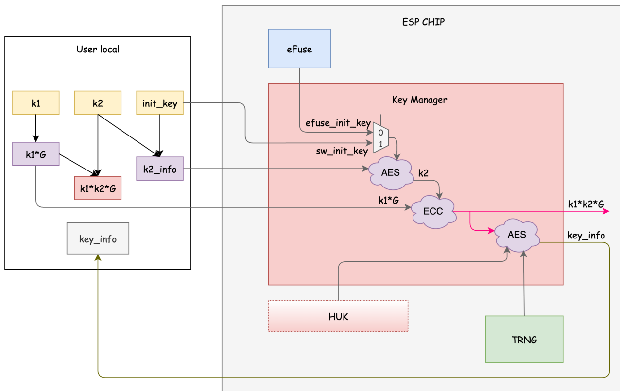
图 31.6-3. ECDH1 部署模式
