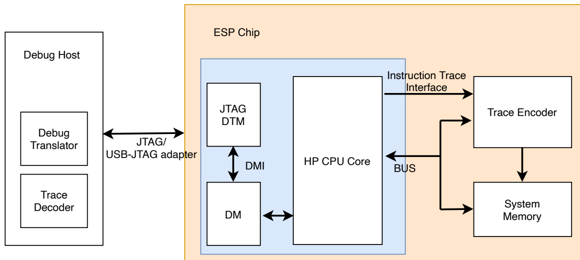
图 3.2-1. 指令追踪流程概览
