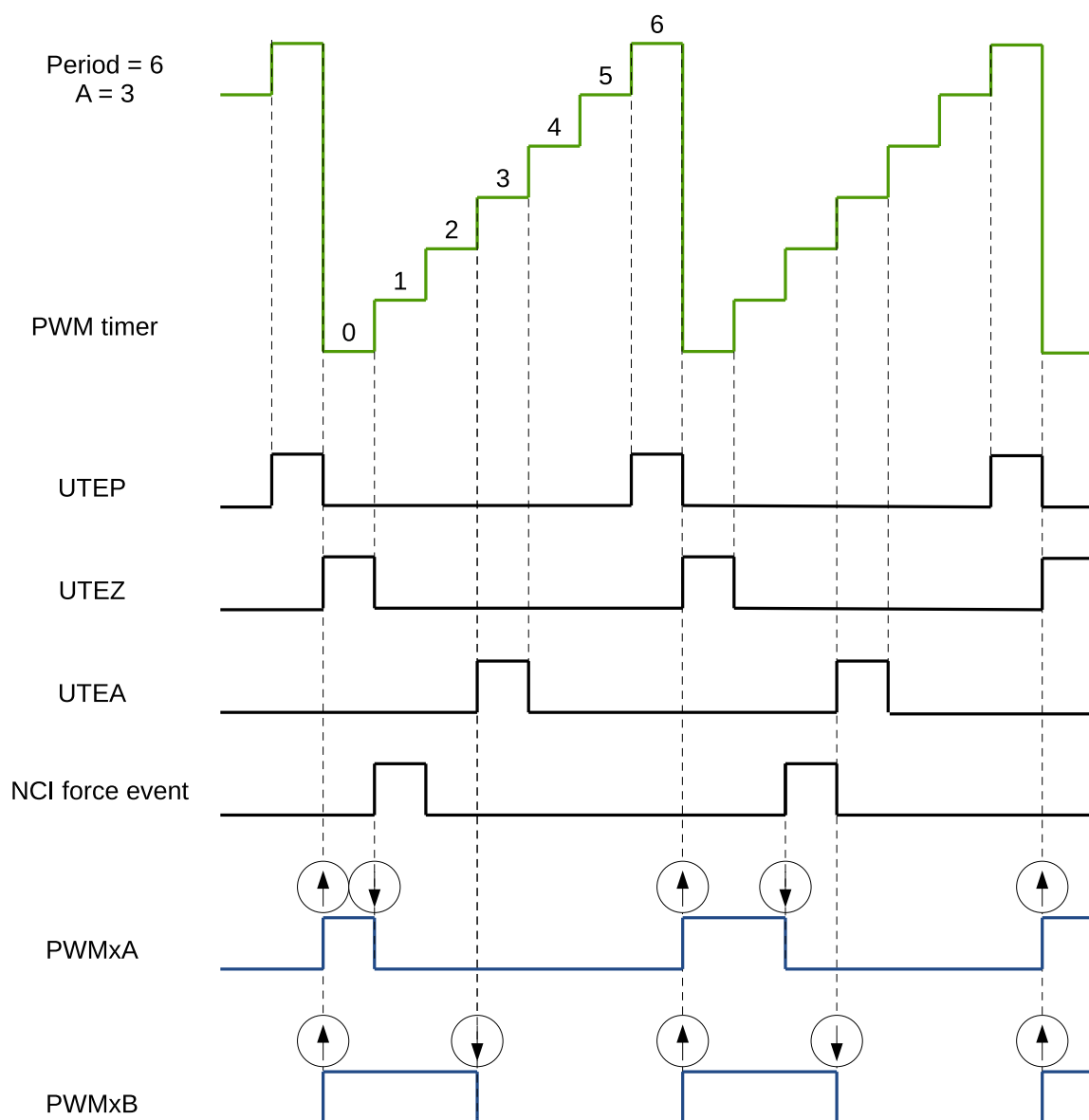
图 41.3-19. NCI 在 PWMxA 输出上软件强制事件示例
