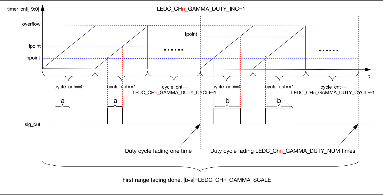
图 40.4-4. 输出信号占空比线性渐变图
