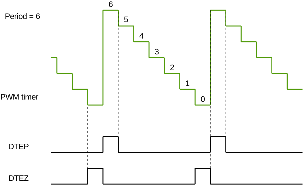
图 41.3-10. 递减模式中生成的 DTEP 和 DTEZ
