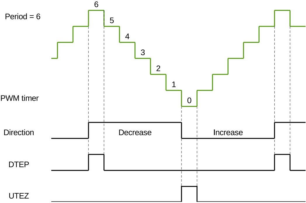
图 41.3-11. 递增递减模式中生成的 DTEP 和 UTEZ
