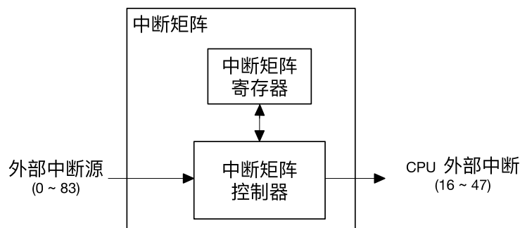
图 11.4-1. 中断矩阵结构图
