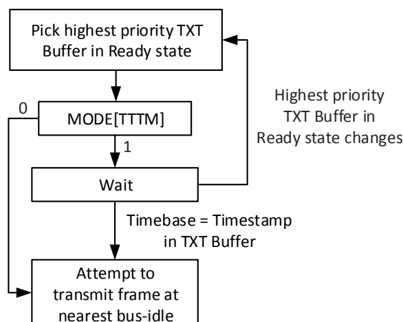
图 38.3-9. TX buffer 选择
