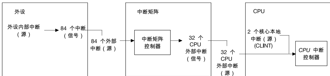
图 11.2-1. ESP32-C5 的中断流
