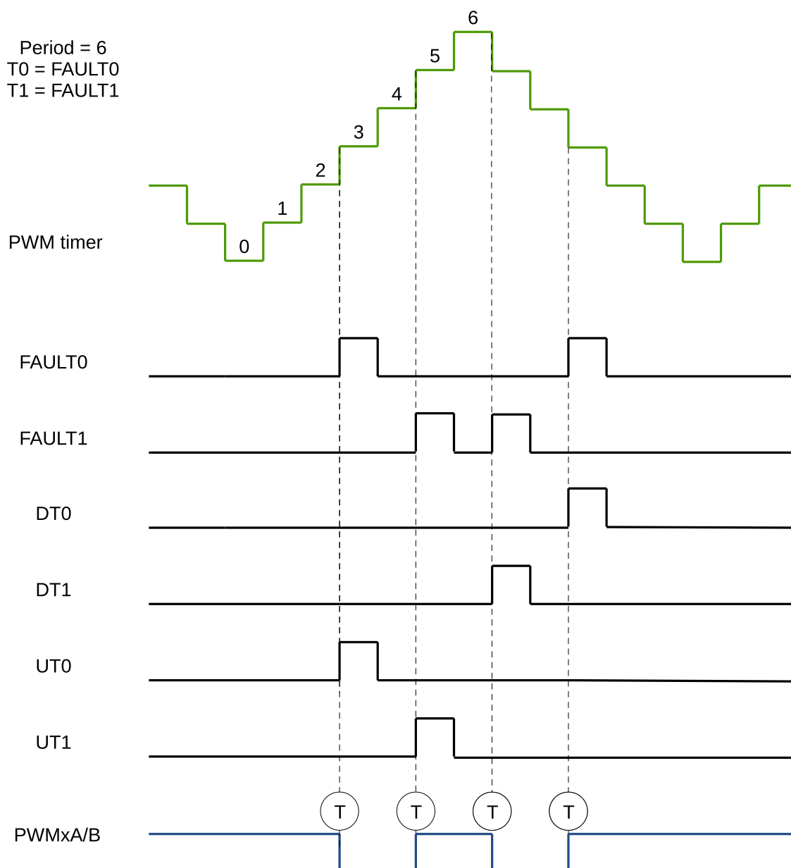
图 41.3-18. 递增递减循环计数模式，错误或同步事件，在 PWMxA 和 PWMxB 上相同调制
