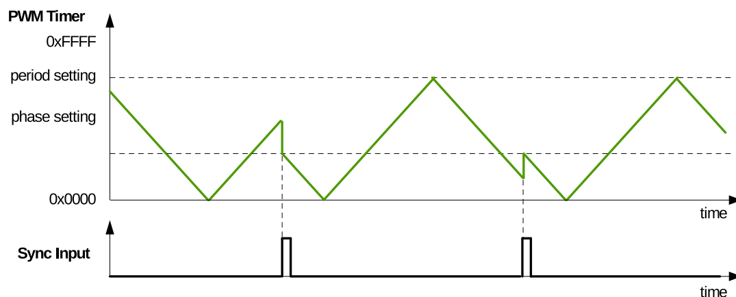
图 41.3-7. 递增递减循环模式波形，同步事件后递减
