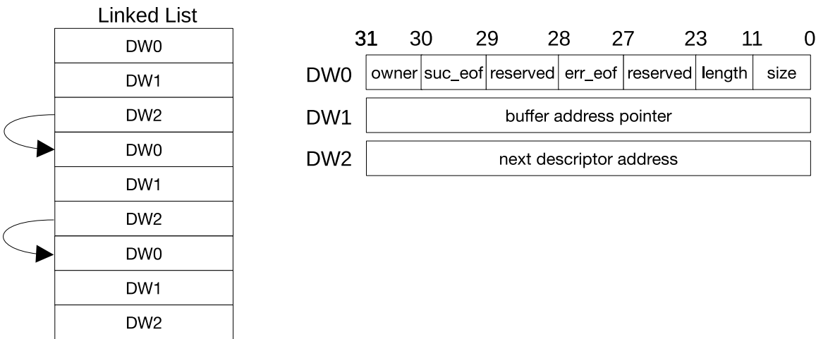
图 5.4-1. 链表结构图
