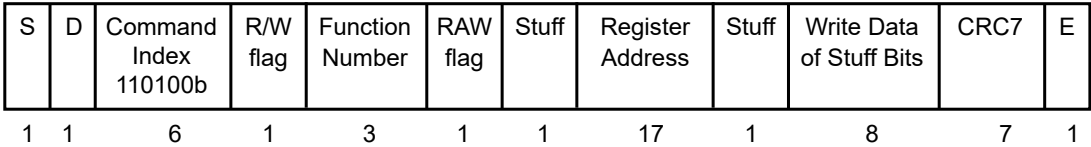
图 39.5-1. CMD52 内容
