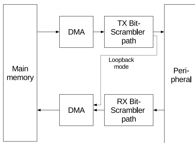
图 44.1-1. 比特调节器系统架构图
