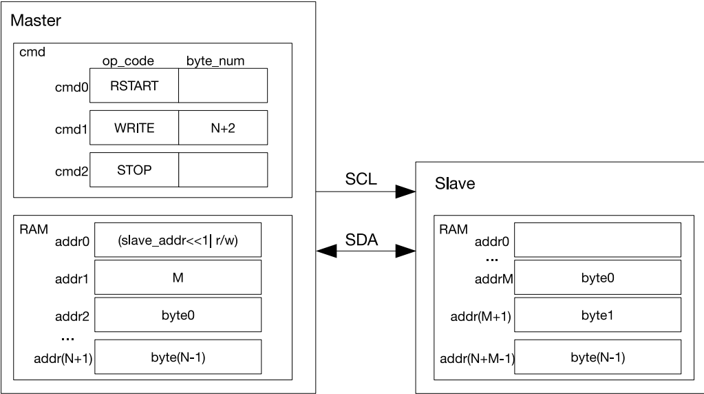
图 34.7-3. I2C 主机写 7 位双地址寻址从机
