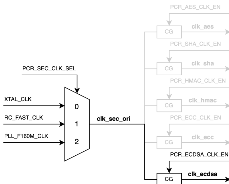
图 28.5-2. clk_ecdsa 时钟图
