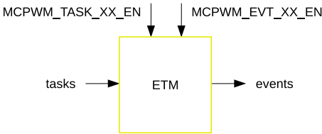
图 41.3-4. ETM 模块
