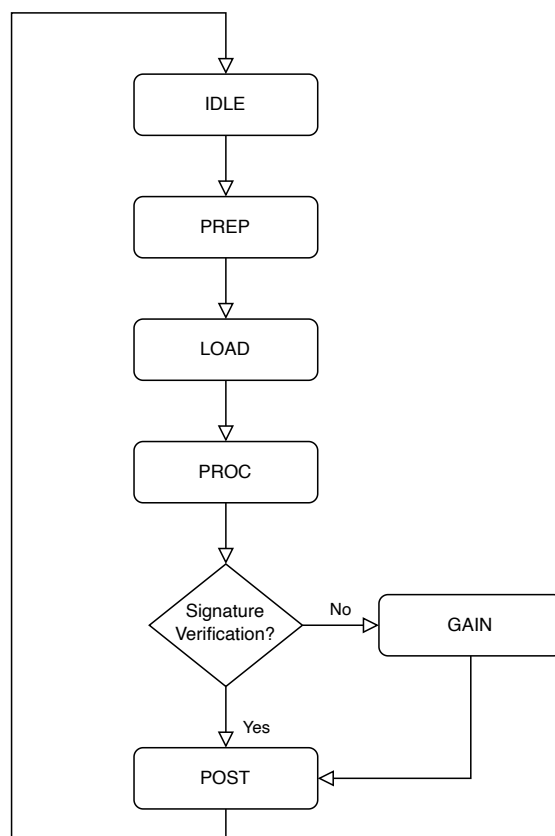
图 28.5-1. ECDSA 流程
