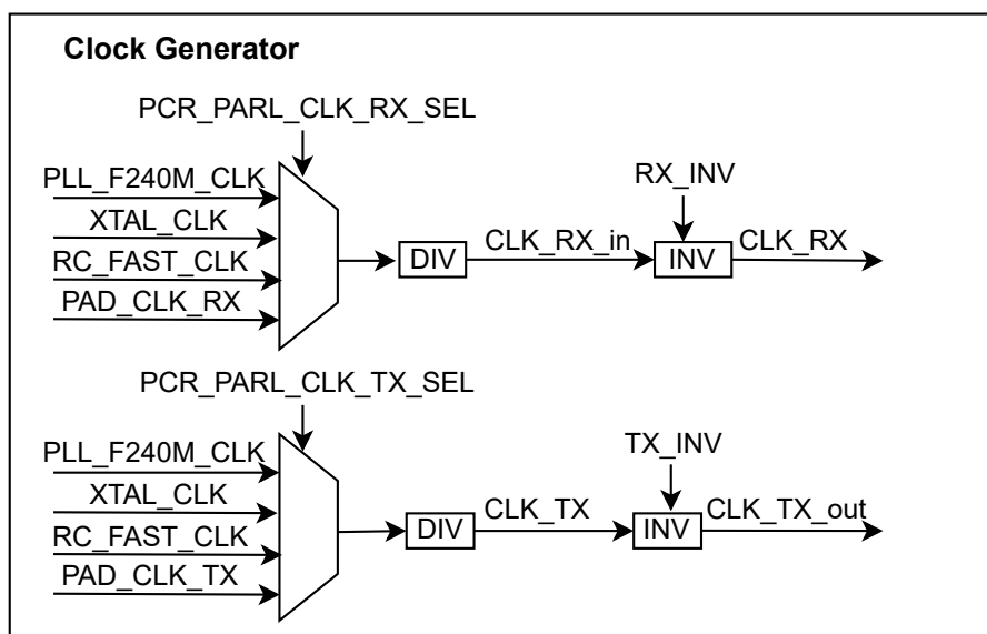
图 43.5-1. PARLIO 时钟生成
