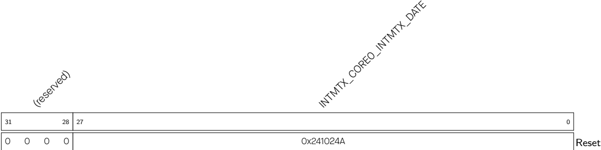
Register 11.80. INTMTX_CORE0_INTMTX_DATE_REG (0x07FC)
