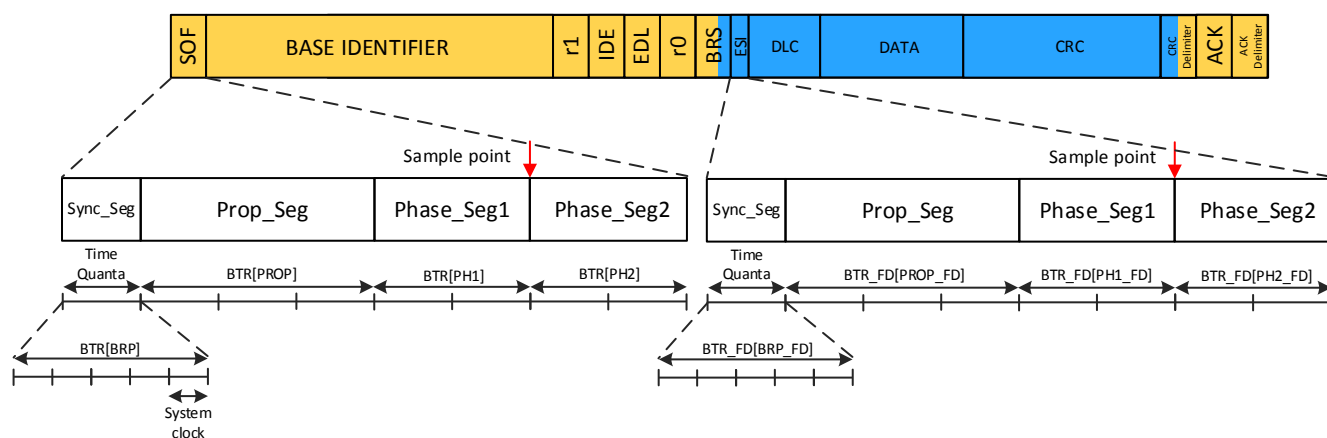
图 38.3-3. 位时间
