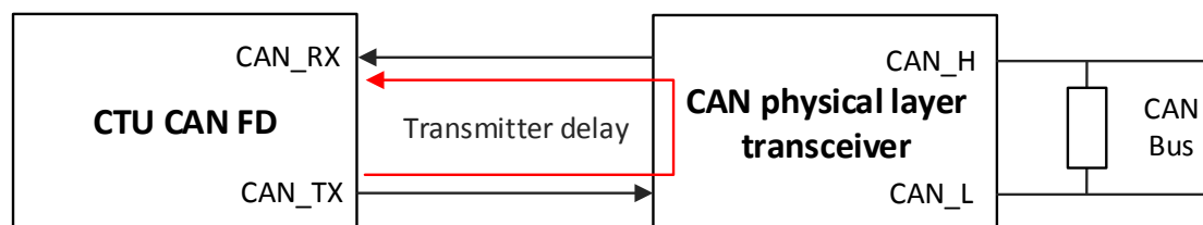
图 38.3-4. 发送器延迟
