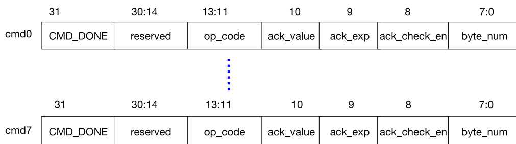
图 34.4-2. I2C 命令寄存器结构
