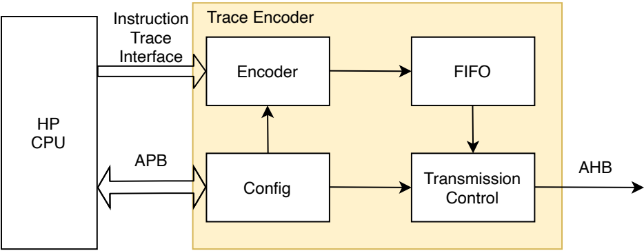
图 3.0-1. 追踪编码器概述图
