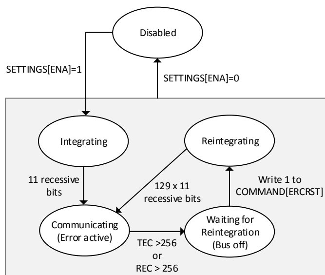
图 38.3-2. 工作模式
