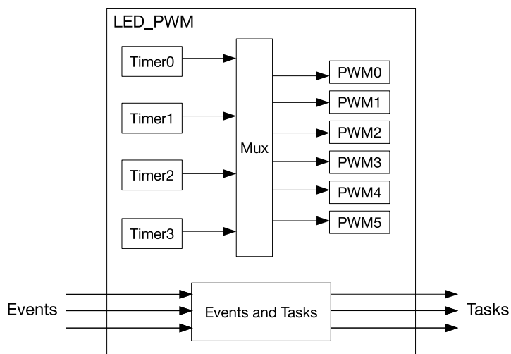
图 40.3-1. LED PWM 控制器架构
