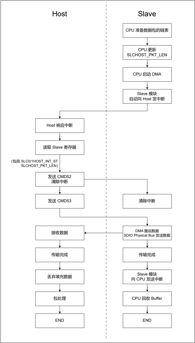
图 39.7-1. 从机向主机发送包的流程
