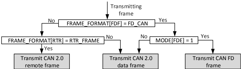
图 38.3-11. TX 帧类型
