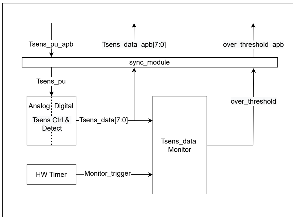
图 45.3-1. 温度传感器结构框图
