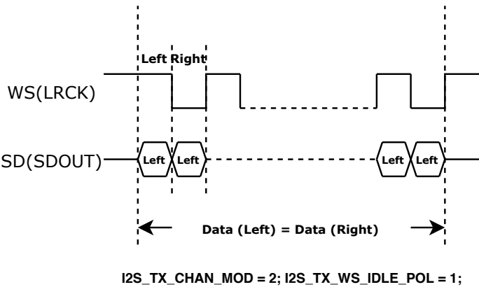
图 35.9-3. PDM 通道控制
