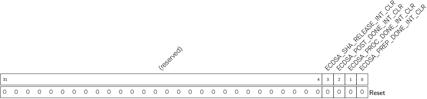
Register 28.7. ECDSA_INT_CLR_REG (0x0018)
