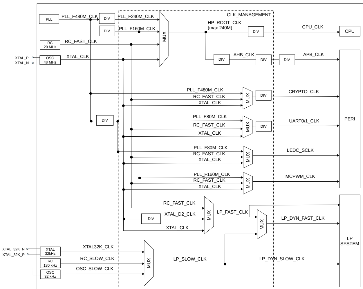
图 9.2-1. 系统时钟
