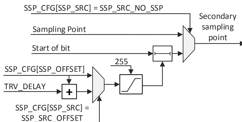
图 38.3-6. 二次采样点
