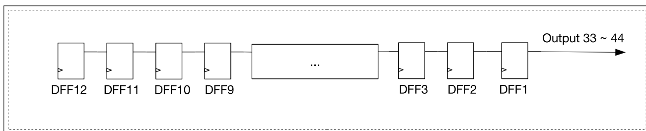
图 7.3-3. 移位寄存器电路图 (后 12 字节)
