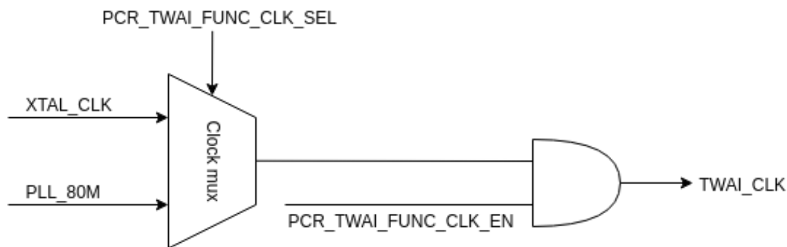
图 38.3-1. TWAI_CLK Diagram
