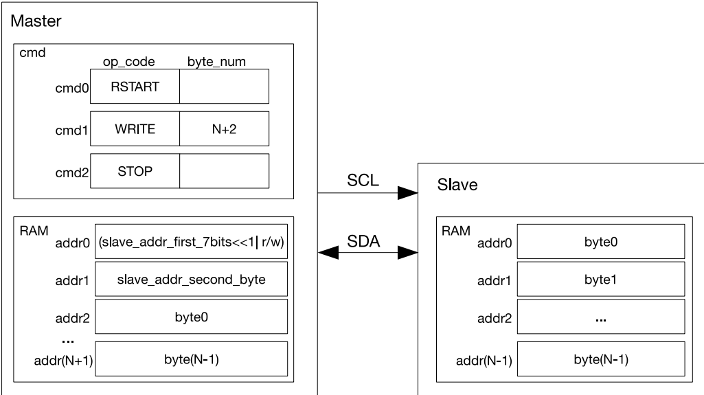
图 34.7-2. I2C 主机写 10 位寻址的从机
