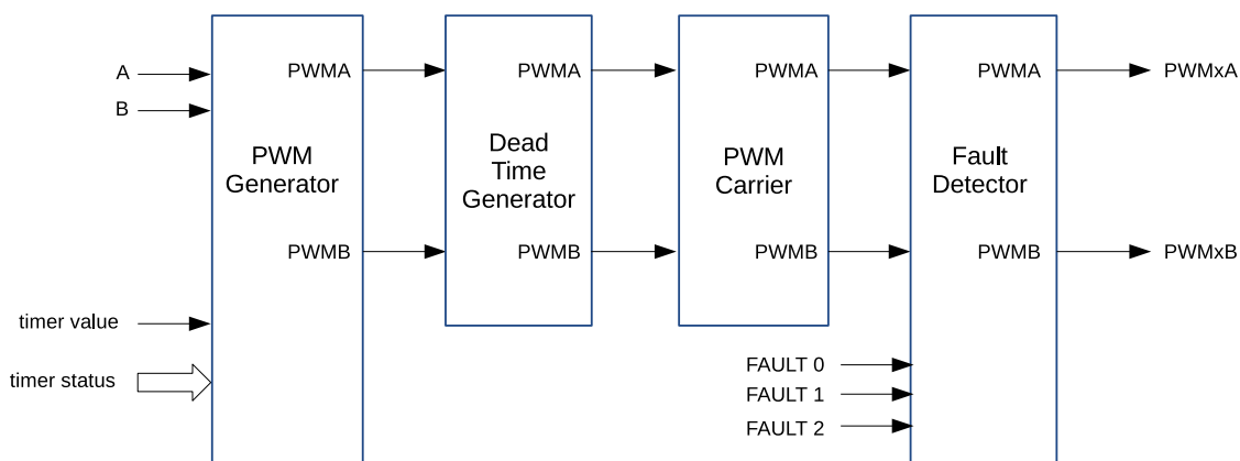
图 41.3-12. PWM 操作器的子模块
