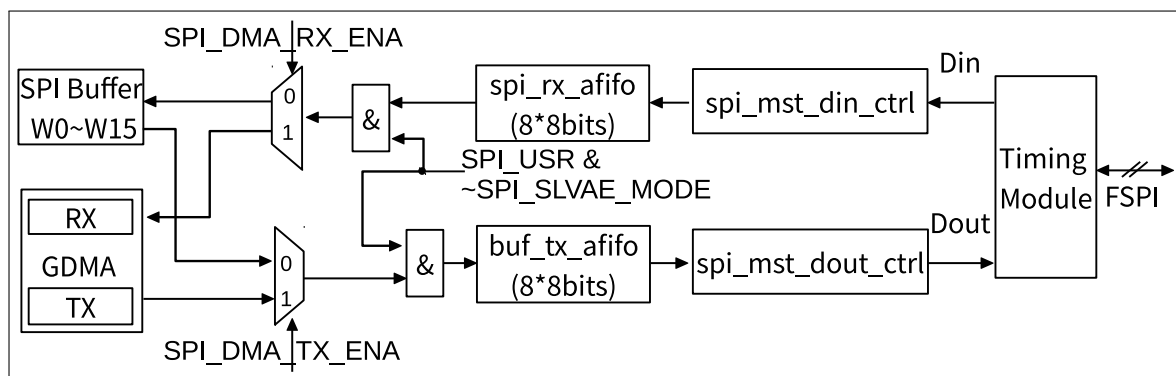
图 33.5-3. GP-SPI2 用作主机时的数据流控制
