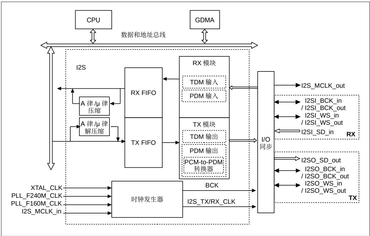
图 35.4-1. ESP32-C5 I2S 系统框图
