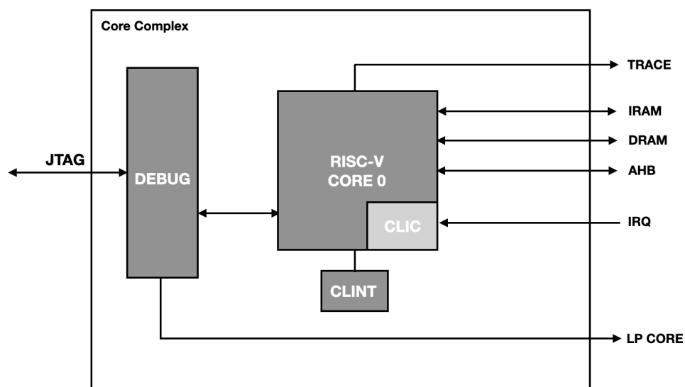
图 2.1-1. CPU 核心系统框图
