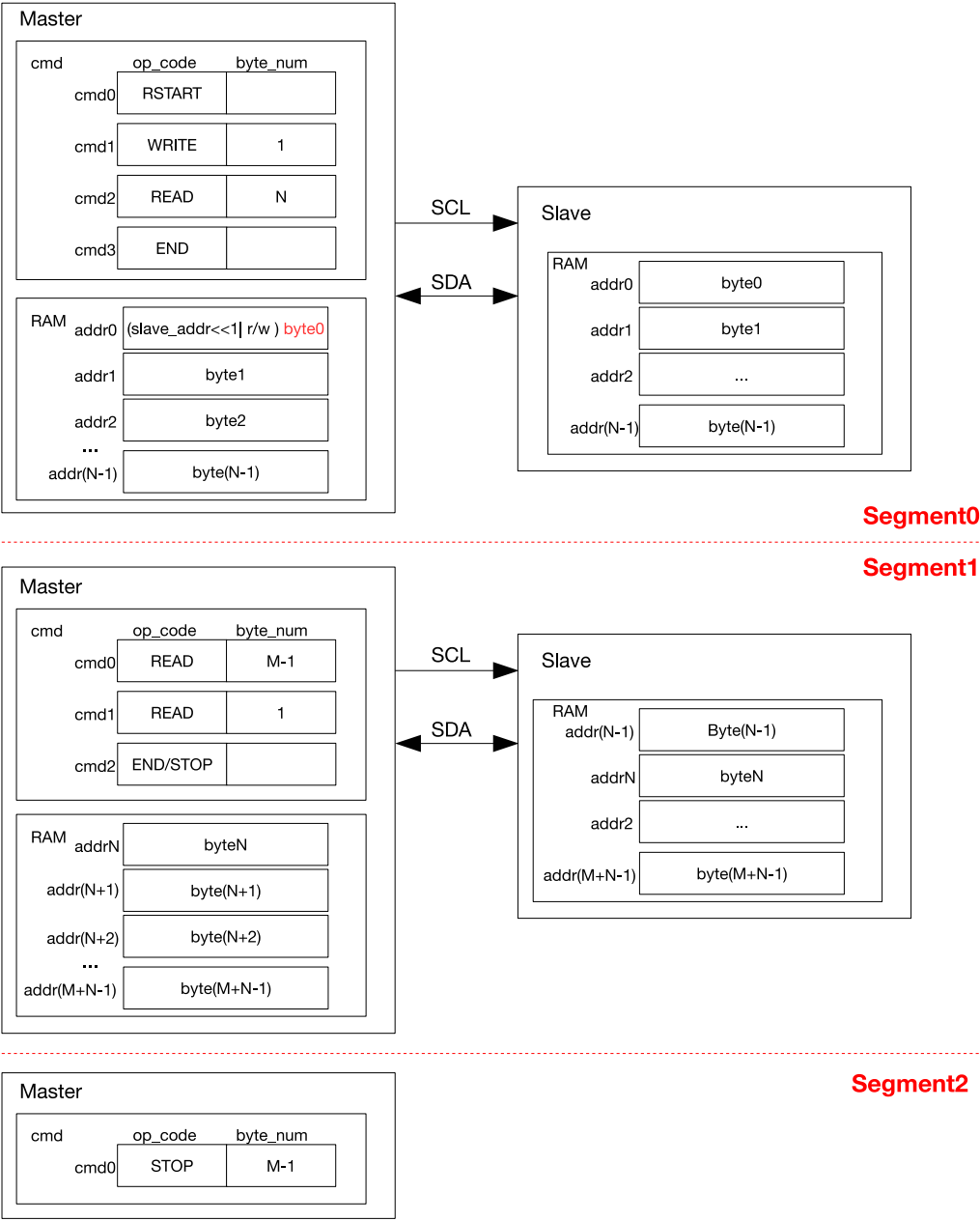
图 34.7-8. I2C 主机分段读 7 位寻址的从机
