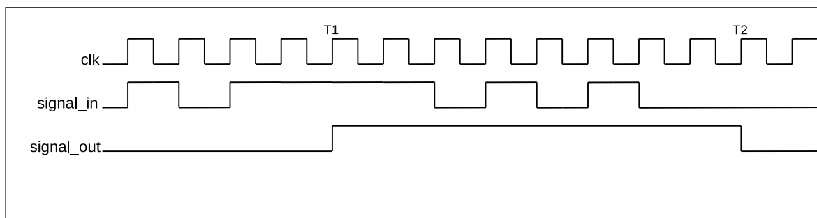
图 8.4-3. 毛刺滤波器时序示例
