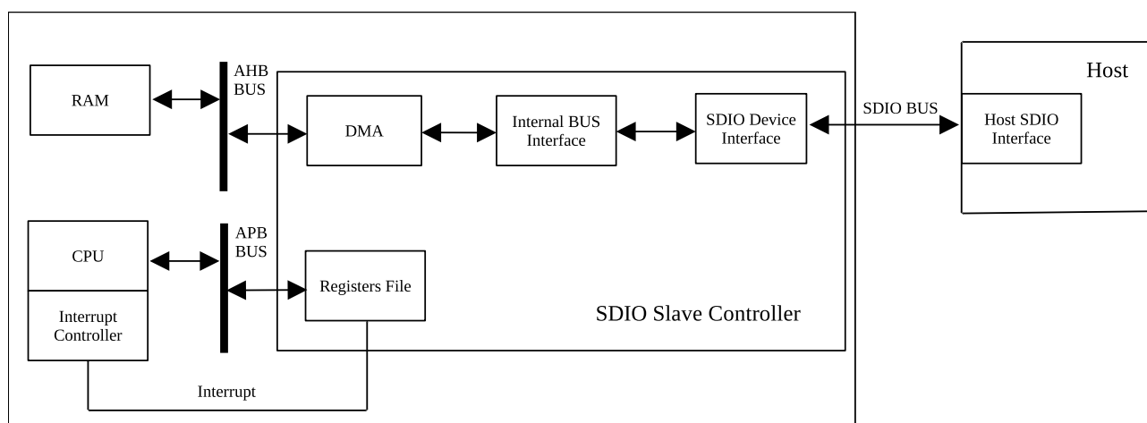
图 39.3-1. SDIO 从机功能结构图
