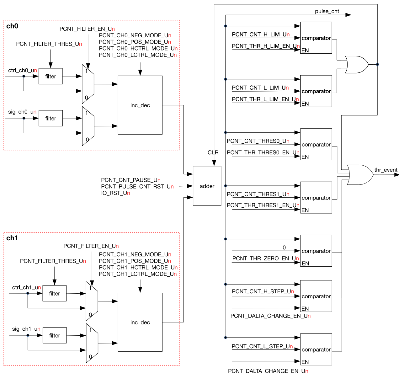
图 36.2-1. PCNT 单元基本架构图
