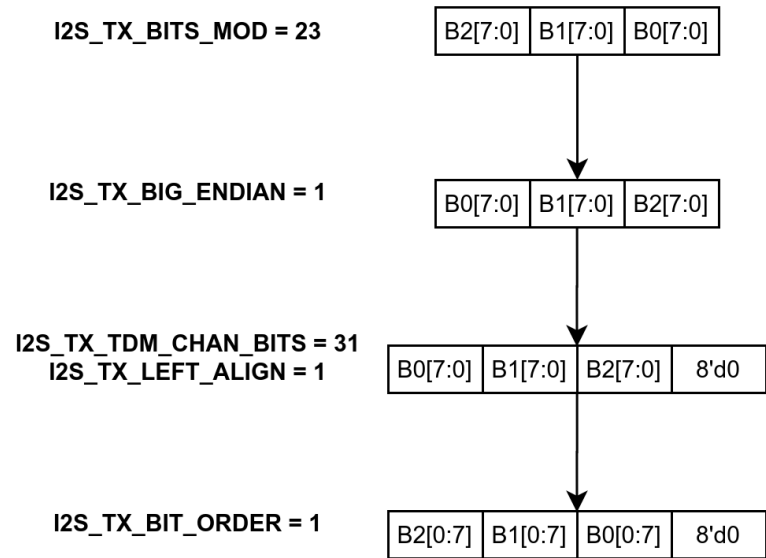
图 35.9-1. TX 数据格式控制
