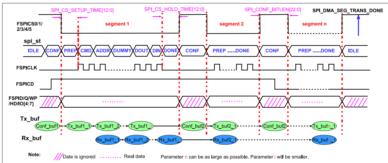
图 33.5-9. DMA 控制的分段配置传输
