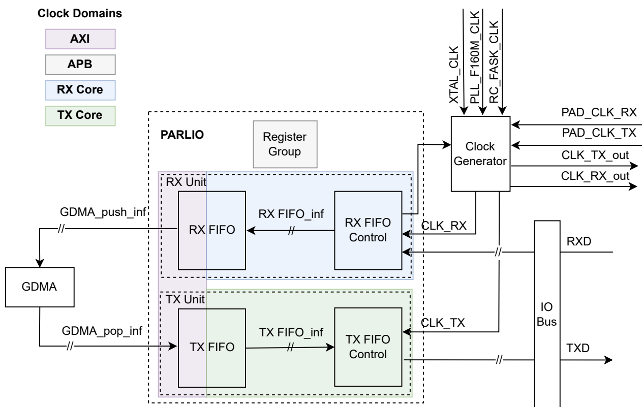
图 43.4-1. PARLIO 系统框图
