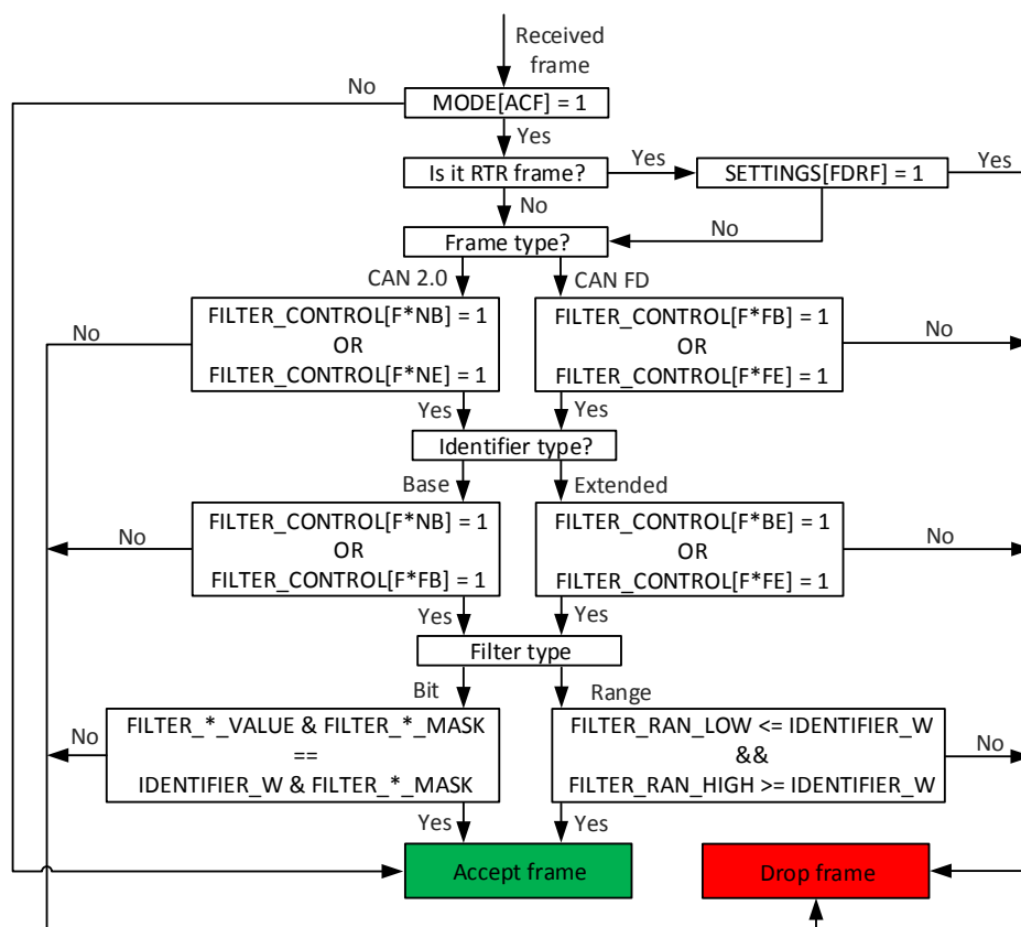
图 38.3-13. 帧过滤器工作流程 (* 以 A/B/C/R 类型过滤器为例)
