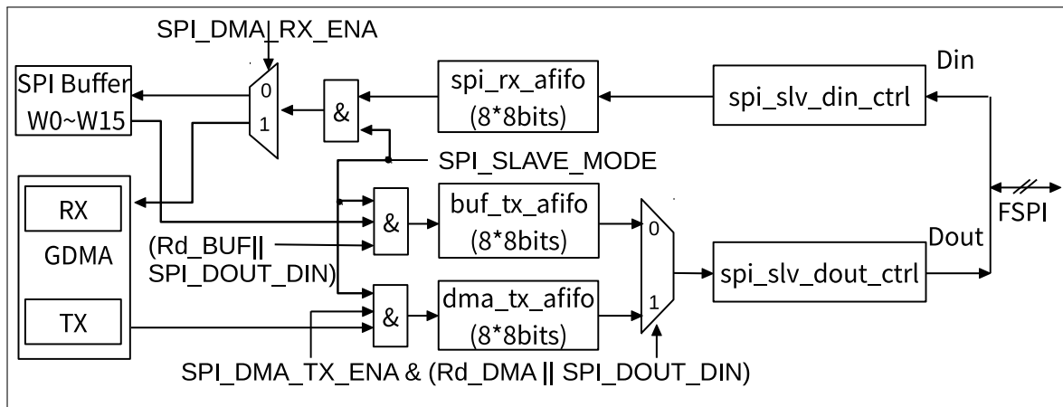
图 33.5-4. GP-SPI2 用作从机时的数据流控制
