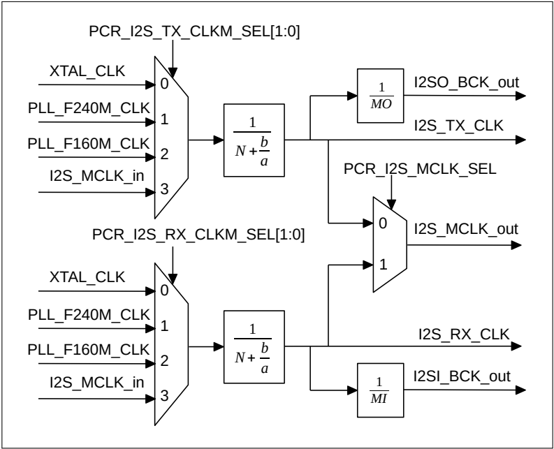
图 35.6-1. I2S 时钟分频器
