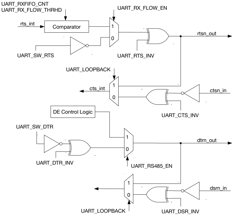
图 32.4-8. 硬件流控图
