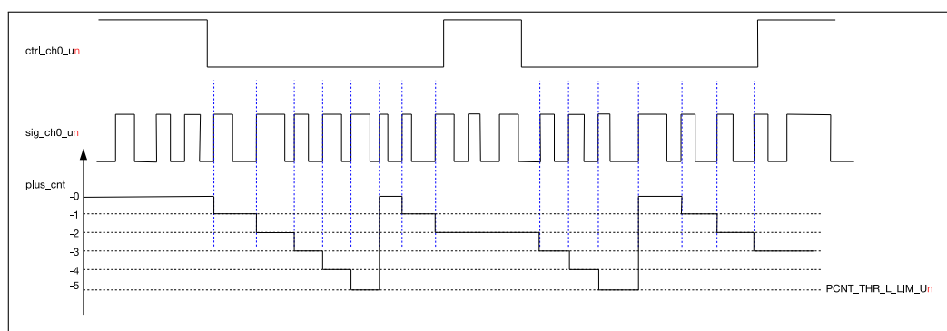
图 36.3-2. 通道 0 递减计数图
