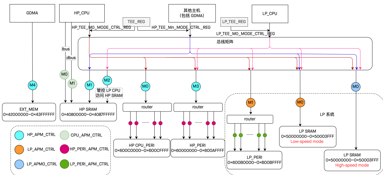
图 18.5-1. APM 控制器结构图
