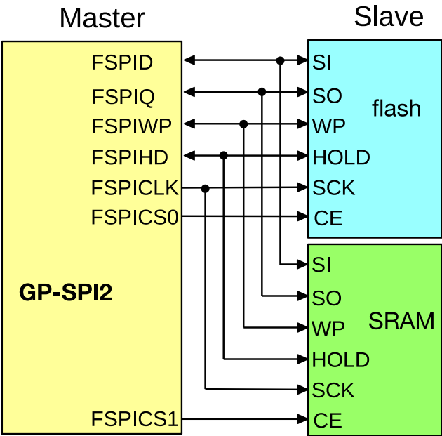
图 33.5-7. 4-bit 模式下 GP-SPI2 与 Flash 以及外部 RAM 的连接方式
