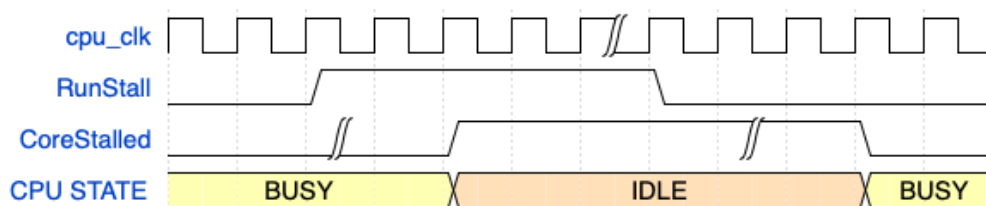
图 2.12-1. 使用 RunStall 时 CPU 核心状态的切换
