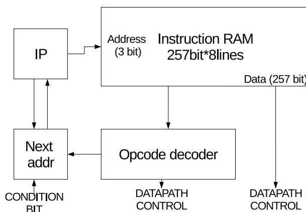
图 44.4-2. 比特调节器控制路径图
