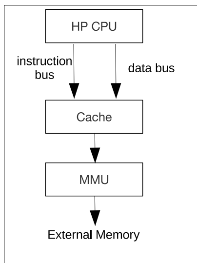
图 6.3-3. Cache 系统结构
