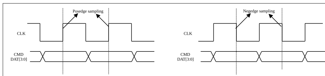
图 39.5-8. 采样时序图
