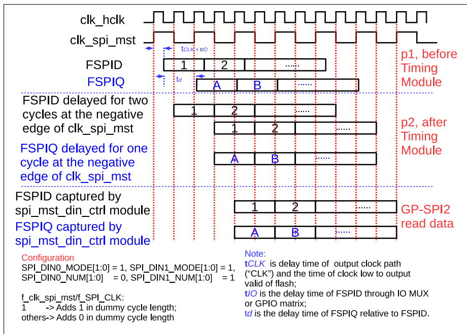
图 33.8-2. GP-SPI2 主机时序补偿示例
