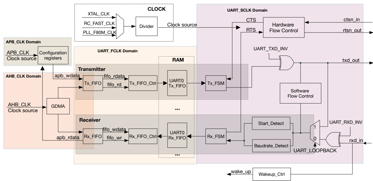
图 32.3-1. UART 基本架构图
