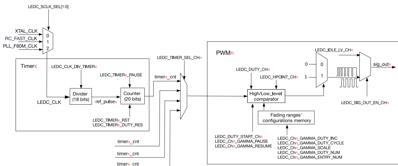
图 40.3-2. 定时器和 PWM 生成器功能框图
