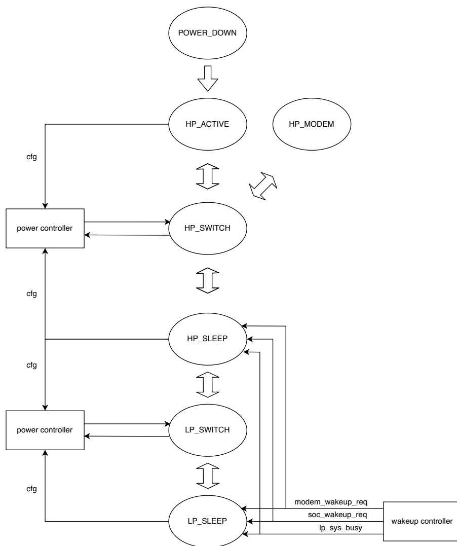
图 13.4-2. PMU 的主要工作流程
