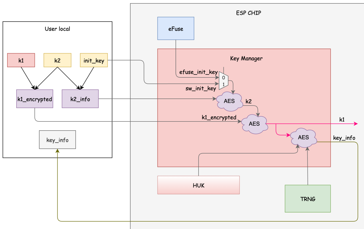
图 31.6-1. AES 部署模式
