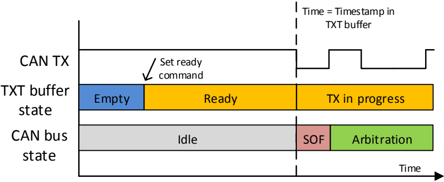
图 38.3-10. 定时发送
