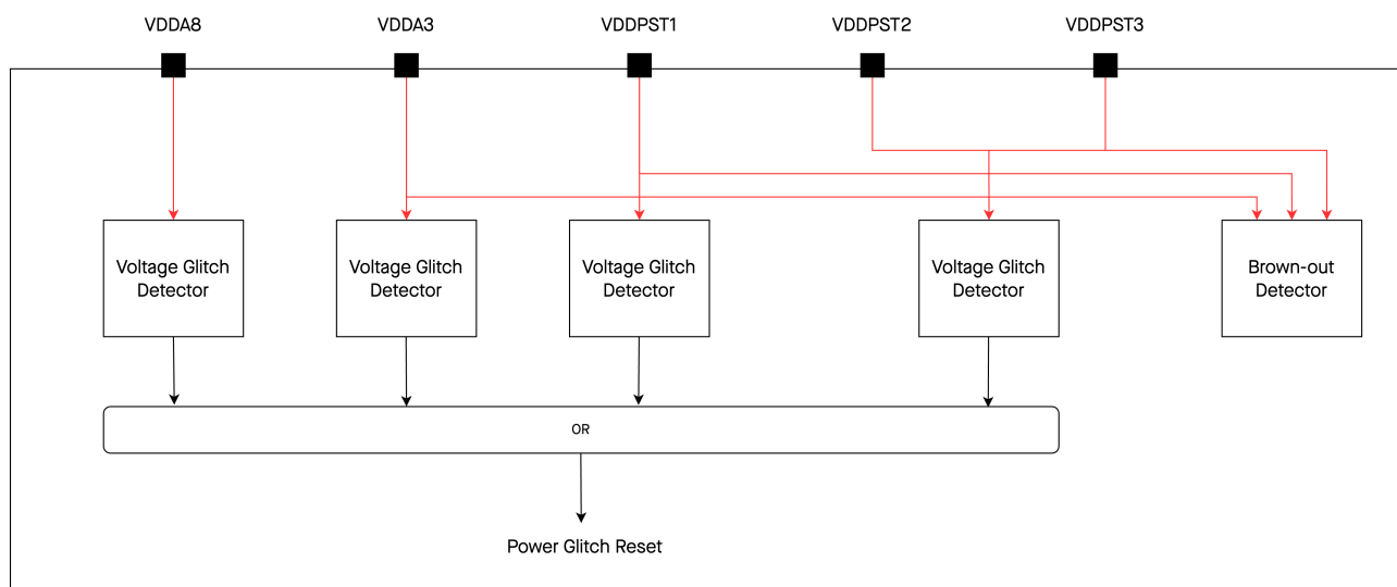
图 21.3-1. 电源检测器架构图
