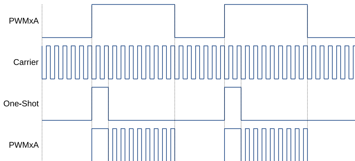
图 41.3-27. 载波模块的第一个脉冲和之后持续的脉冲示例
