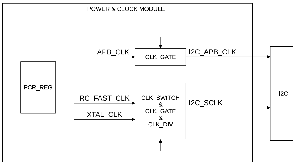
图 9.3-1. 时钟配置示例
