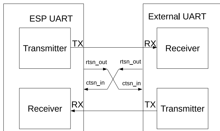
图 32.4-9. 硬件流控信号连接图
