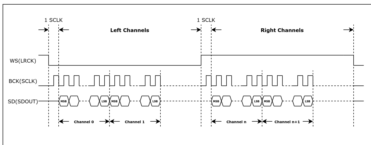
图 35.5-1. 时序图 – TDM Philips 标准
