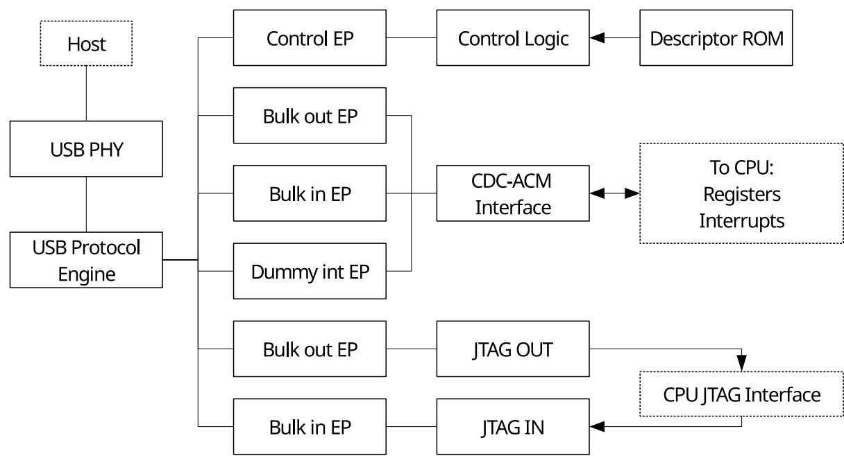
图 37.2-2. USB 串口/JTAG 控制器框图
