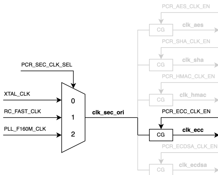
图 23.4-1. clk_ecc 时钟图
