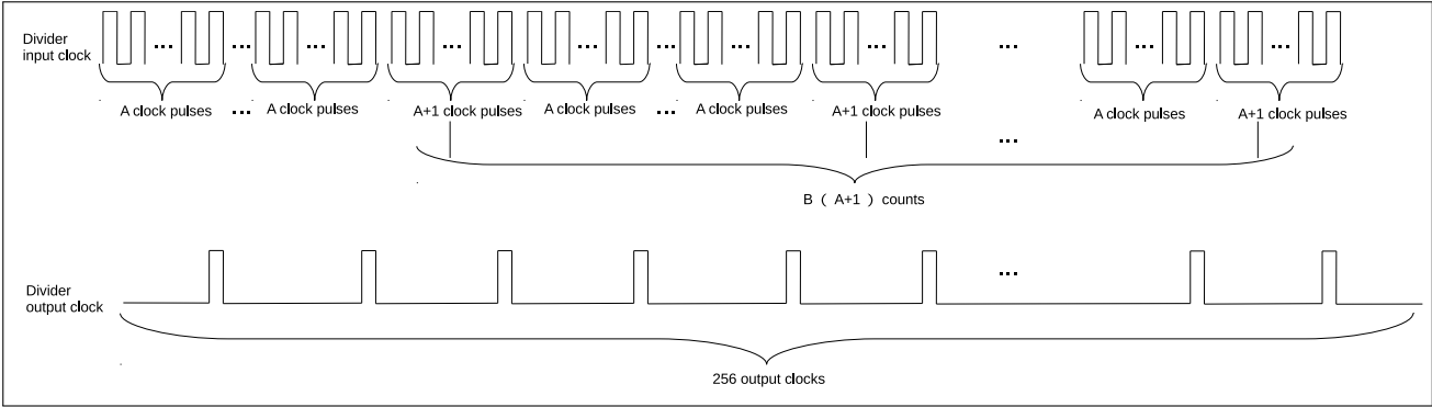
图 40.4-1. LEDC_CLK_DIV 为非整数时的分频
