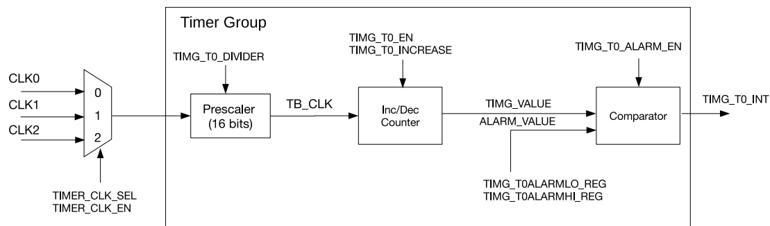
图 15.3-1. 定时器组架构
