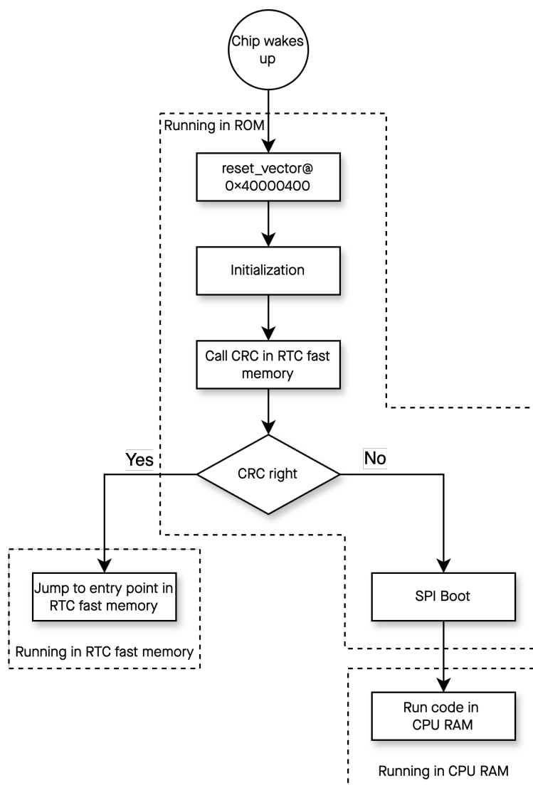
图 13.6-1. ESP32-C5 唤醒后的启动流程
