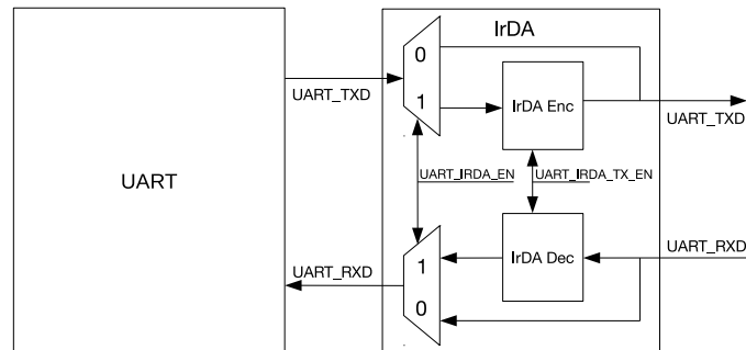
图 32.4-7. IrDA 编解码结构图
