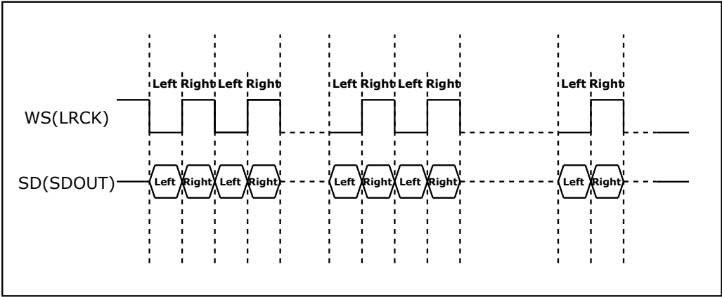
图 35.5-4. 时序图 – PDM 标准
