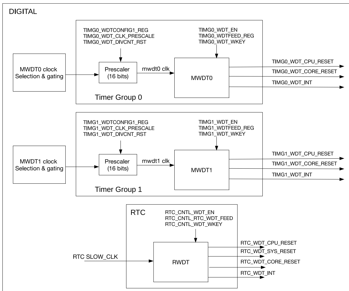
图 16.2-1. ESP32-C5 的数字看门狗定时器
