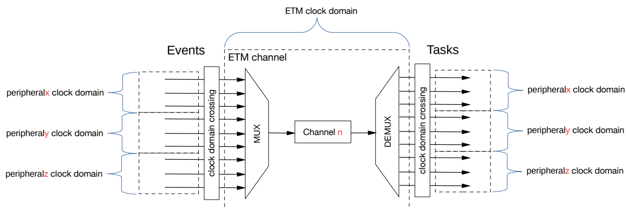
图 12.3-2. 事件任务矩阵时钟结构
