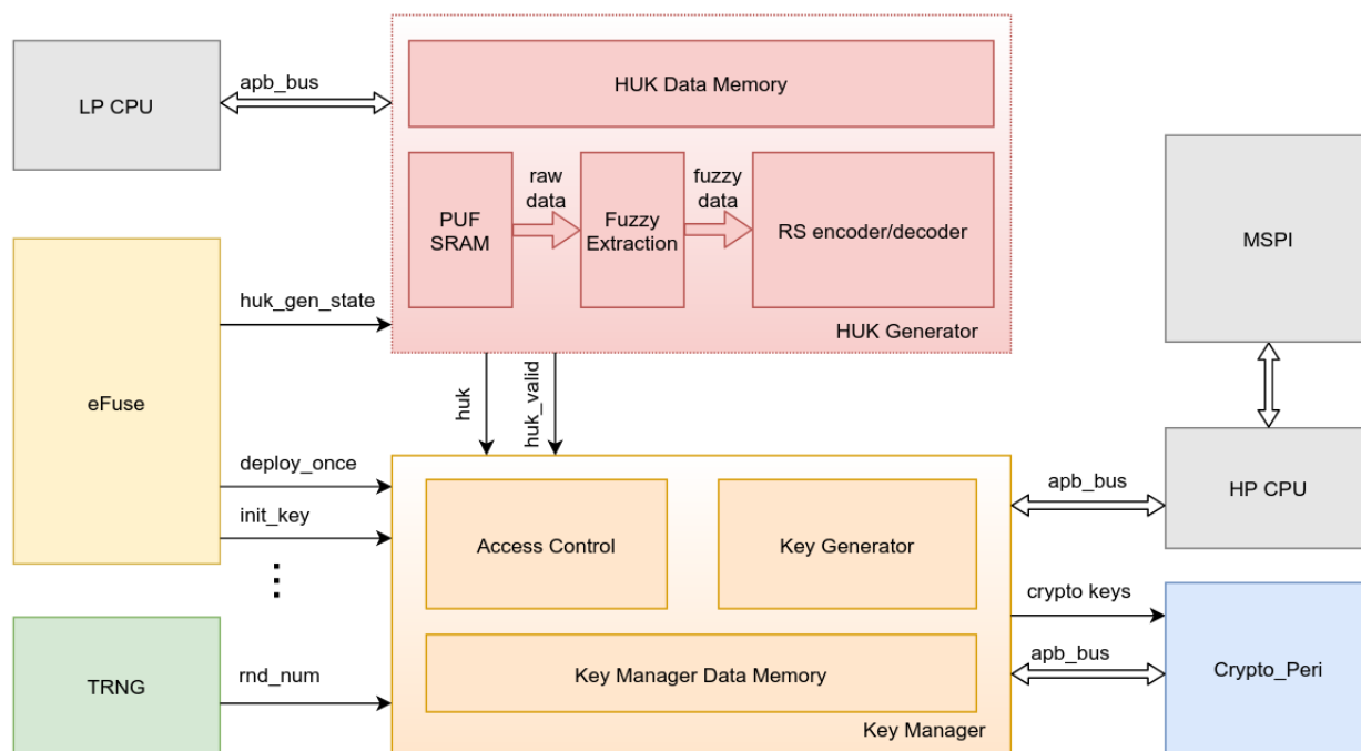
图 31.5-1. 密钥管理器 &amp; HUK 生成器架构
