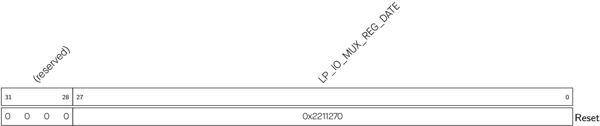
Register 8.59. LP_IO_MUX_DATE_REG (0x01FC)
