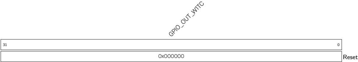
Register 8.4. GPIO_OUT_W1TC_REG (0x000C)
