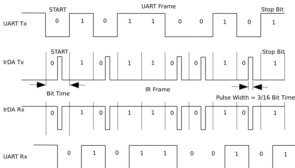
图 32.4-6. SIR 模式编解码时序图
