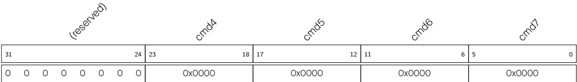
图 46.5-4. APB_SARADC_SAR_PATT_TAB2_REG 包含样式 4 - 7
