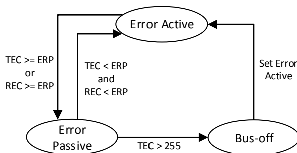
图 38.3-14. 故障限制
