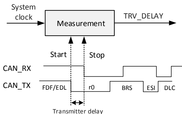
图 38.3-5. 发送器延迟测量
