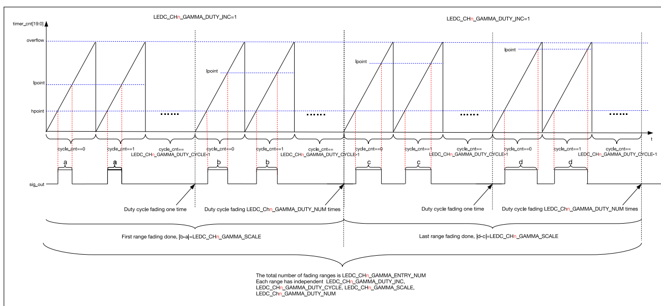
图 40.4-5. 输出信号占空比伽马曲线渐变图
