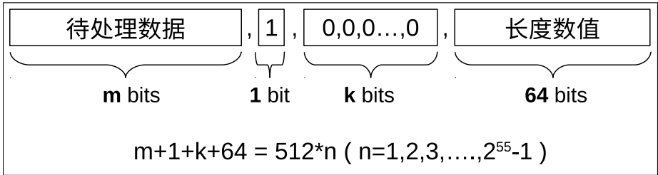
图 24.6-1. HMAC 附加填充位示意图
