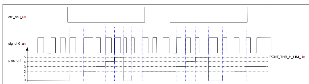
图 36.3-1. 通道 0 递增计数图
