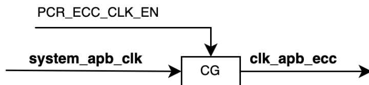
图 23.4-2. clk_apb_ecc 时钟图
