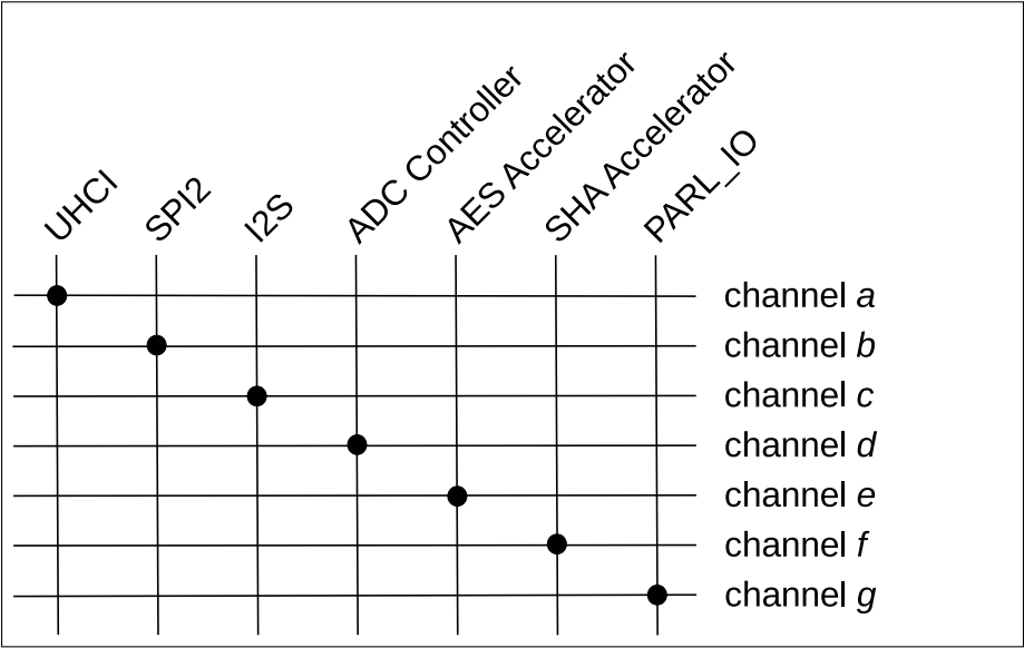
图 6.3-4. 具有 GDMA 功能的外设/模块
