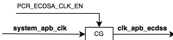
图 28.5-3. clk_apb_ecdsa 时钟图
