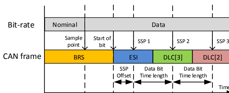
图 38.3-7. 二次采样点 2
