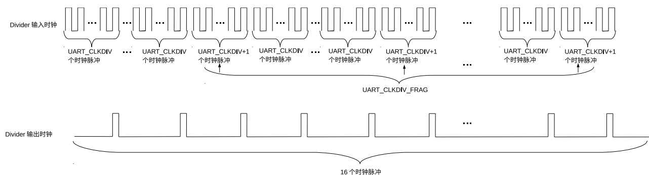
图 32.4-1. UART 控制器分频
