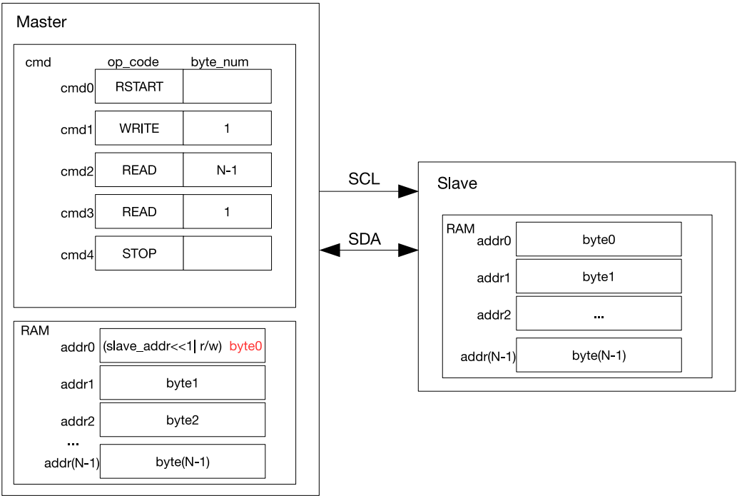
图 28.5-5. I2C 主机读 7 位寻址的从机
