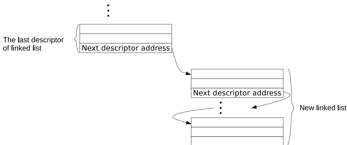
图 2.4-2. 链表关系图
