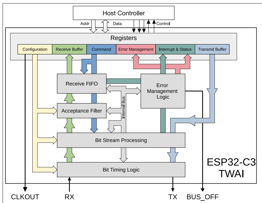
图 31.3-1. TWAI 概略图
