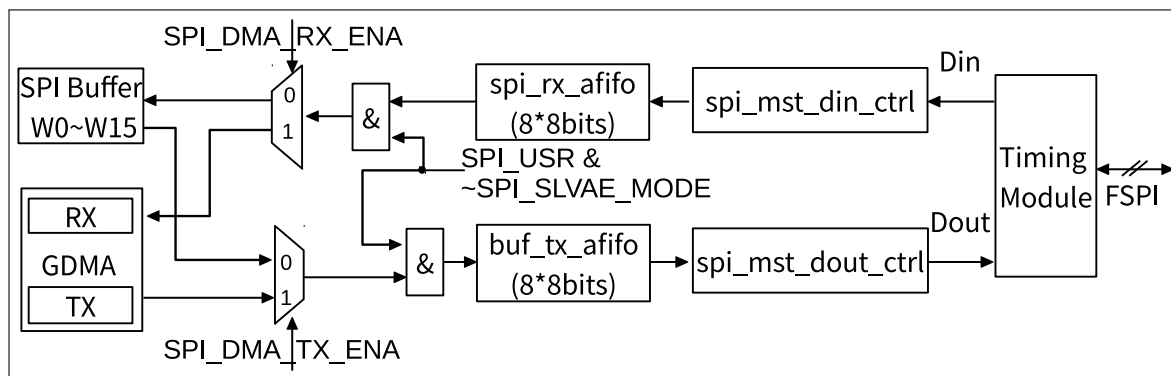
图 27.5-3. GP-SPI2 主机模式下的数据流控制
