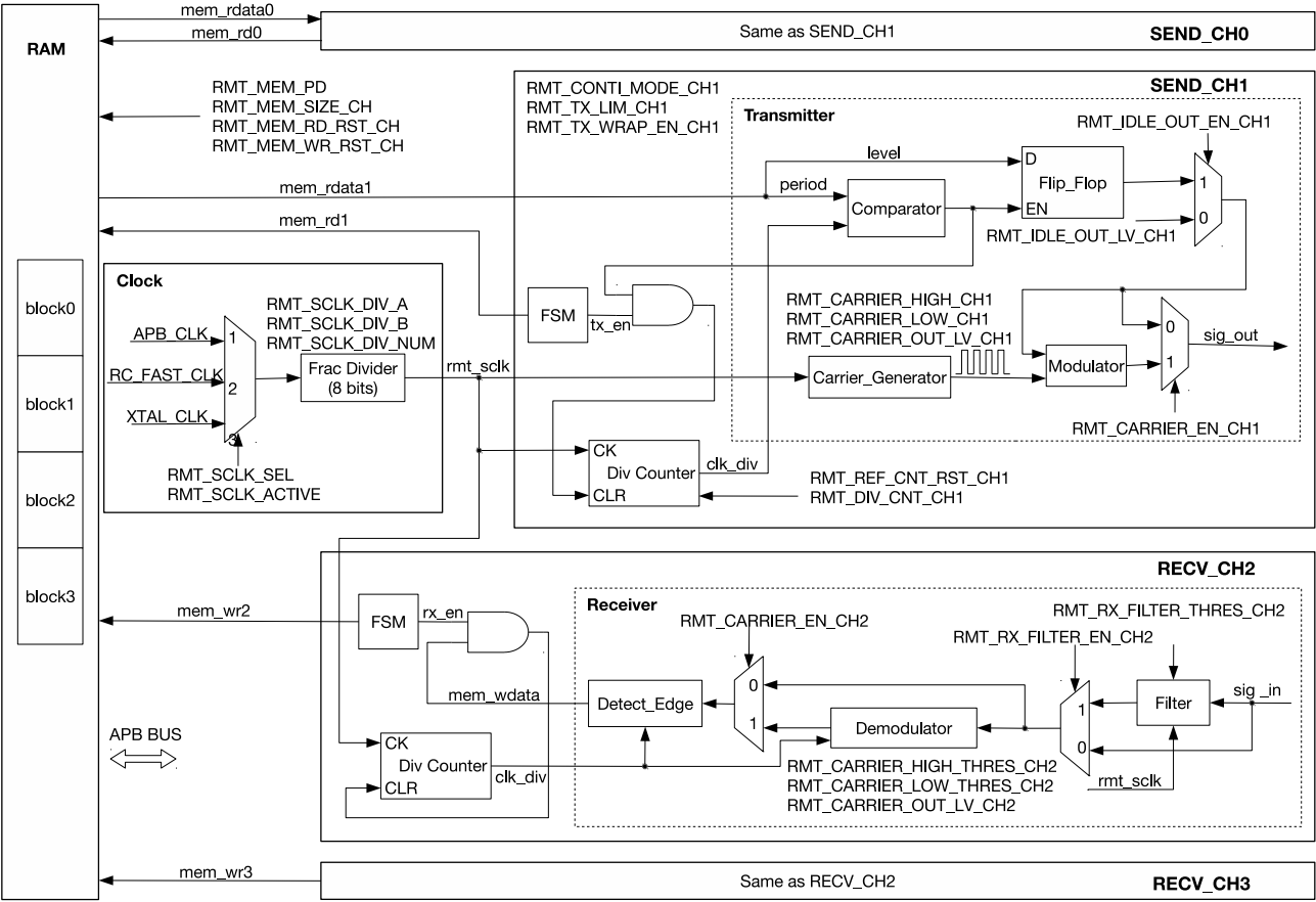
图 33.3-1. RMT 结构框图
