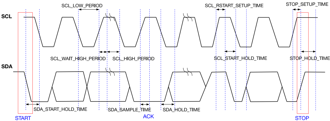
图 28.4-1. I2C 时序图
