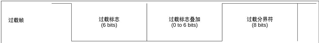
图 31.2-3. 过载帧中的位域
