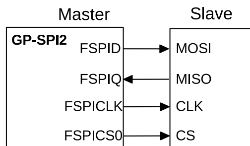
图 27.5-6. GP-SPI2 主机使用全双工模式与 SPI 从机通信框图
