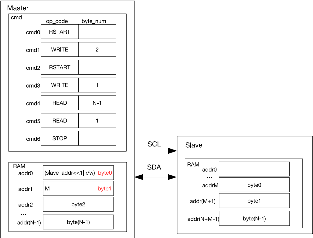
图 28.5-7. I2C 主机从 7 位寻址从机的 M 地址读取 N 个数据
