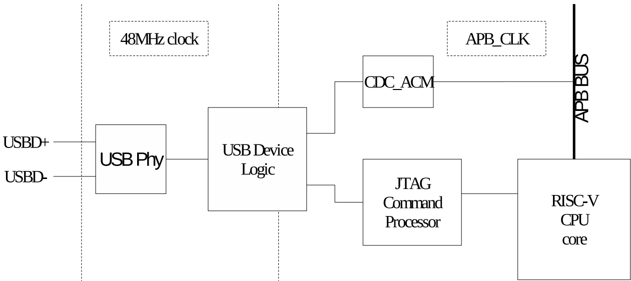
图 30.2-1. USB Serial/JTAG 高层框图
