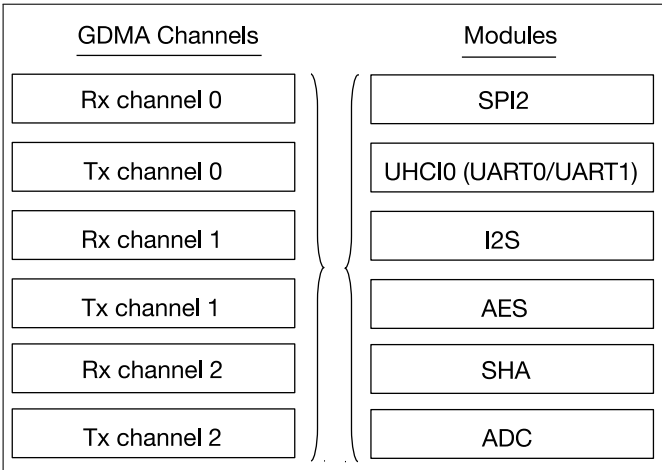
图 2.1-1. 具有 GDMA 功能的模块和 GDMA 通道
