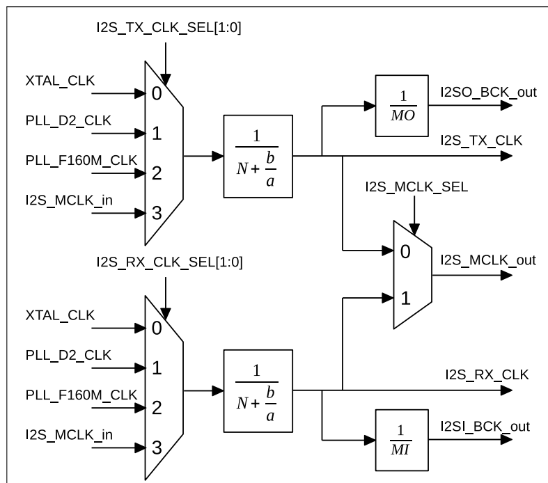
图 29.6-1. I2S 时钟
