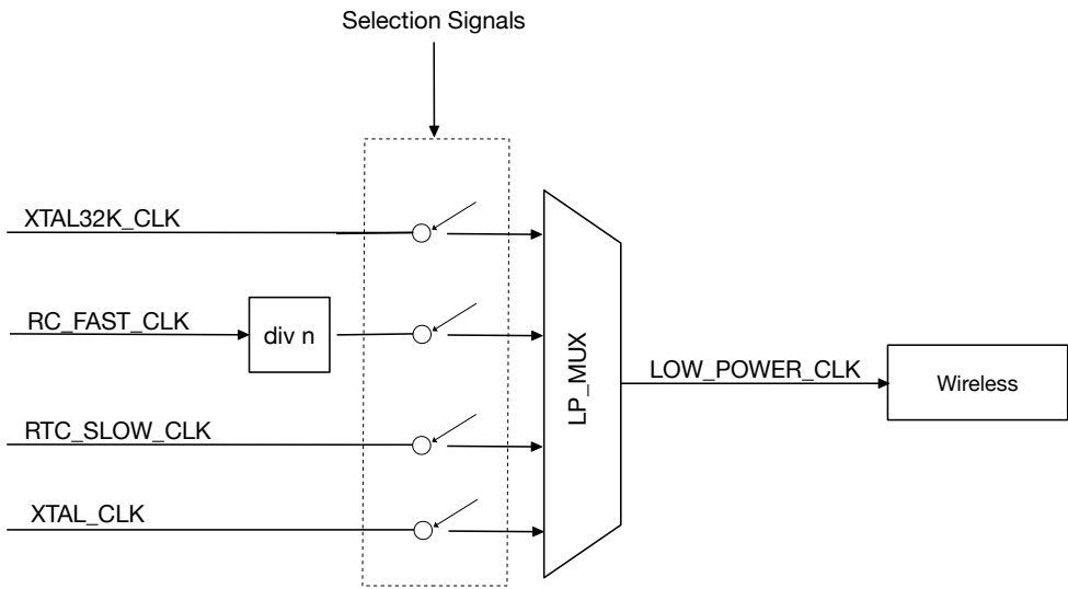
图 9.3-4. Wireless 时钟
