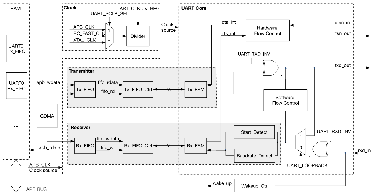
图 26.3-2. UART 基本架构图
