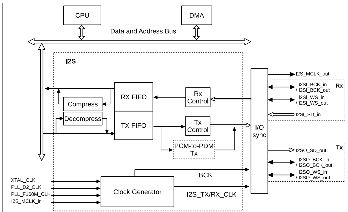
图 29.4-1. ESP32-C3 I2S 系统框图
