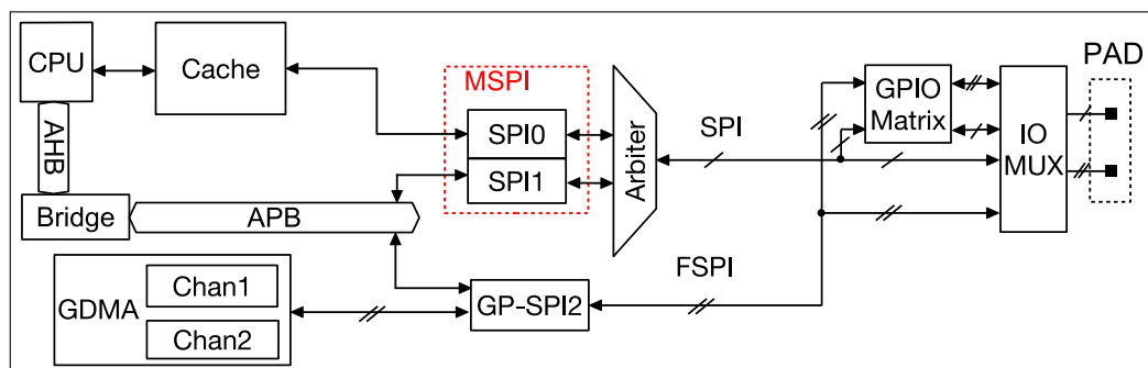
图 27.4-1. SPI 模块概览
