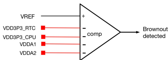
图 9.3-7. 欠压检测器
