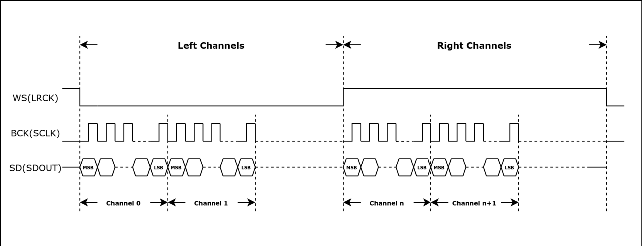
图 29.5-2. 时序图 – TDM MSB 对齐标准
