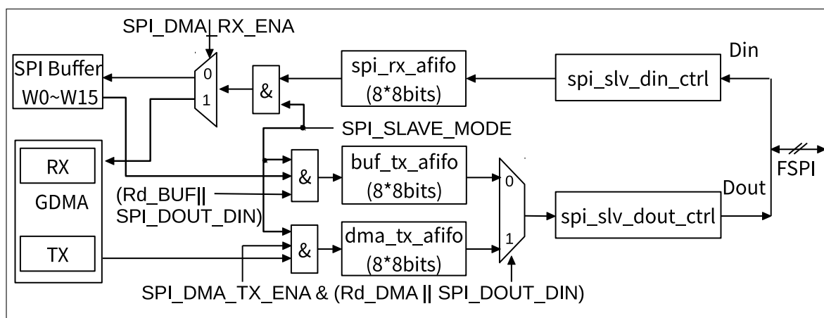
图 27.5-4. GP-SPI2 从机模式下的数据流控制
