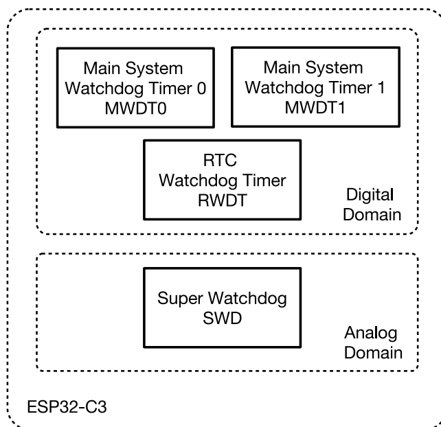
图 12.1-1. 看门狗定时器概览
