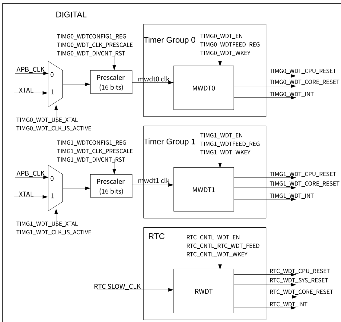
图 12.2-1. ESP32-C3 的看门狗定时器
