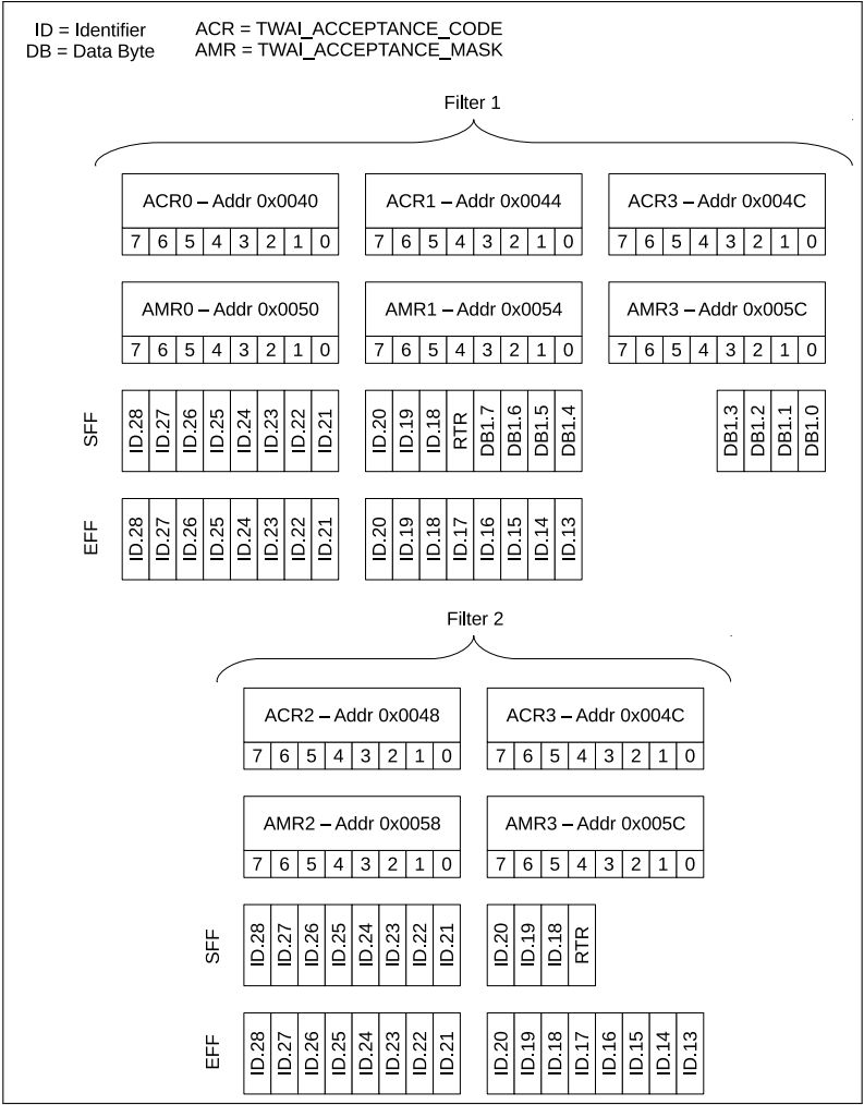
图 31.4-3. 双滤波模式
