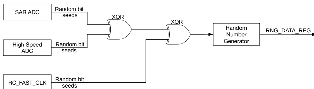
图 24.3-1. 噪声源
