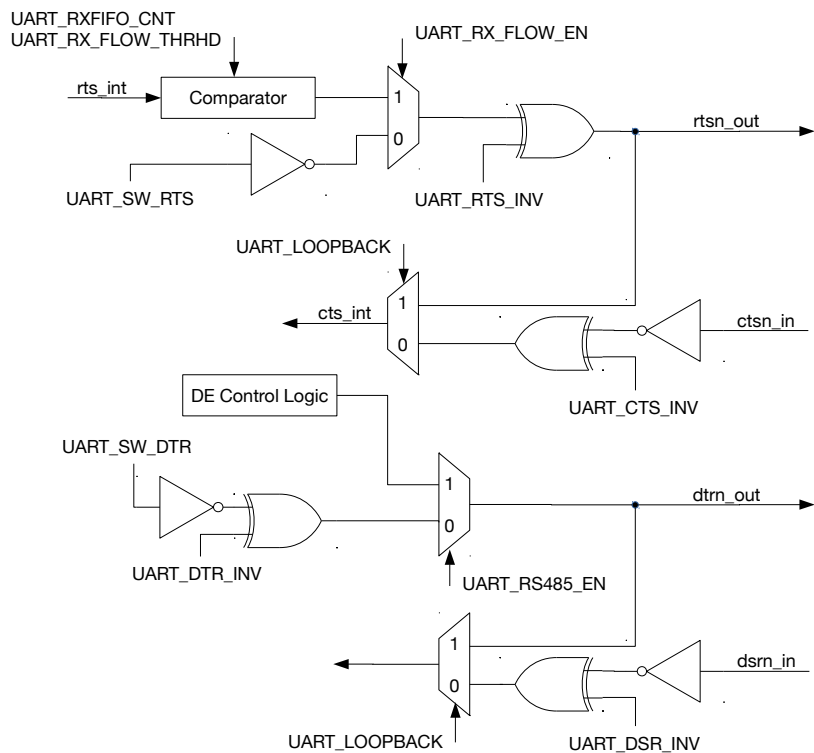
图 26.4-9. 硬件流控图
