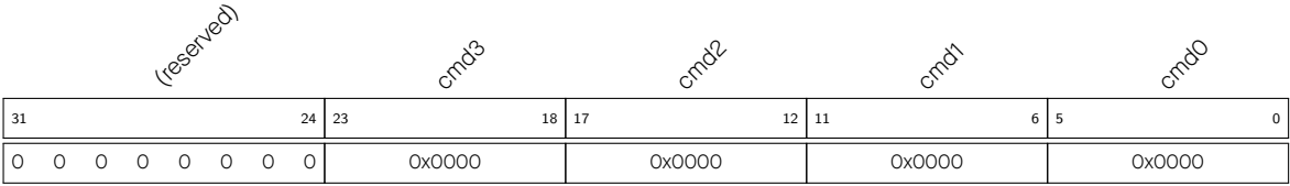
图 34.2-3. APB_SARADC_SAR_PATT_TAB1_REG 与样式 0 - 3
