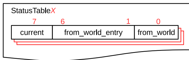
图 15.5-1. 世界切换记录表
