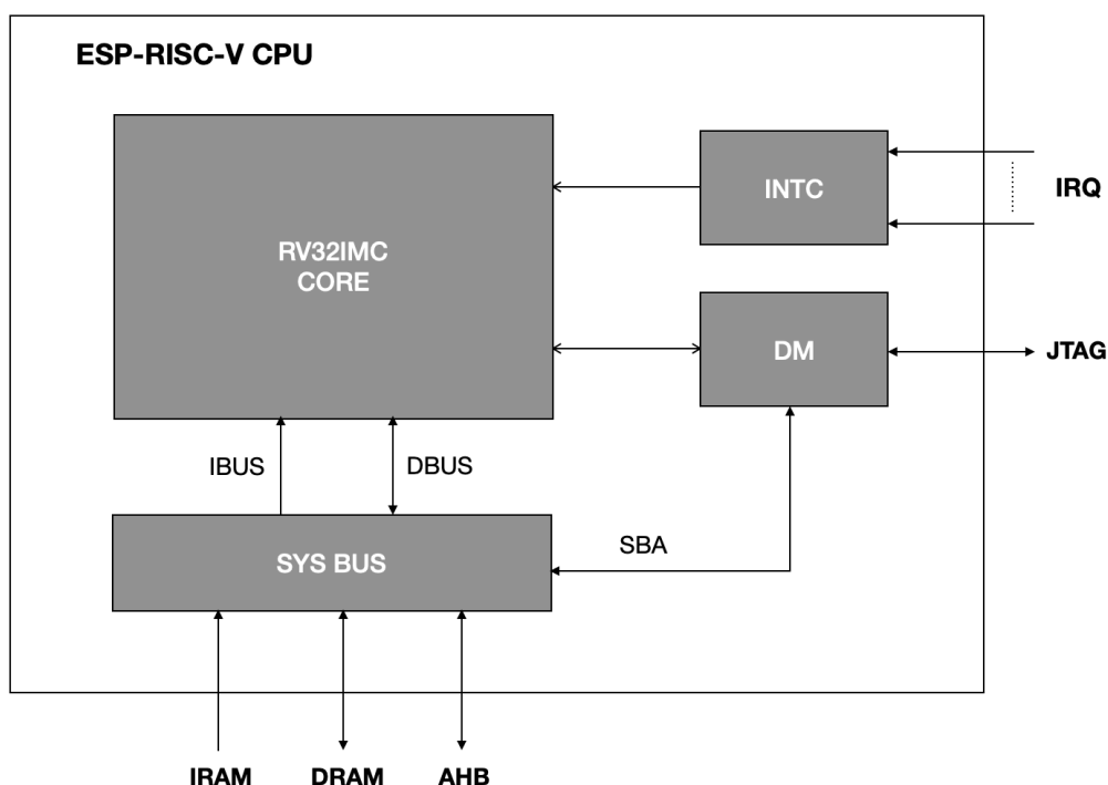
图 1.1-1. CPU 框图
