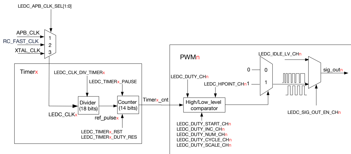
图 32.3-1. 定时器和 PWM 生成器功能块
