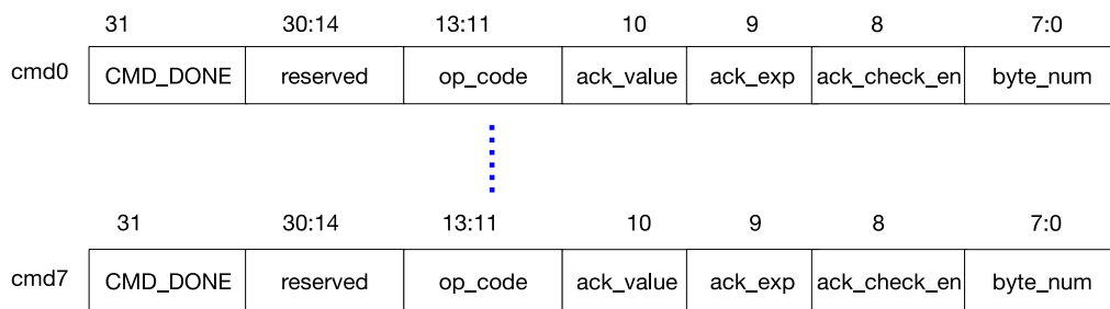
图 28.4-2. I2C 命令寄存器结构
