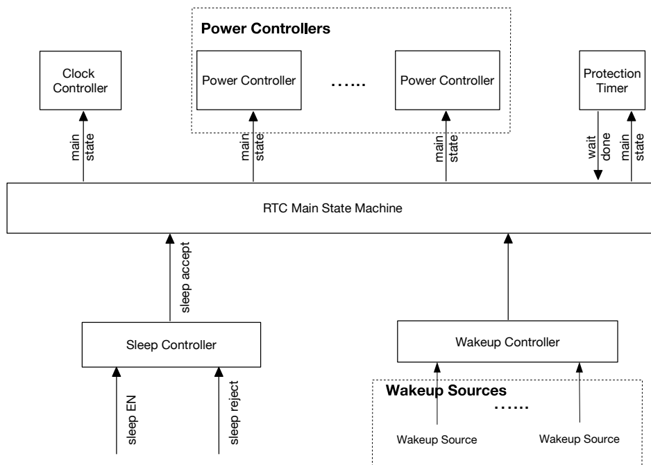
图 9.3-2. 电源管理单元的主要工作流程
