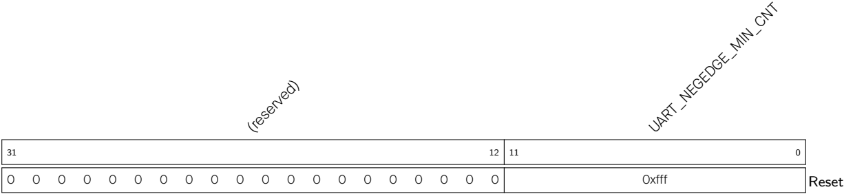
Register 26.27. UART_NEGPULSE_REG (0x0074)
