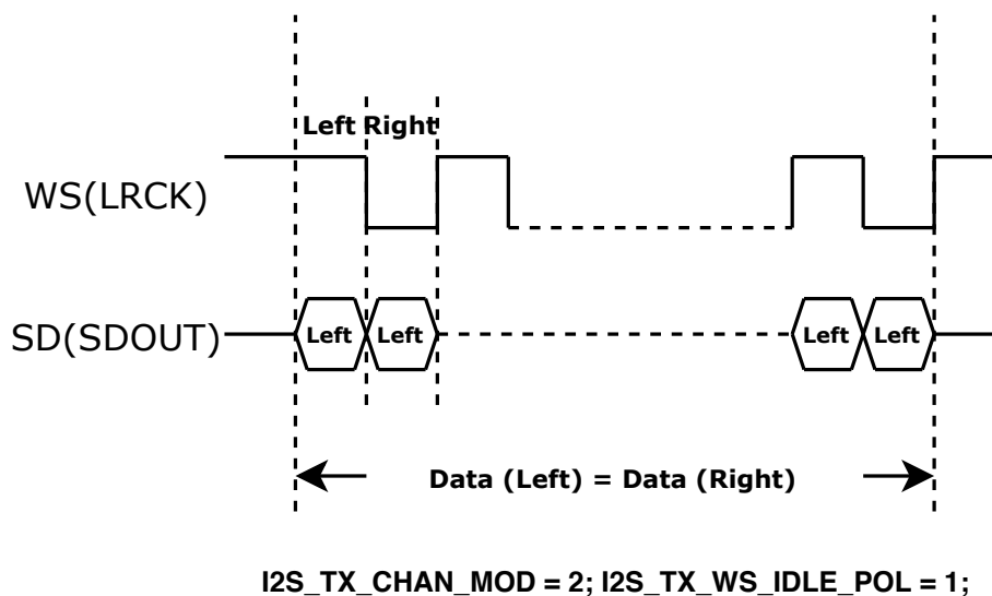
图 29.9-3. PDM 通道控制
