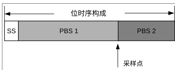
图 31.2-5. 标称位构成
