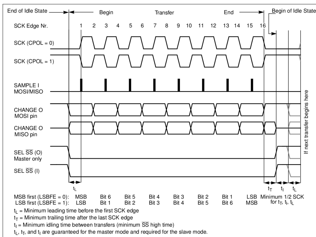
图 27.7-1. SPI 时钟模式 0 和时钟模式 2
