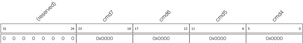
图 34.2-4. APB_SARADC_SAR_PATT_TAB2_REG 与样式 4 - 7
