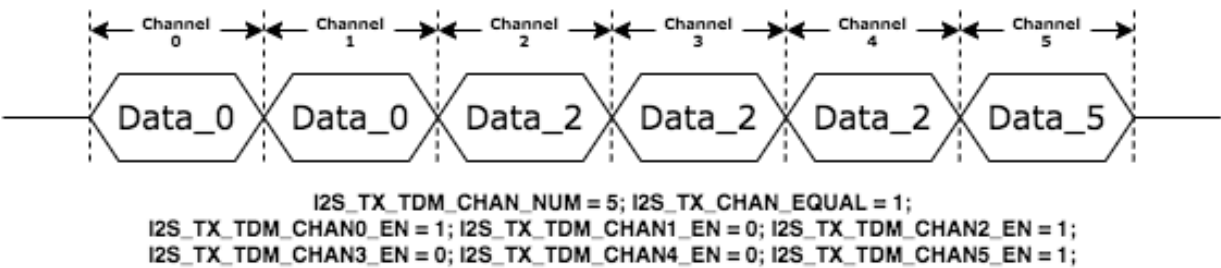
图 29.9-2. TDM 通道控制
