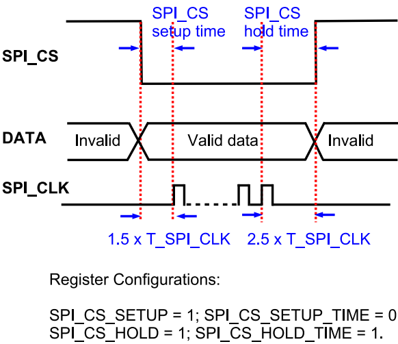
图 27.6-1. GP-SPI2 访问外部 RAM 时推荐的 CS 时序配置
