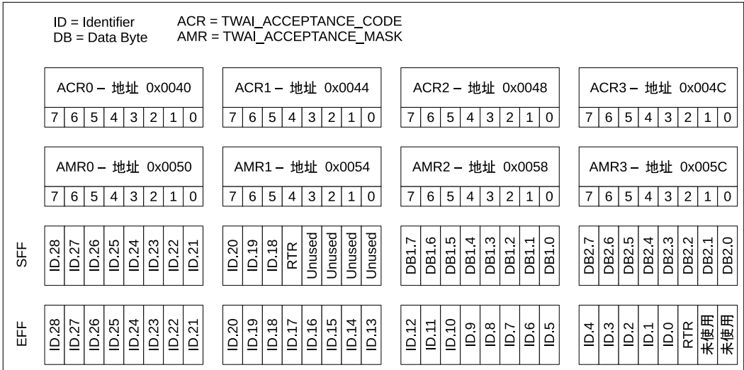
图 31.4-2. 单滤波模式
