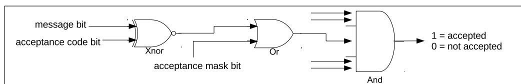
图 31.4-1. 接收滤波器
