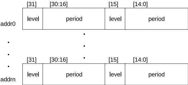
图 33.3-2. RAM 中脉冲编码结构
