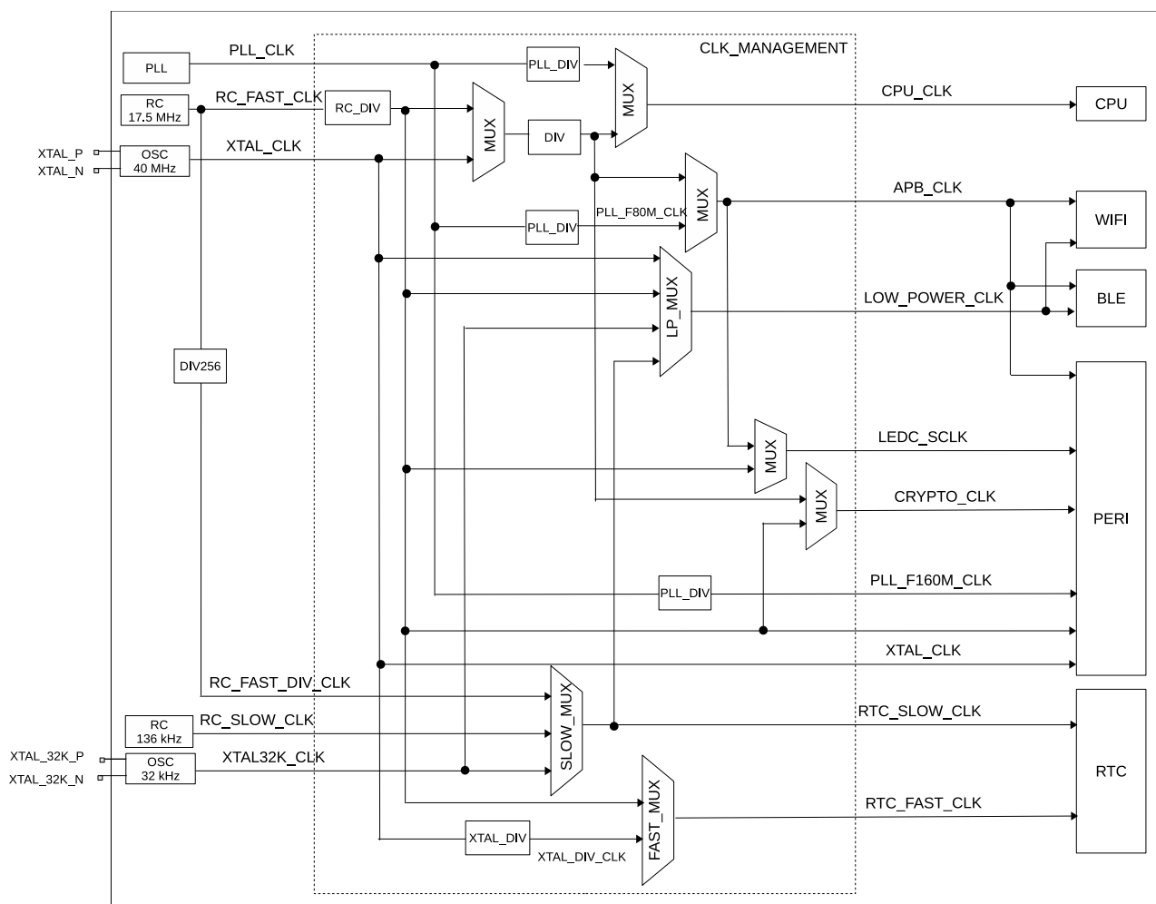
图 6.2-1. 系统时钟
