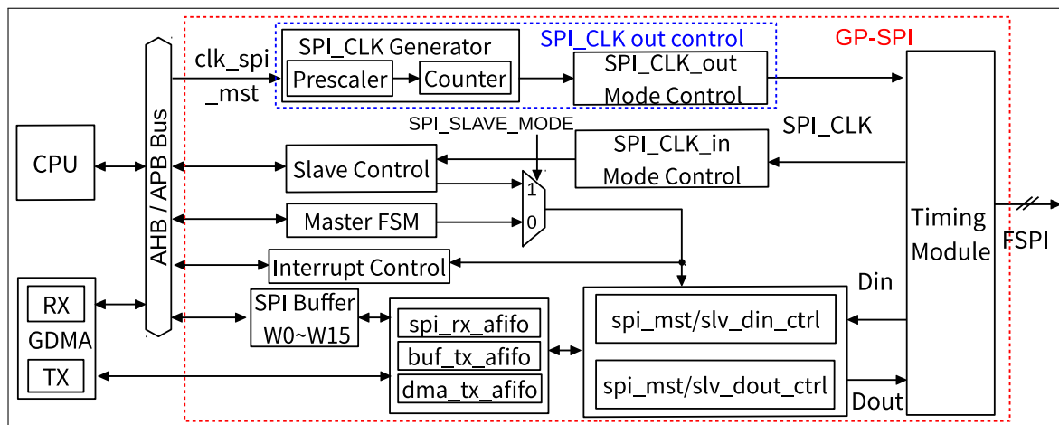
图 27.5-2. GP-SPI2 功能块图
