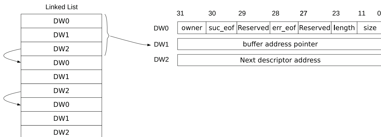
图 2.4-1. 链表结构图
