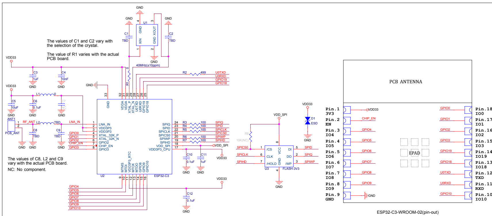
图 8-1. ESP32-C3-WROOM-02 原理图
