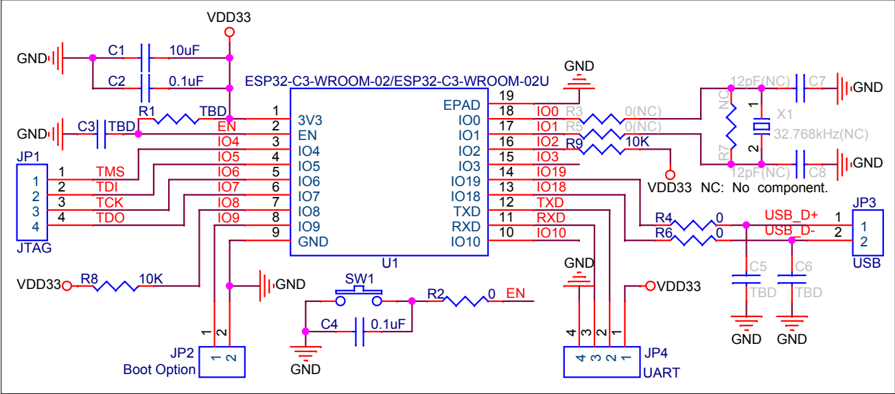
图 9-1. 外围设计原理图
