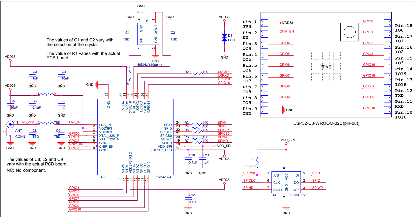
图 8-2. ESP32-C3-WROOM-02U 原理图
