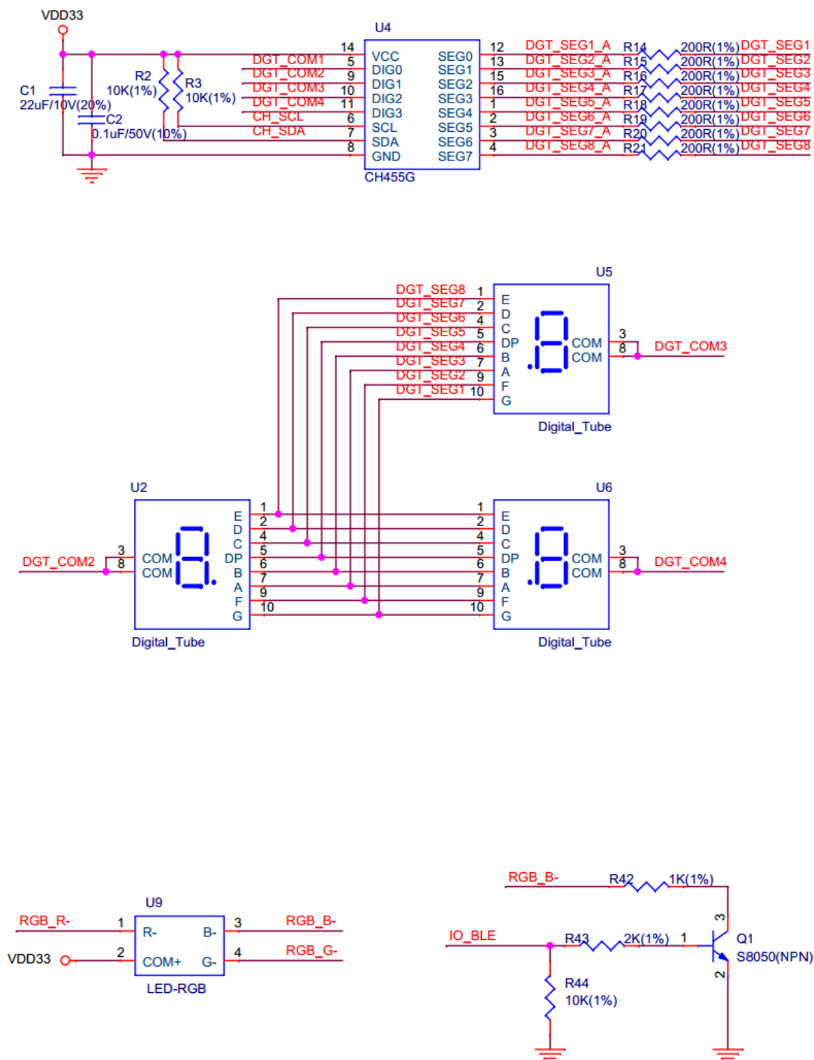
Fig. 10: Display Unit
